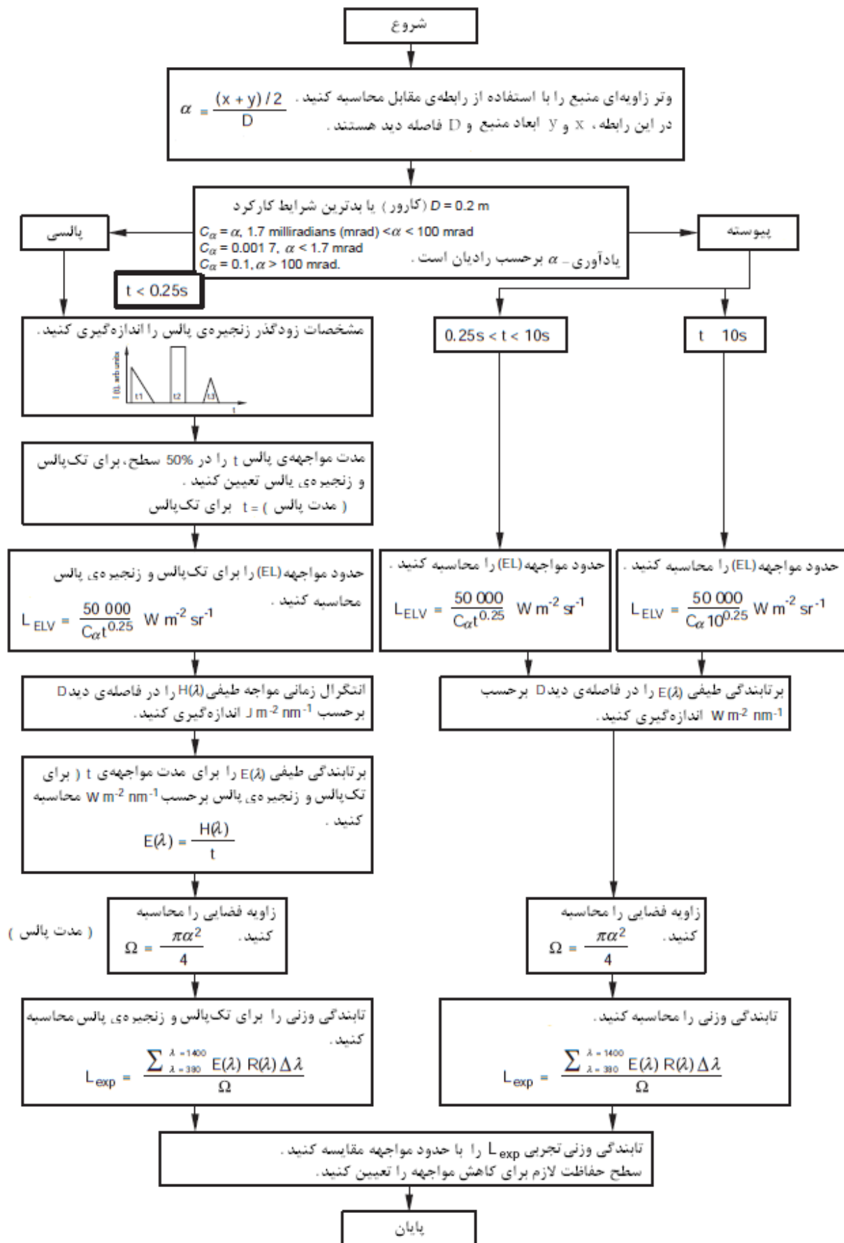
شکل ب-۱- فلوچارت ارزیابی خطر حرارتی بر روی شبکه
