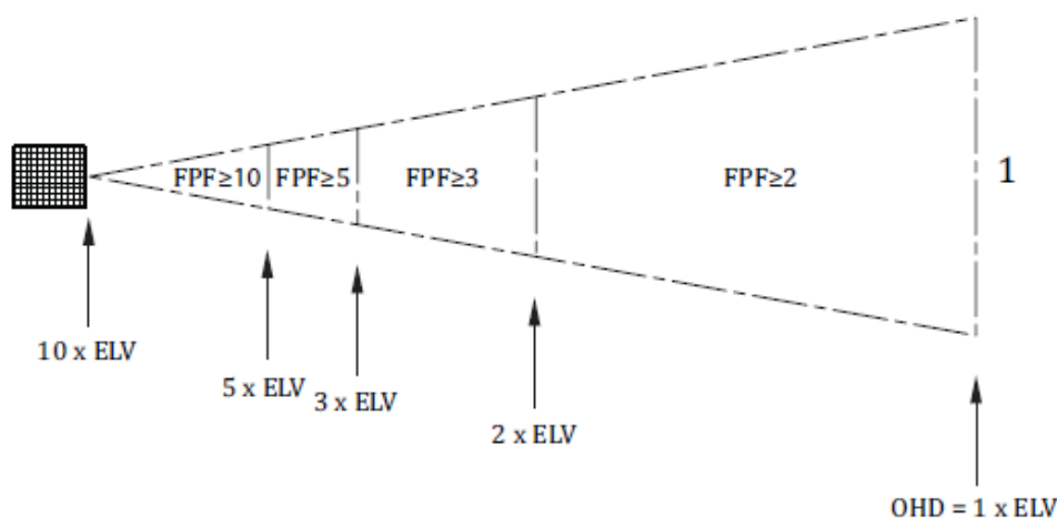
شکل ج-۱- سطح الزامی حفاظت چشم به‌وسیله یک وسیله ILS که با ضریب ۱۰ از ELV فراتر می‌رود
