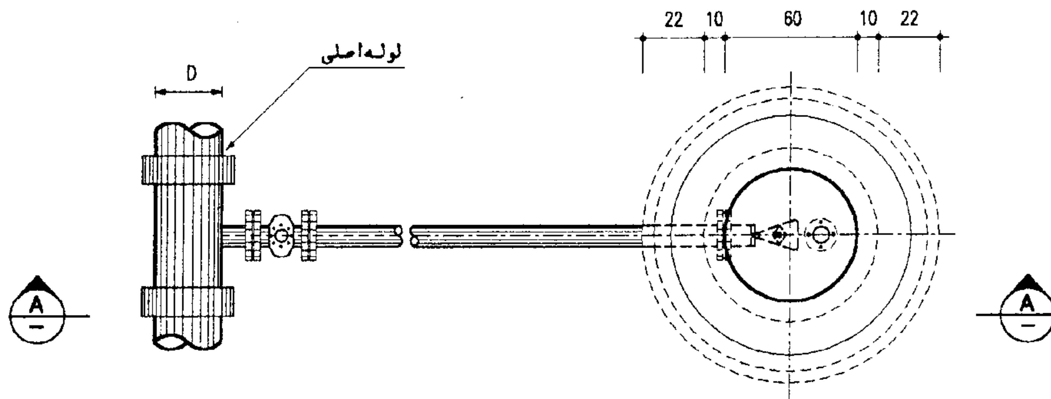
PLAN N.T.S
