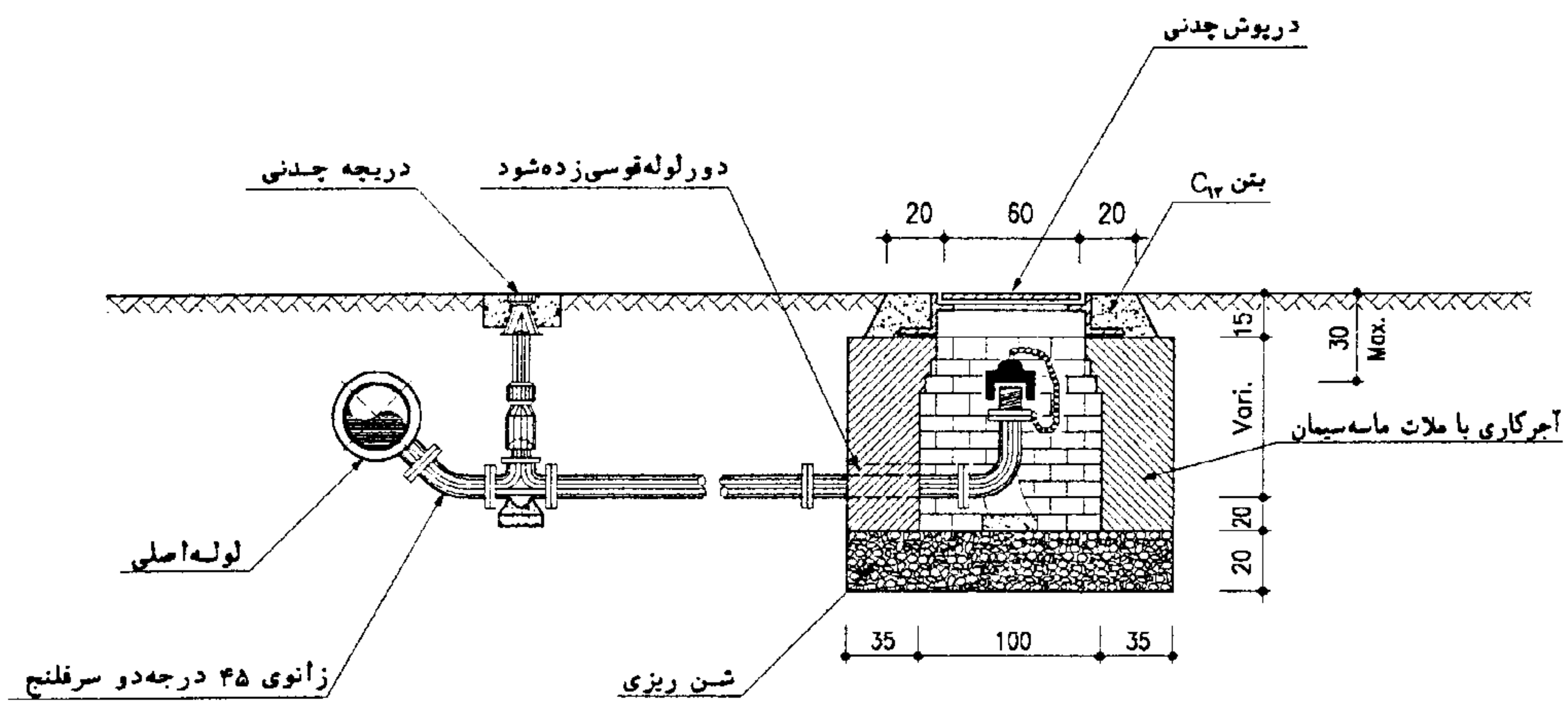
PLAN N.T.S
