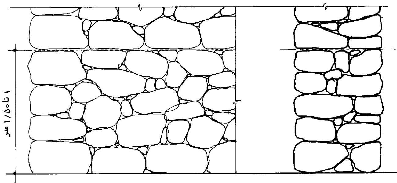
نمای دیوار
