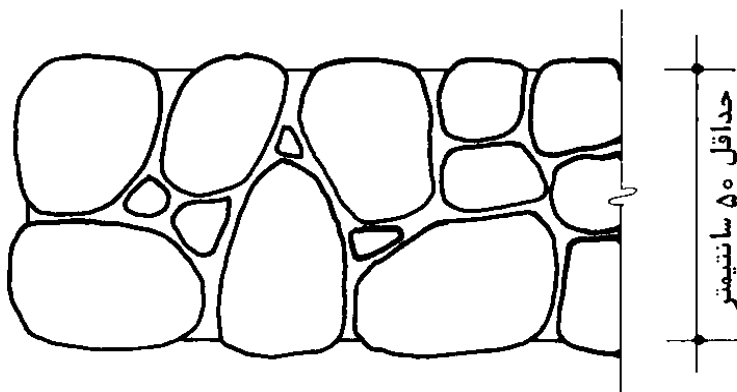
بافت افقی دیوار
