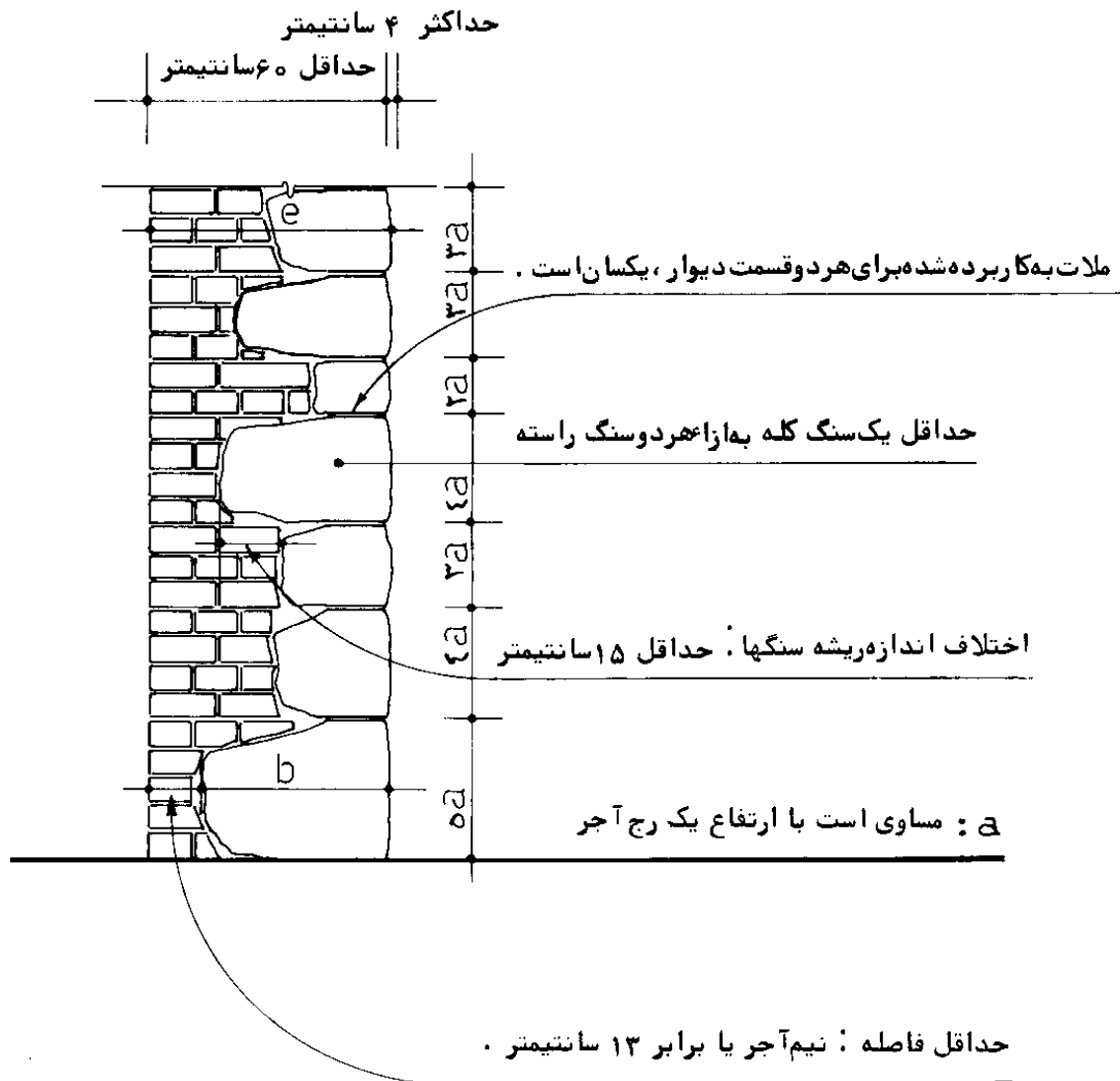
مقطع دیوار
