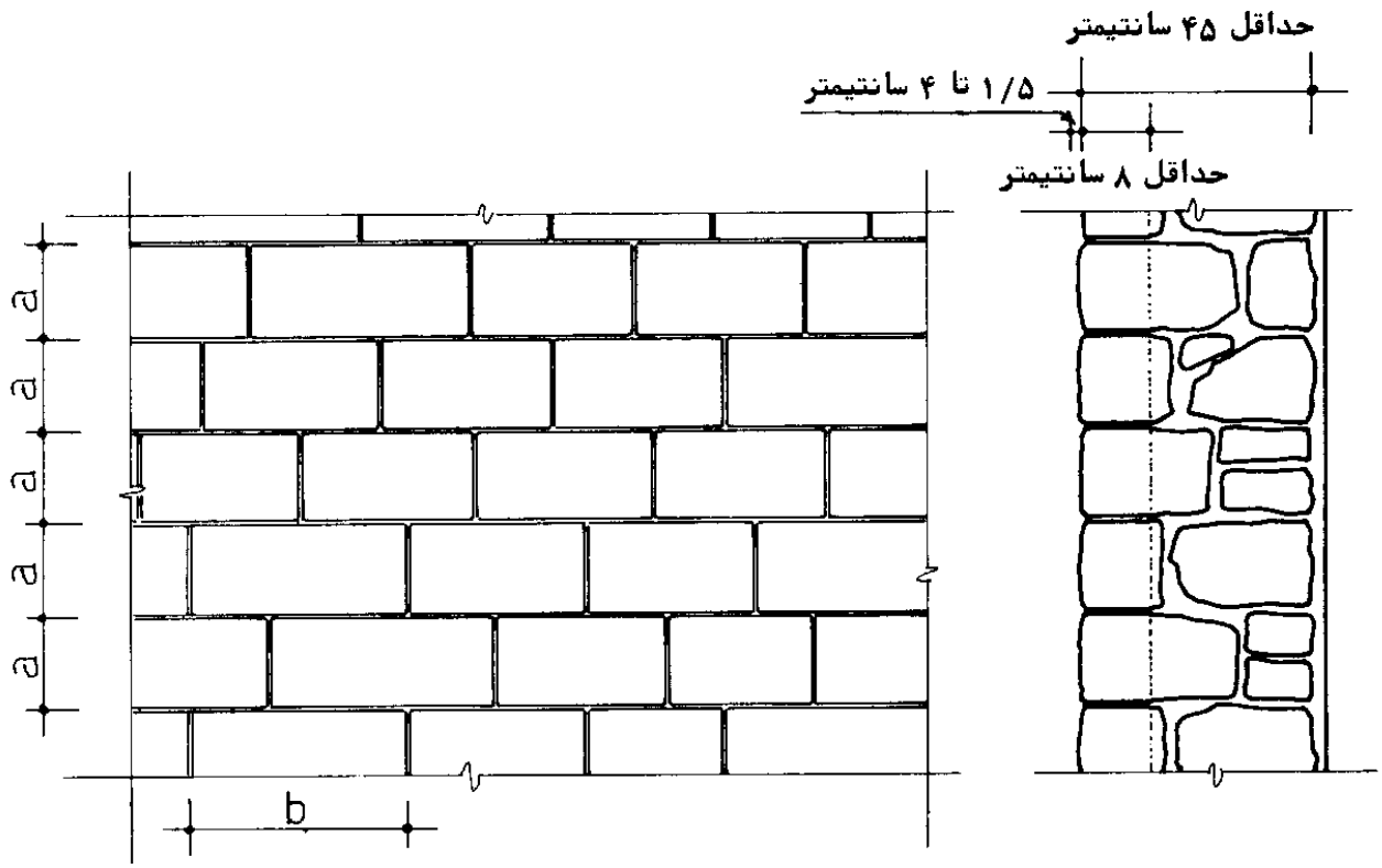
نمای دیوار
