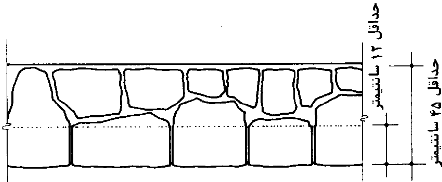
بافت افقی دیوار
