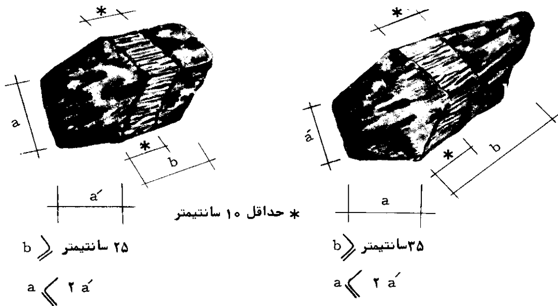
سنگ چندوجهی نامنظم سرتراش (کله وراسته)
