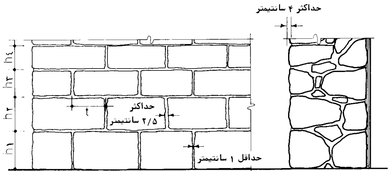
مقطع دیوار
