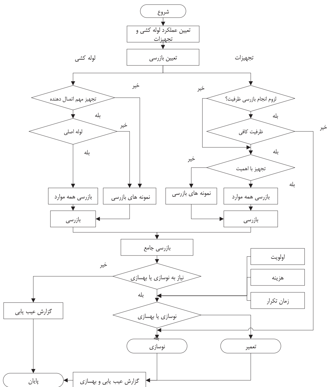
شکل ۹-۹ روند نمای ارزیابی لرزه‌ای تجهیزات داخلی
