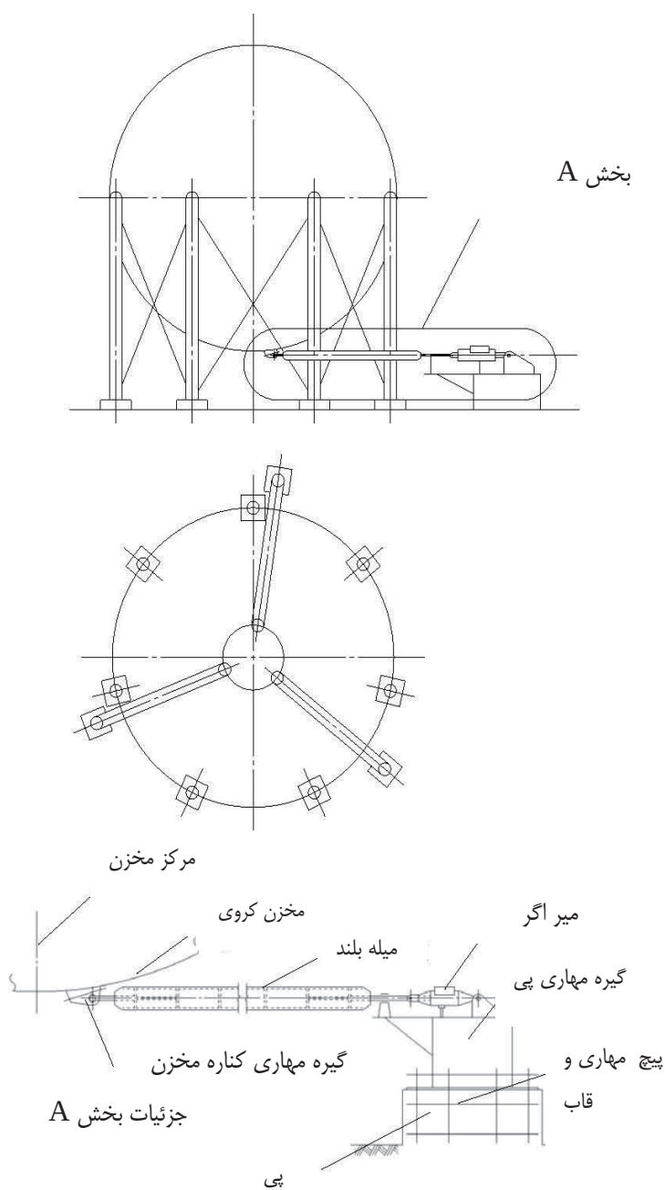
شکل ۳۵-۵ کنترل ارتعاش با استفاده از میراگر (از نوع میل بلند)
