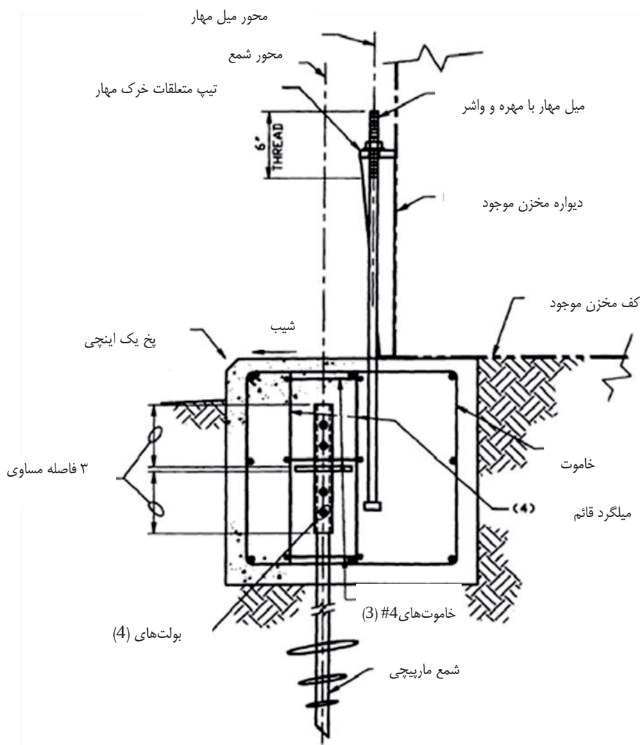
شکل ۶-۲۲ شم‌های ماریچج بکار رفته با پی دیواره حلقوی
