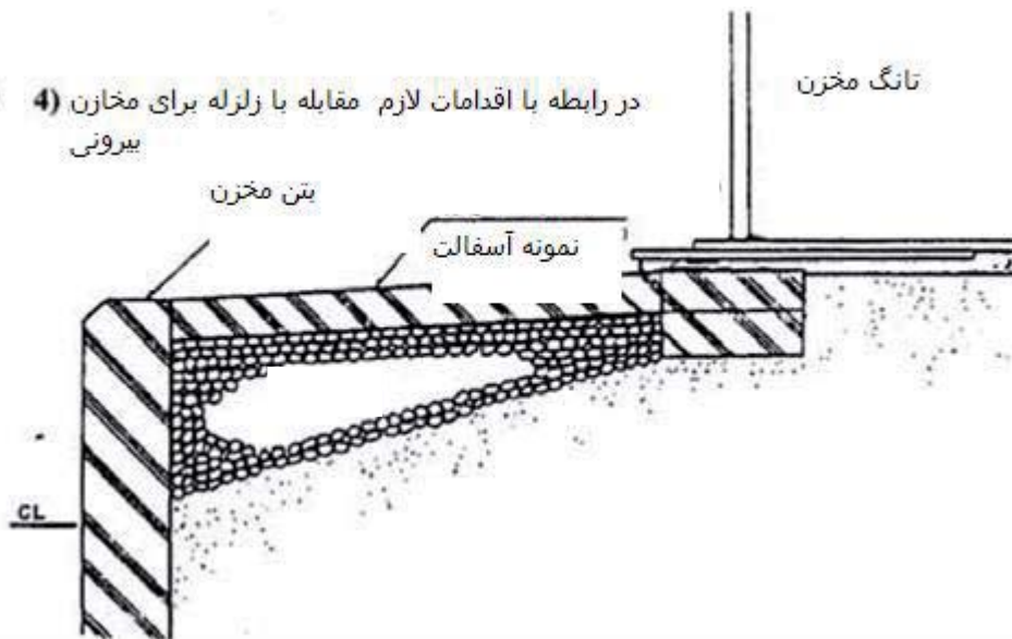
شکل ۶-۲۱ روش تقویت پی مخازن
