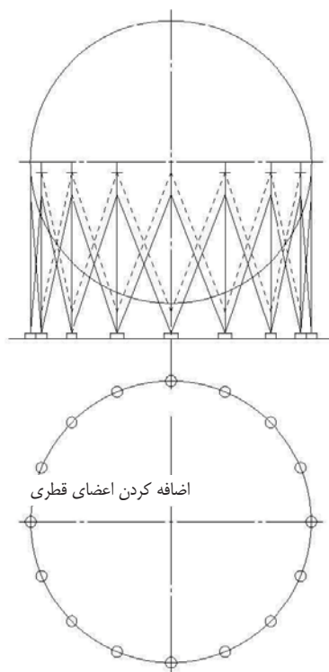
شکل ۳۰-۵ تقویت با اضافه کردن بادبند مهاری
