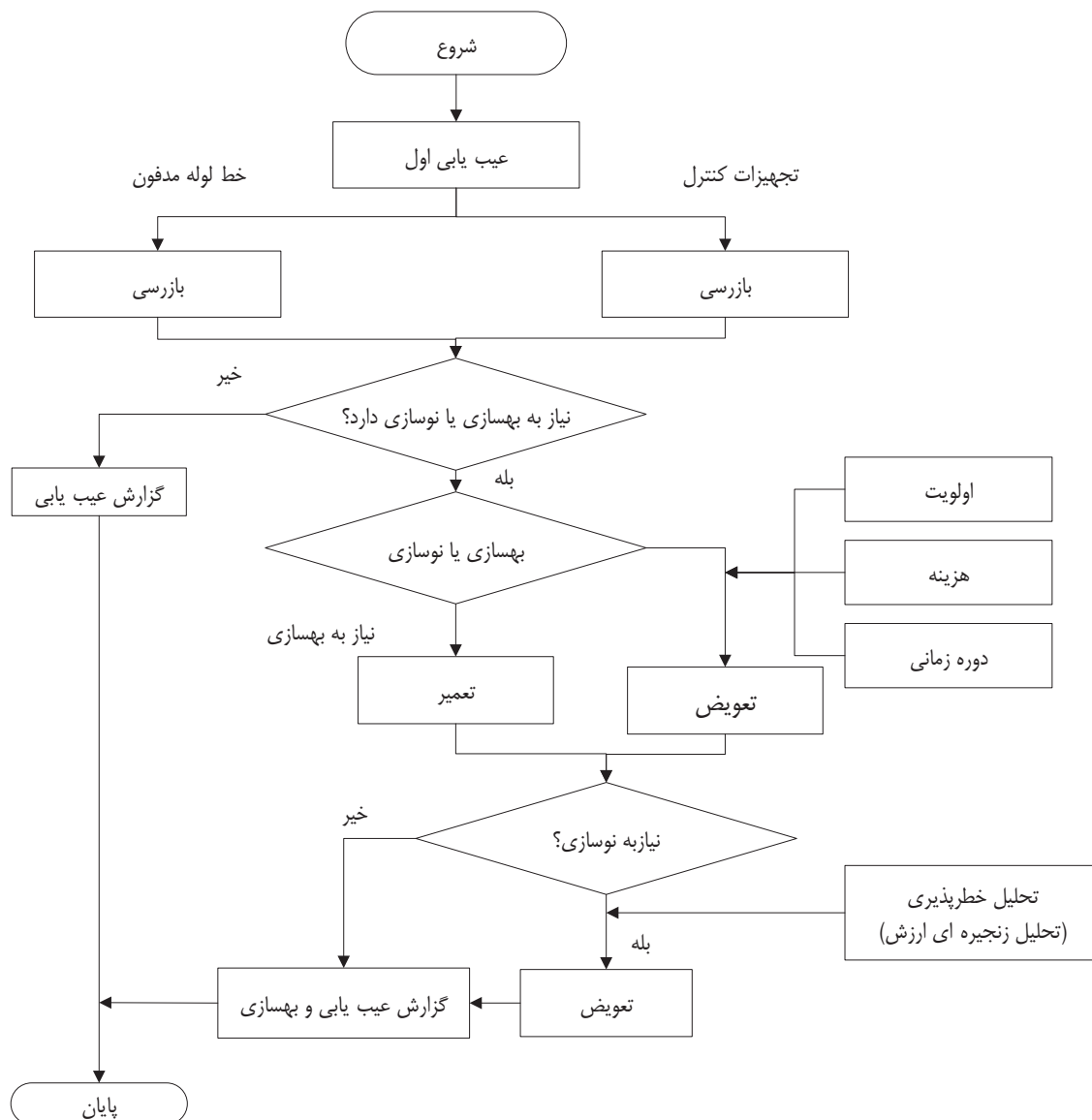
شکل ۸-۴ روند ارزیابی لوله‌های خط لوله مدفون و تأسیسات کنترل آن
