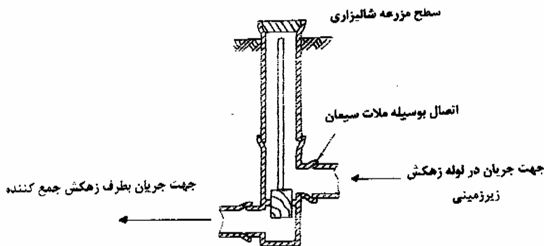
شکل (۴-۱)- شمای یک عدد چاهک کمکی (Relief well) و اجزای آن
