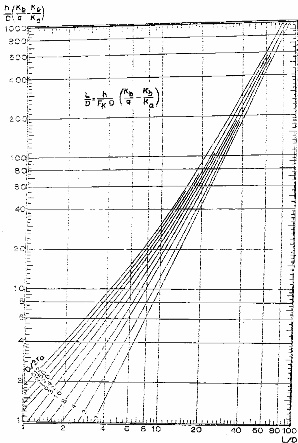
شکل (۴-۵) - نمودار تعیین فاصله زهکش های زیرزمینی به روش کرکهام (تعدیل شده بوسیله توکسوز و کرکهام، ۱۹۶۱)
