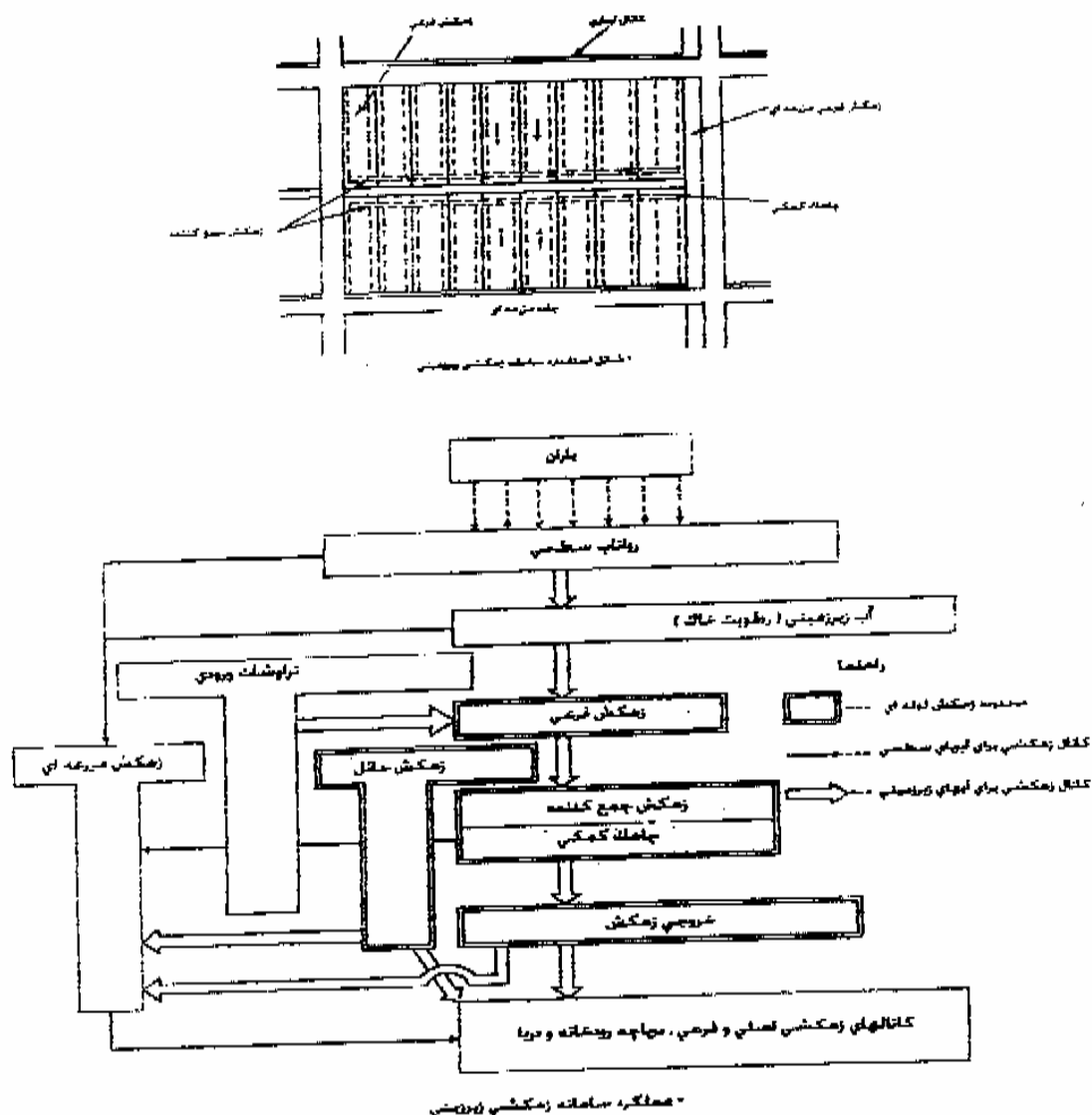
شکل (۴-۱۰) - اجزای سامانه و عملکرد (کارآمدی) زهکش زیرزمینی
