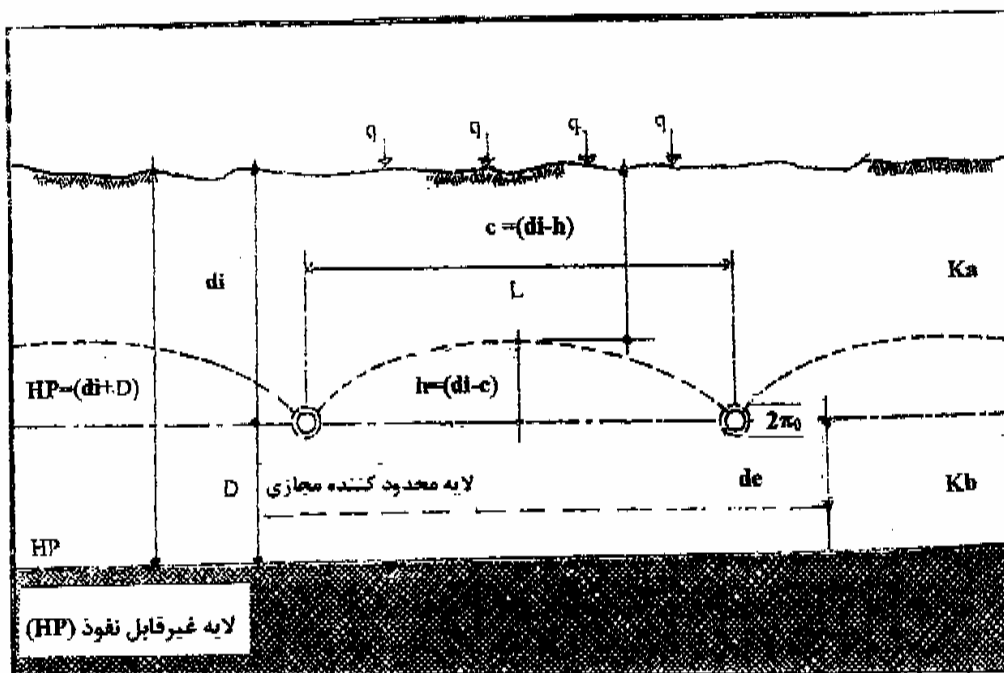
شکل (۴-۴) - علایم و نشانه های بکار رفته در اشتقاق روابط مبتنی بر حالت جریان همگام (ماندگار) زهکشی زیرزمینی و شرایط تعدیل شده آن (معادله های هوخهات و کرکهام)
