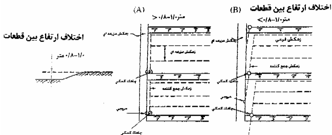
شکل (۸-۴) - نمونه ای از سامانه زهکشی زیرزمینی در اراضی شیب دار
