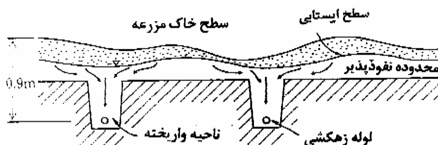
شکل (۳-۴) - چگونگی عملکرد سامانه زهکشی زیرزمینی
