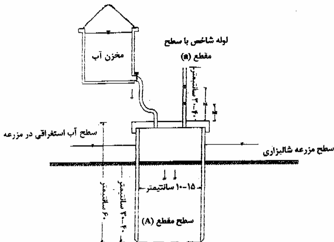
شکل (۴-۲) - شمای یک دستگاه اندازه گیری مقدار نفوذ آب به خاک به روش سریع
