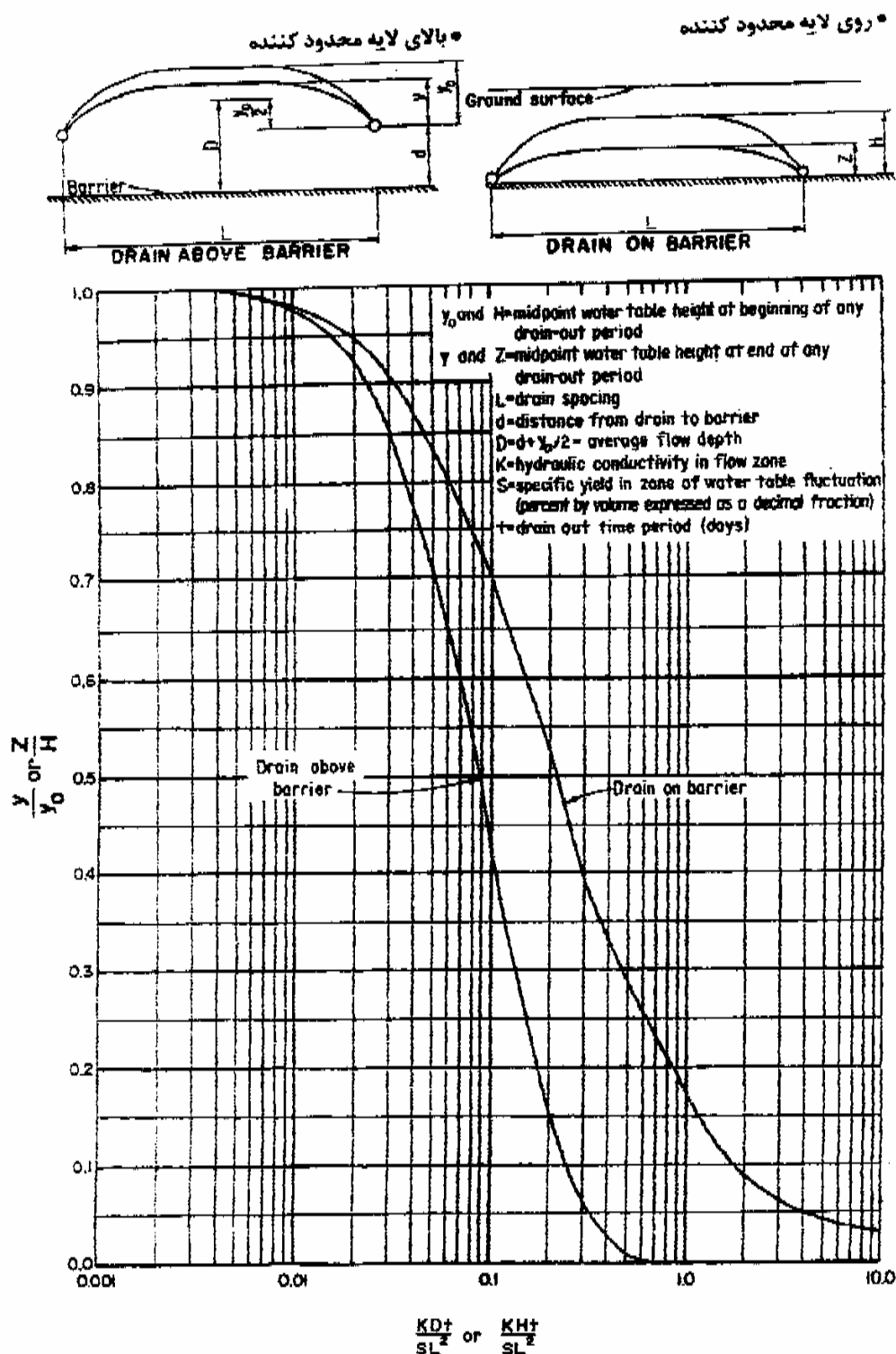
شکل (۶-۴) - علایم و نشانه های بکار رفته در اشتقاق رابطه "کلاور-دام" برای شرایط استقرار زهکشهای زیرزمینی (لوله ای) روی لایه محدود کننده (Barrier) و بالای آن
