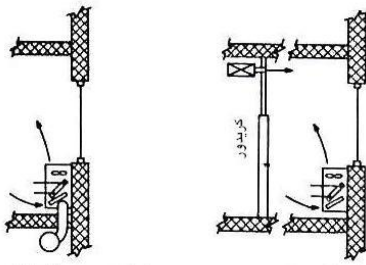
شکل ۱-۵: واحد فن کویل، زمانیکه هوای تازه اتاق توسط مرکز جداگانه‌ای تهیه می‌شود (سیستم هوا-آب)
