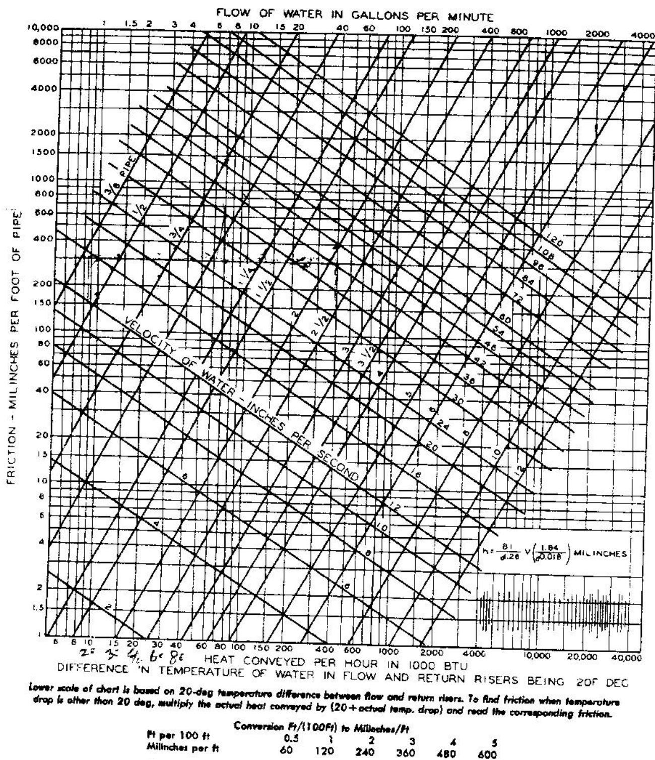
شکل ۲-۲: نرخ افت فشار ناشی از جریان آب در لوله‌های آهنی
