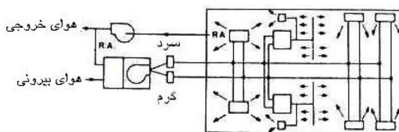
شکل ۹-۱: سیستم تمام هوای دو کاناله
