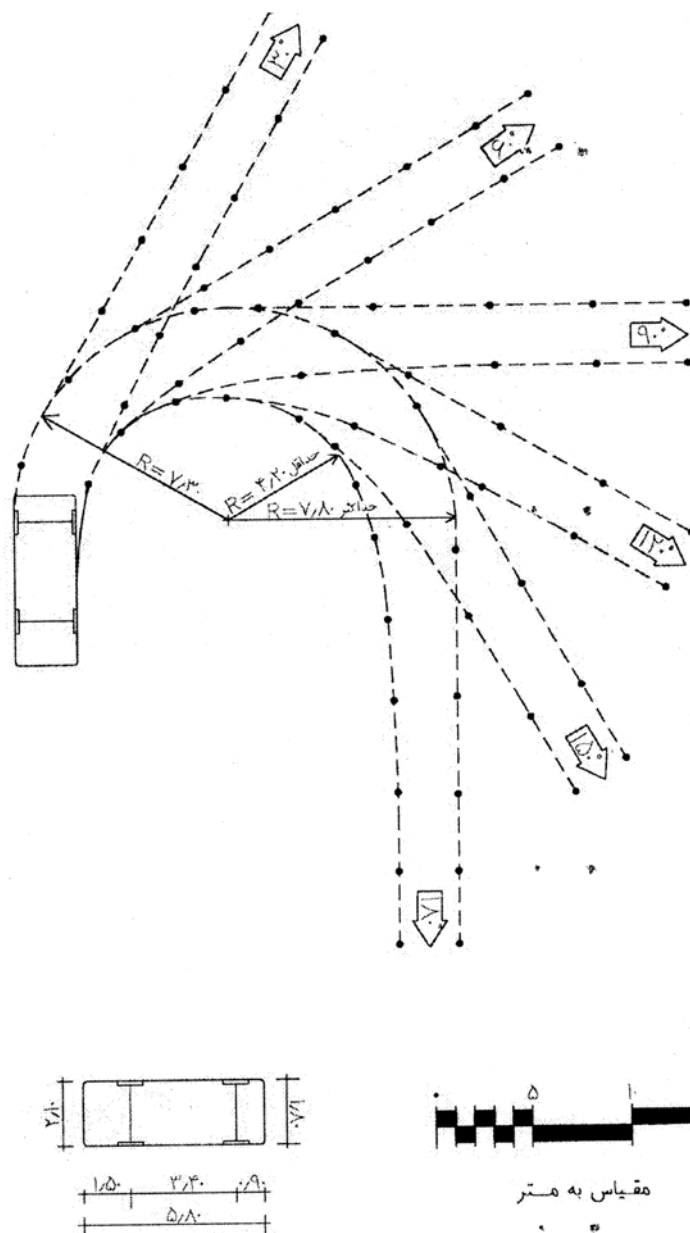
شکل ۳-۷: مشخصات مسیر گردش خودروی سواری
