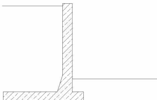
شکل ۳-۳: ترانشه دیواره‌ای با دیوار و پاشنه بتنی
