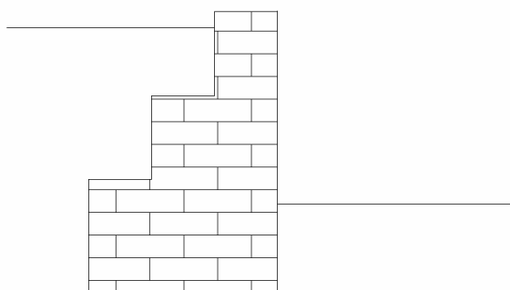
شکل ۳-۴: ترانشه دیواره‌ای با دیوار سنگ‌چین
