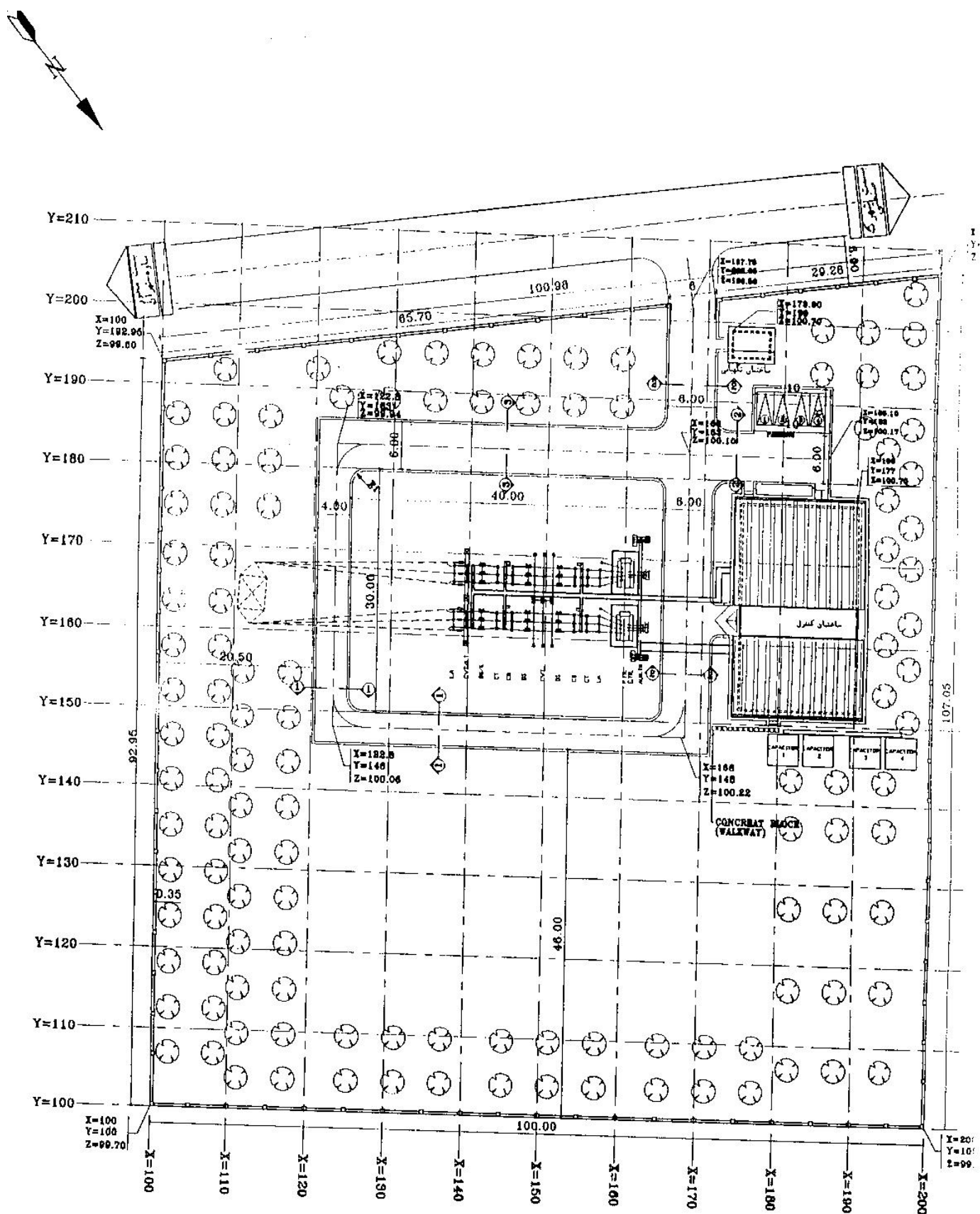
نقشه ۱: سایت پلان پست ۶۳/۲۰ کیلوولت پرندک
