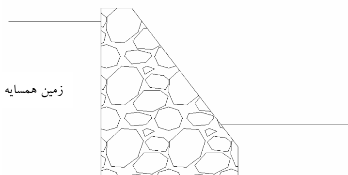
شکل ۳-۶: ترانشه دیواره‌ای با دیوار سنگ‌چین در مجاورت زمین همسایه
