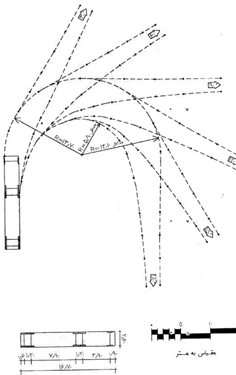
شکل ۳-۸: مشخصات مسیر گردش تریلی بزرگ
