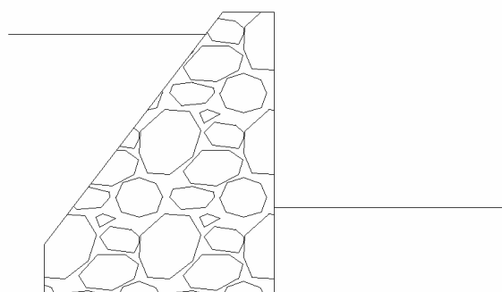
شکل ۳-۴: ترانشه دیواره‌ای با دیوار سنگ‌چین
