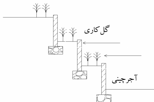
شکل ۳-۲: ترانشه پله ای
