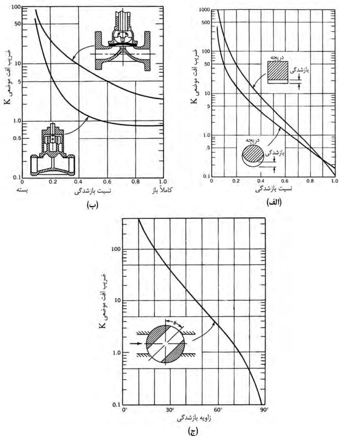
شکل الف-۶- تعیین ضریب افت موضعی انواع متداول شیر با توجه به میزان بازشدهگی آن،
