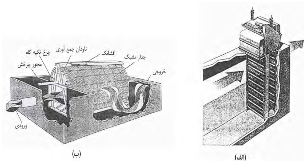
شکل ۸-۵- (الف) آشغال‌گیر دانه ریز از نوع متحرک، (ب) آشغال‌گیر از نوع ریز صافی
