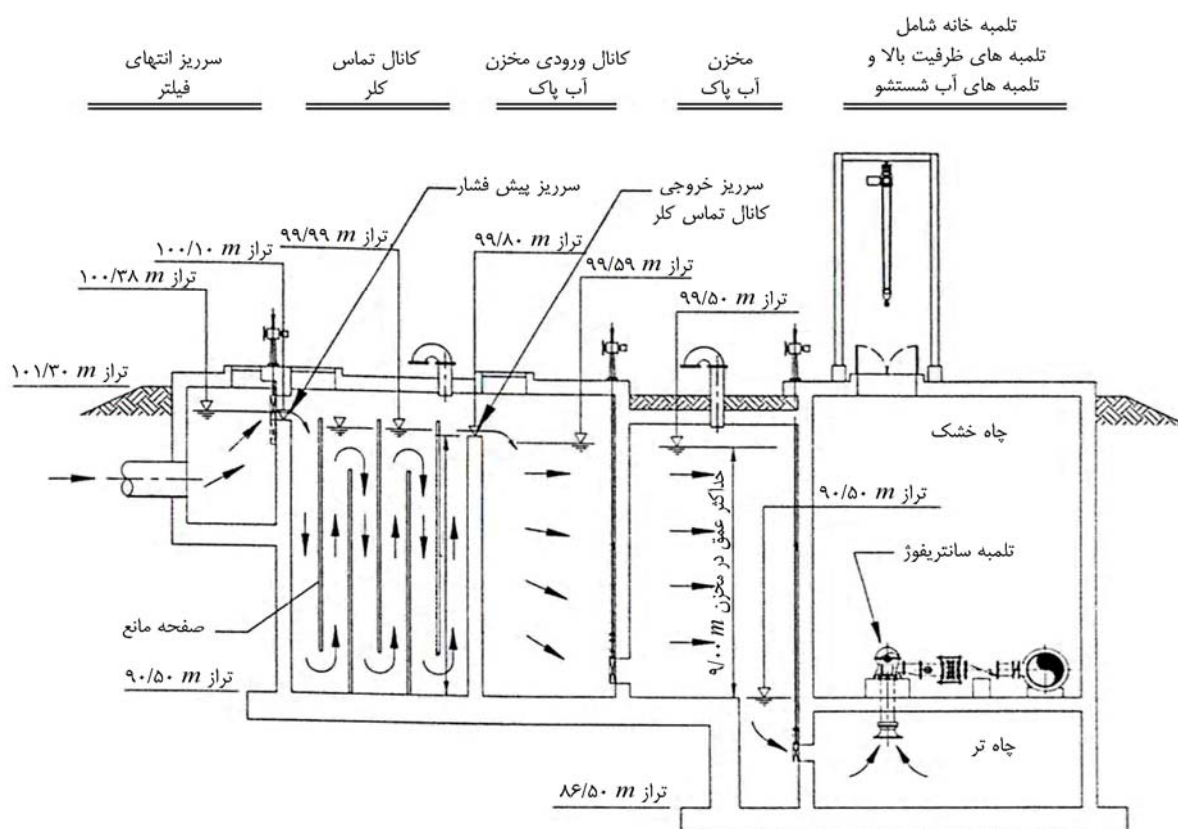
شکل ب-۲۴- نیمرخ هیدرولیکی در کانال تماس کلر و مخزن آب پاک
