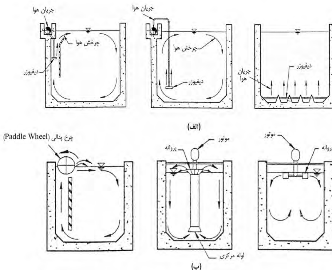
شکل ۸-۱۰- انواع متداول هواده‌های در تصفیه‌خانه آب، (الف) هواده‌های پخشی، (ب) هواده‌های مکانیکی
