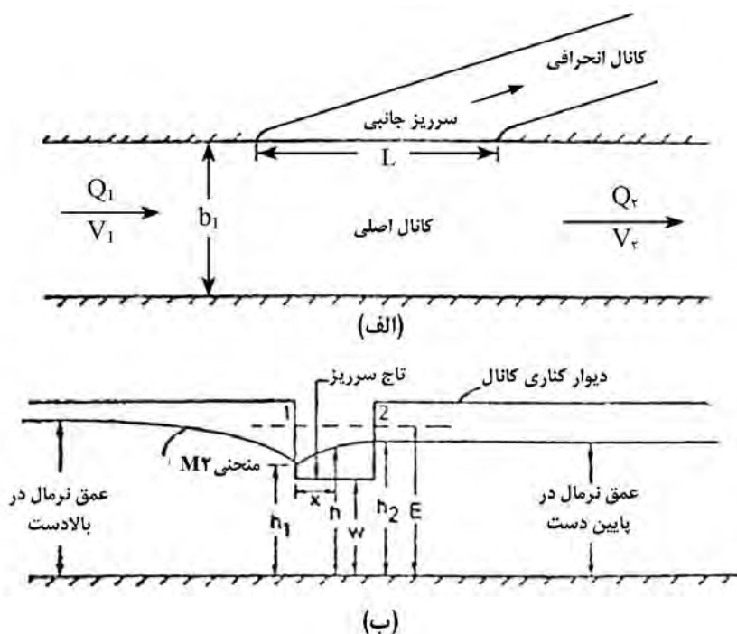
شکل ۳-۹- سرریز جانبی (الف) تصویر افقی، (ب) مقطع
