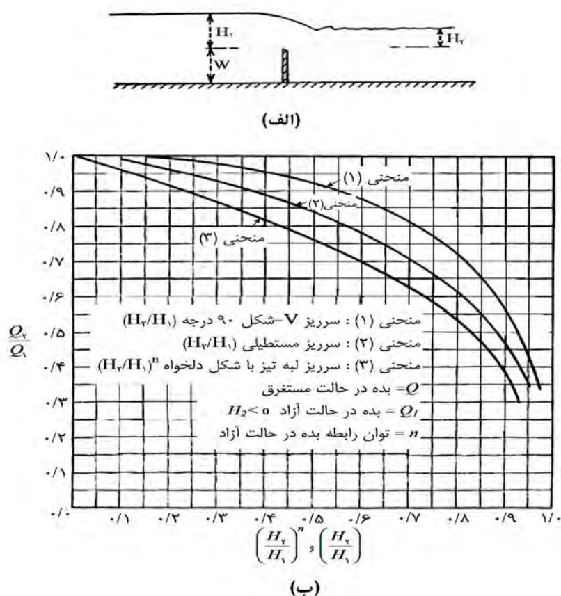
شکل ۵-۵- جریان در سرریز مستغرق، (الف) سرریز مستغرق، (ب) منحنی بده در حالت مستغرق [۴]
