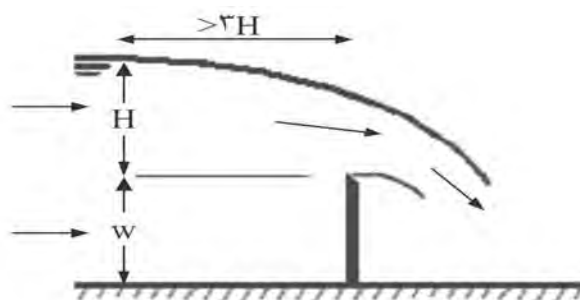
شکل ۵-۱- سرریز لبه تیز آزاد
