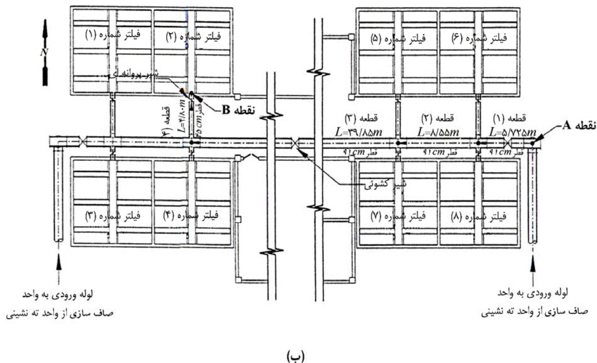
شکل ب-۱۸- جانمایی لوله‌های ورودی صافی برای محاسبه افت ارتفاع، (الف) توزیع جریان، (ب) جانمایی قسمت‌ها و ابعاد
