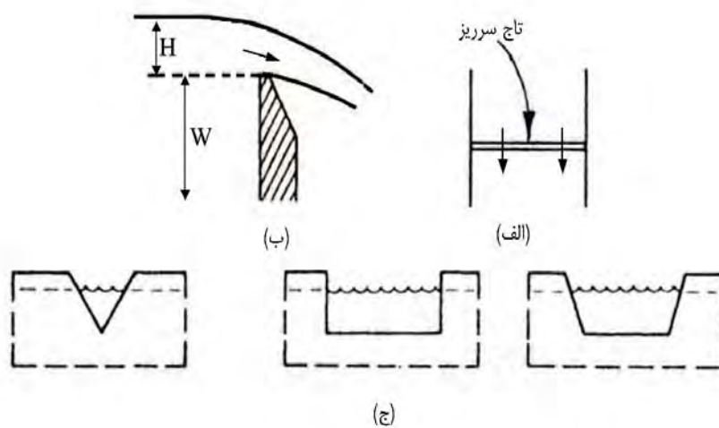
شکل ۷-۱۱ - سرریز اندازه‌گیری جریان، (الف) تصویر افقی، (ب) مقطع طولی، (ج) مقطع عرضی
