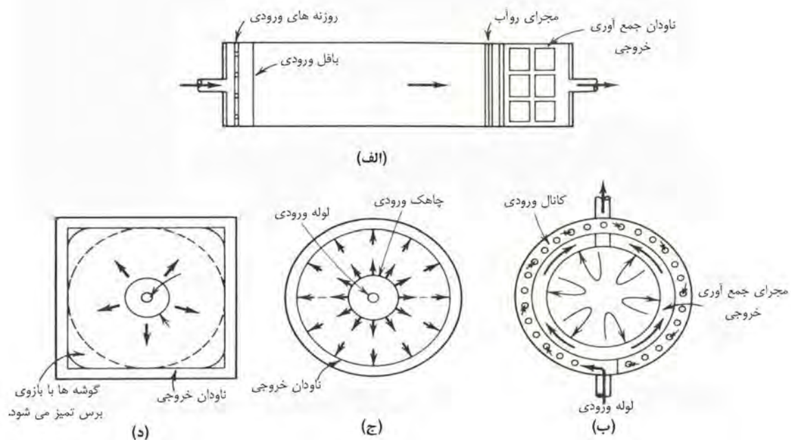
شکل ۱۰-۱- انواع مختلف هندسه حوض ته‌نشینی، (الف) مستطیلی، (ب) دایره‌ای با ورودی محیطی، (ج) دایره‌ای با ورودی از مرکز، (د) مربعی
