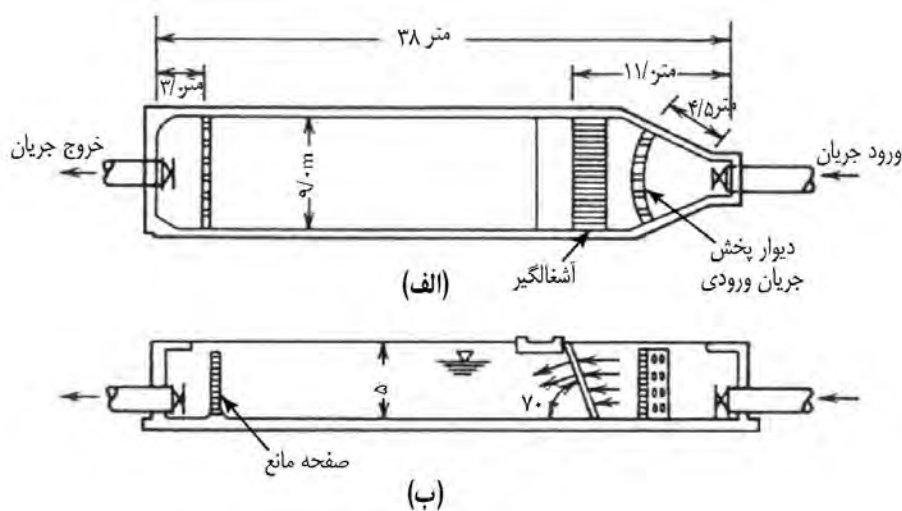
شکل ۸-۱۱- نمونه ای از حوض دانه گیر، (الف) تصویر افقی، (ب) مقطع طولی [۱۶]
