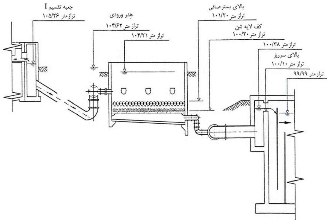
شکل ب-۲۰- نیمرخ سطح آب در طول واحد صافسازی (از انتهای واحد ته‌نشینی تا ابتدای مخزن ذخیره آب پاک)
