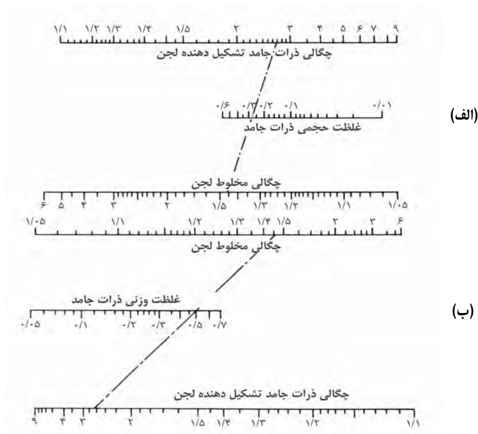
شکل ۴-۱- تعیین چگالی مخلوط لجن، (الف) روش غلظت حجمی، (ب) روش غلظت وزنی [۸]
