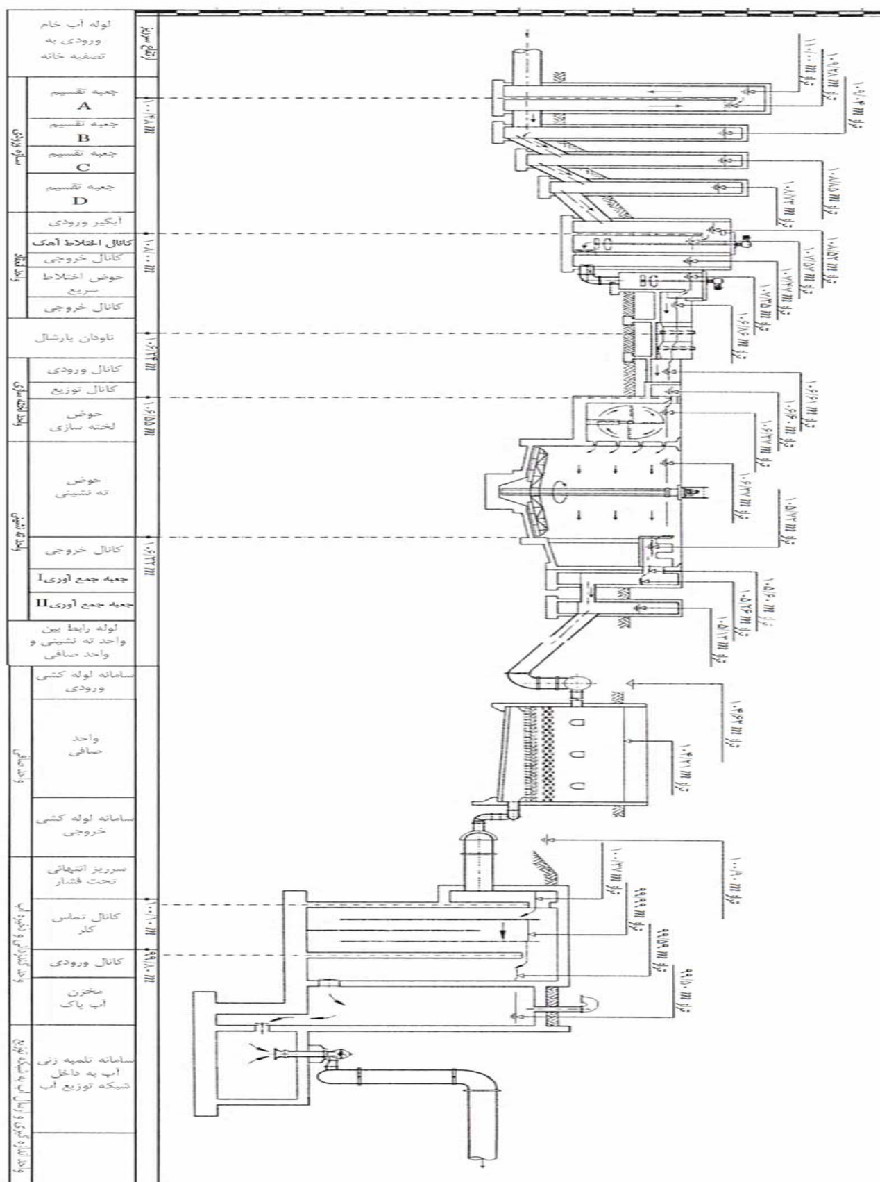
شکل ب-۲۵- نیمرخ سطح جریان در طول تصفیه‌خانه آب
