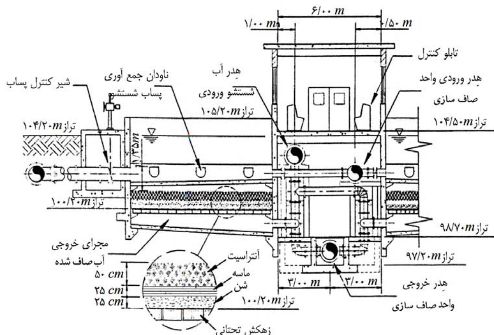
شکل ب-۱۷- برش از صافی شامل بستر ماسه، بستر شنی نگهدارنده، زهکش‌ها و سامانه ناودان‌های جمع‌آوری آب شستشو
