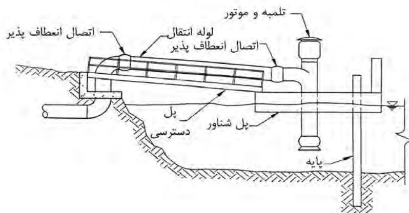
شکل ۸-۱- آبگیر شناور
