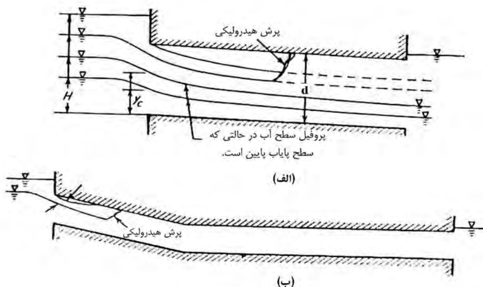
شکل ۵-۹- آبرو، (الف) انواع جریان در آبرو با شیب ثابت، (ب) آبرو با شیب متغیر
