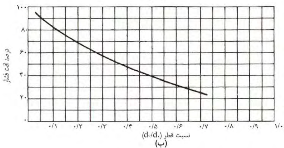
شکل ۷-۷- نمونه‌ای از منحنی‌های تعیین ضریب افت فشار در شیپوره [۱۵]
