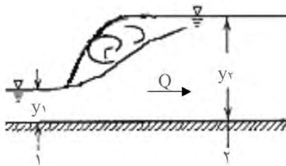
شکل ۳-۳- پرش هیدرولیکی
