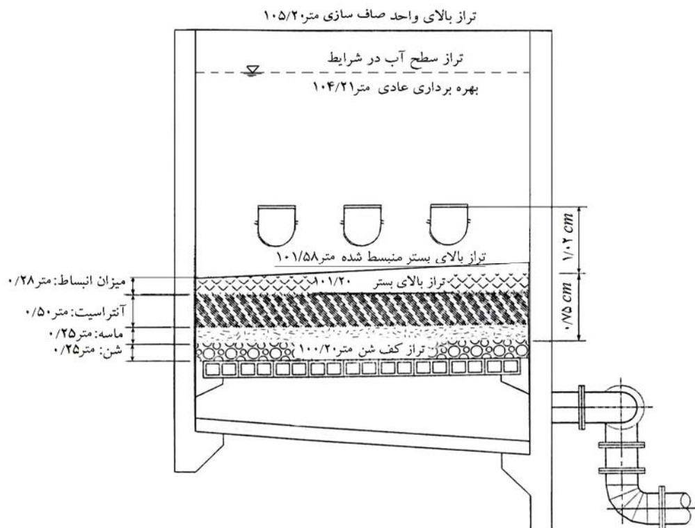
شکل ب-۲۱- مشخصات طراحی ناودان‌های جمع‌آوری آب شستشو
