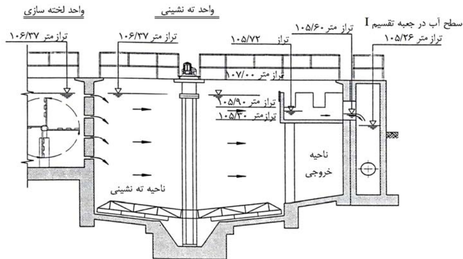
شکل ب-۱۴- نیمرخ هیدرولیکی جریان در واحد ته نشینی
