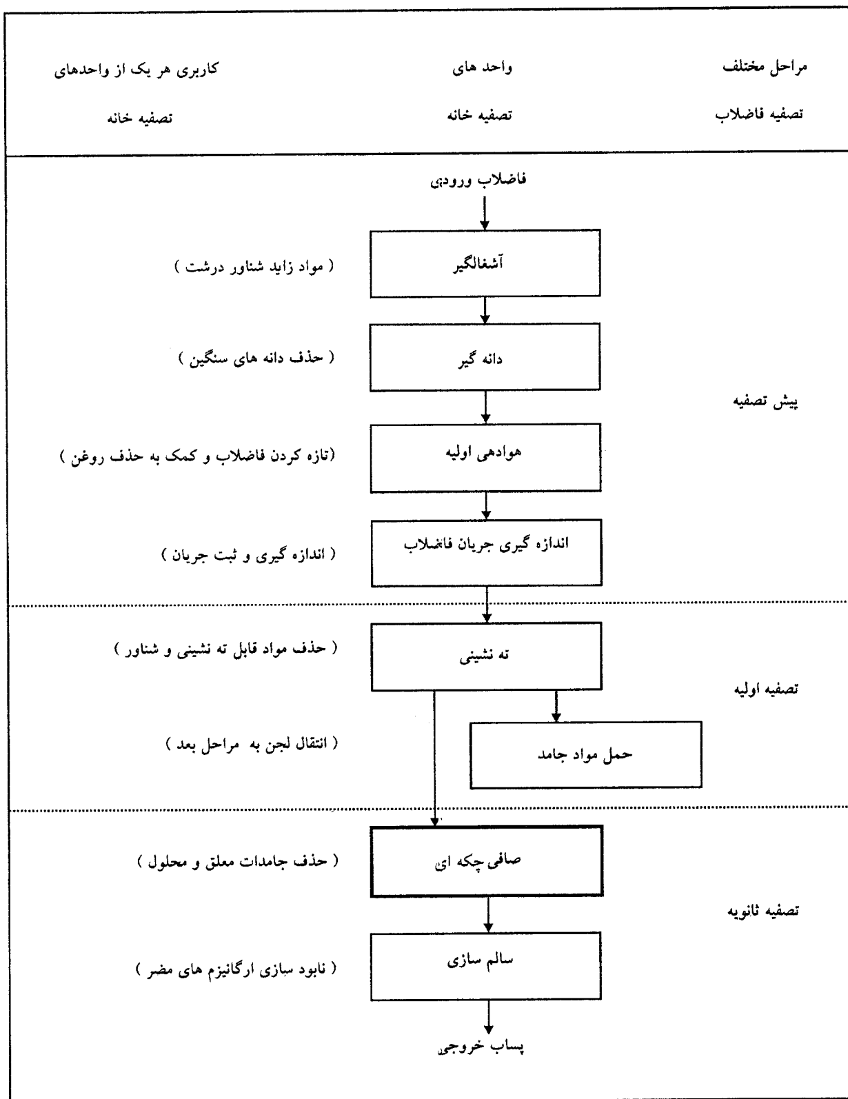
نمودار ۳-۱- موقعیت صافی چکه ای در تصفیه خانه فاضلاب
