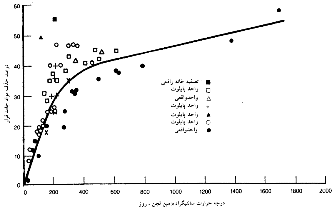
شکل ۴-۱۵- حذف مواد جامد فرار به عنوان تابعی از درجه حرارت و سن لجن
