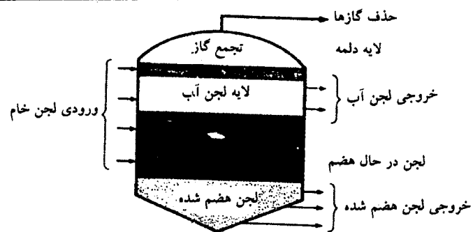
الف ( نمونه ای از یک هاضم کند
