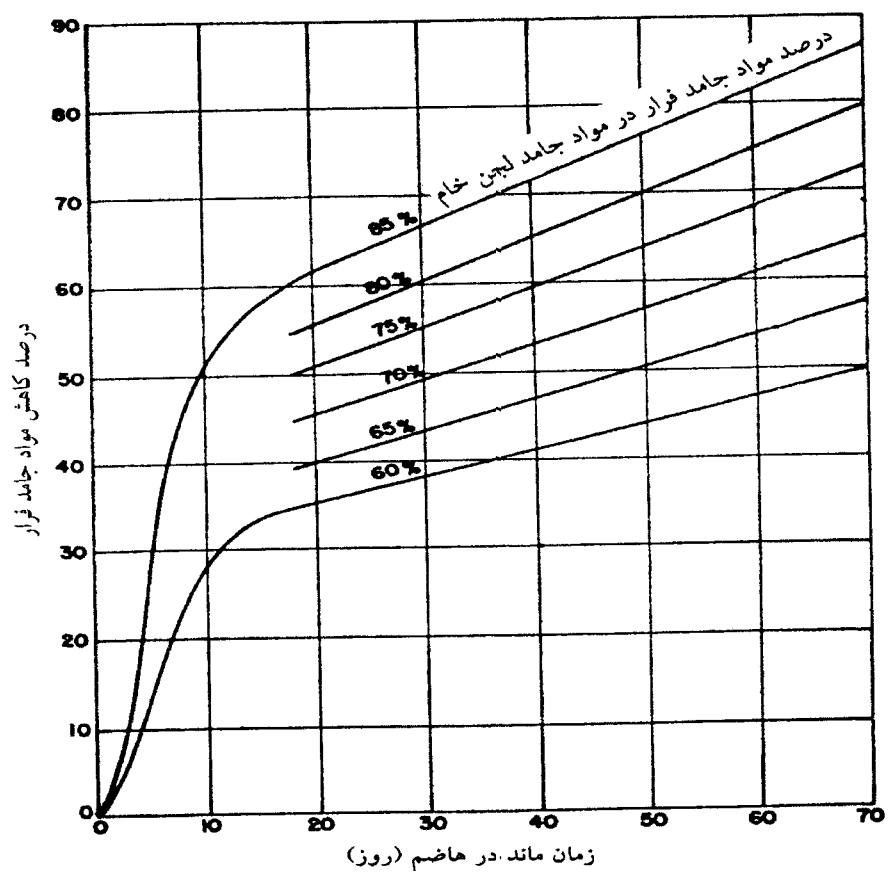
شکل ۳-۴ - کاهش مواد جامد فرار در لیجن های مختلف در برابر مدت زمان هضم
