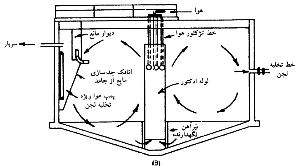
شکل ۴-۱۴- نمونه ای از هاضم هوازی با عملکرد پیوسته
