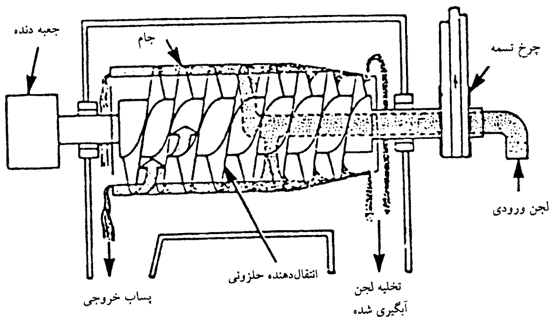
شکل ۴-۱۸- دستگاه سانتریفوژ (جام جامدات) با جریان مخالف
