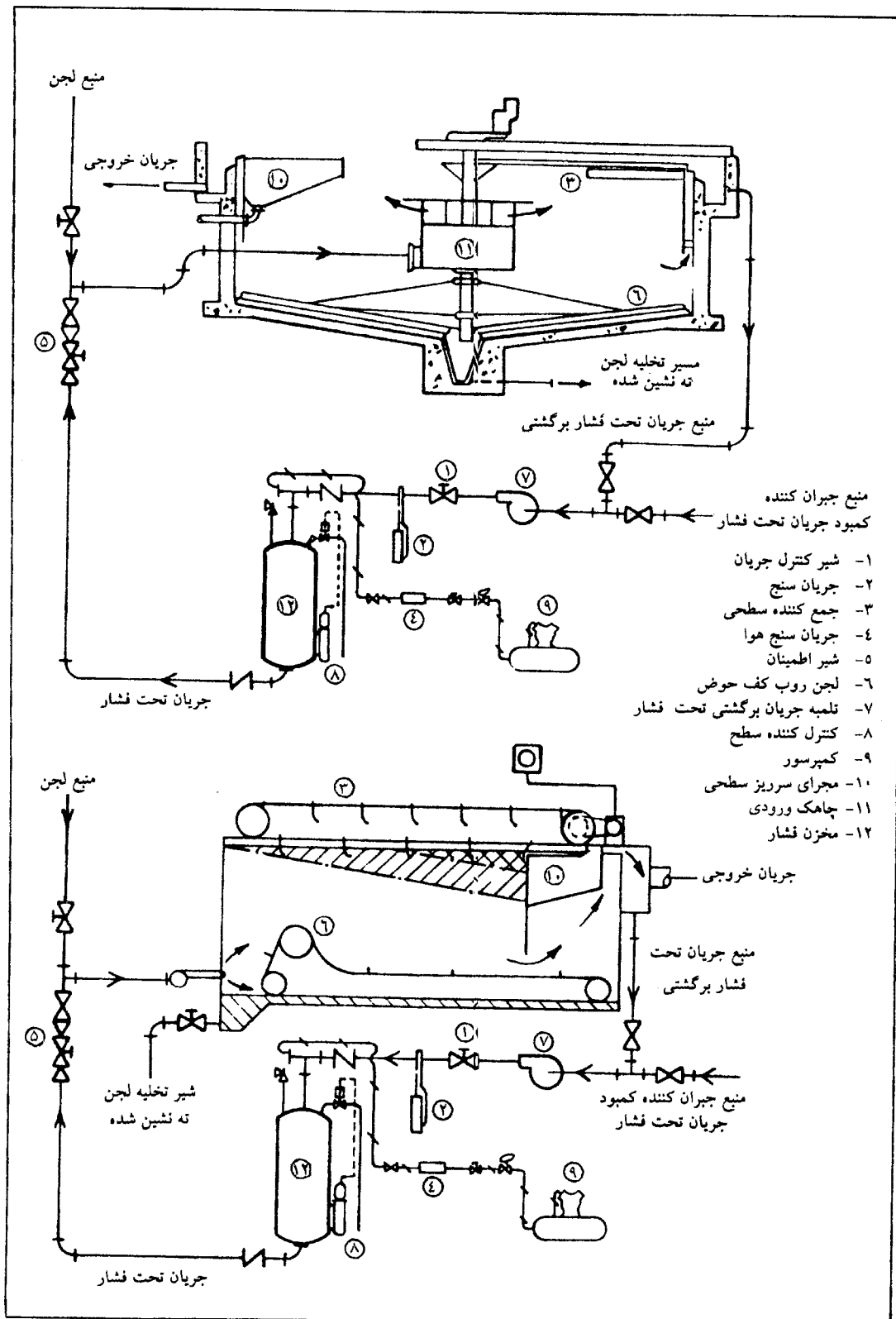
شکل ۴-۱۷- طرح‌هایی کلی از حوض‌های تغلیظ‌کننده متعارف با فرایند شناورسازی به کمک هوای محلول
