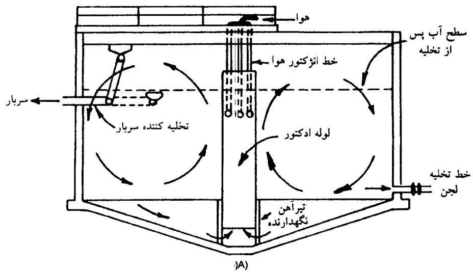
شکل ۴-۱۳- نمونه ای از هاضم هوازی با عملکرد نوبتی
