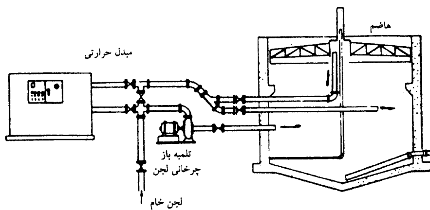
شکل ۴-۷- نمونه ای از سیستم حرارت دهی به وسیله مبدل حرارتی نصب شده در خارج از هاضم
