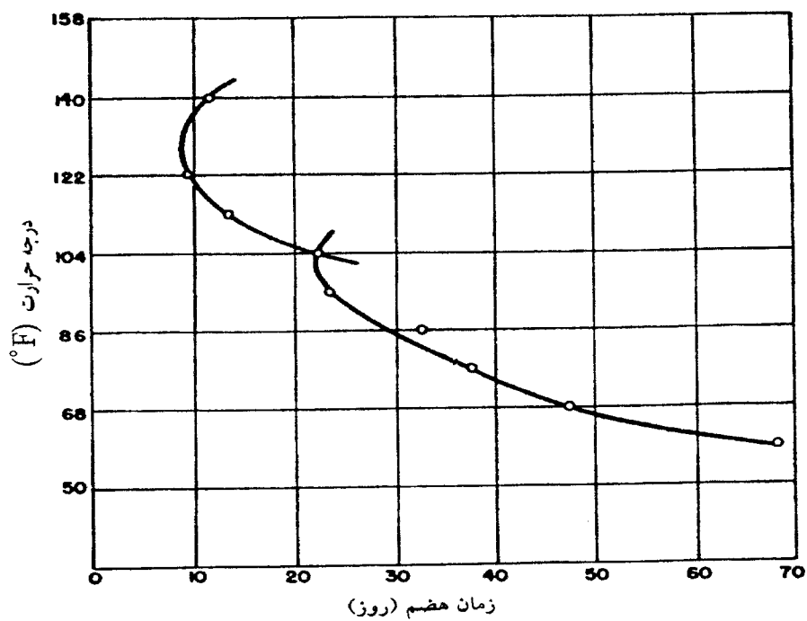
شکل ۴-۴ - رابطه مدت زمان هضم و درجه حرارت
