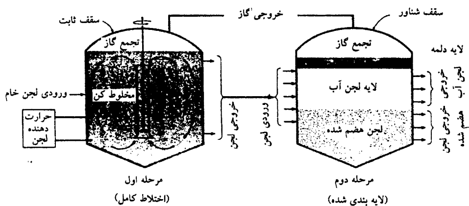
ب ( نمونه ای از یک هاضم سریع
