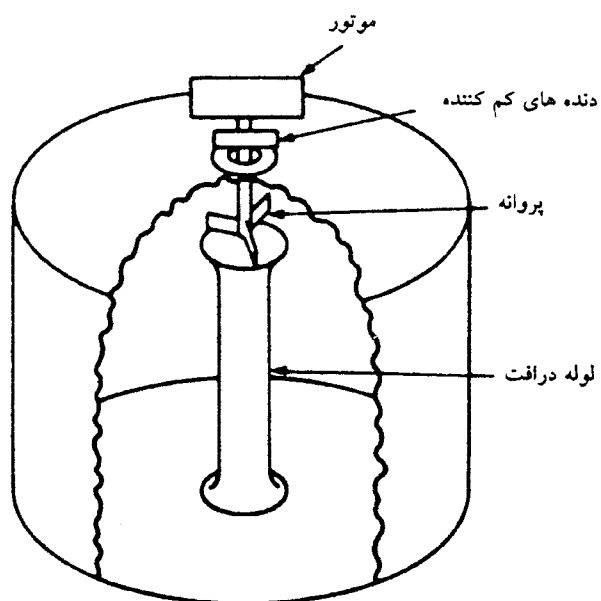
شکل ۴-۱۰- اختلاط لجن به وسیله بهم زن مکانیکی
