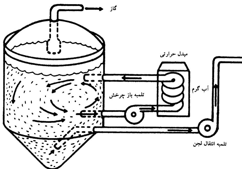
شکل ۴-۹- اختلاط هاضم به وسیله باز چرخش لجن
