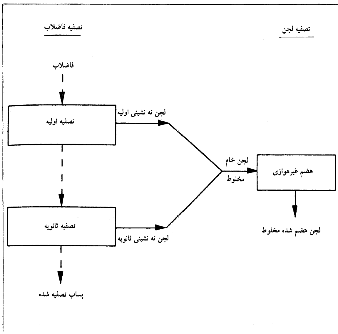
شکل ۴-۱- روابط بین فرآیندهای تصفیه فاضلاب و جریان لجن
