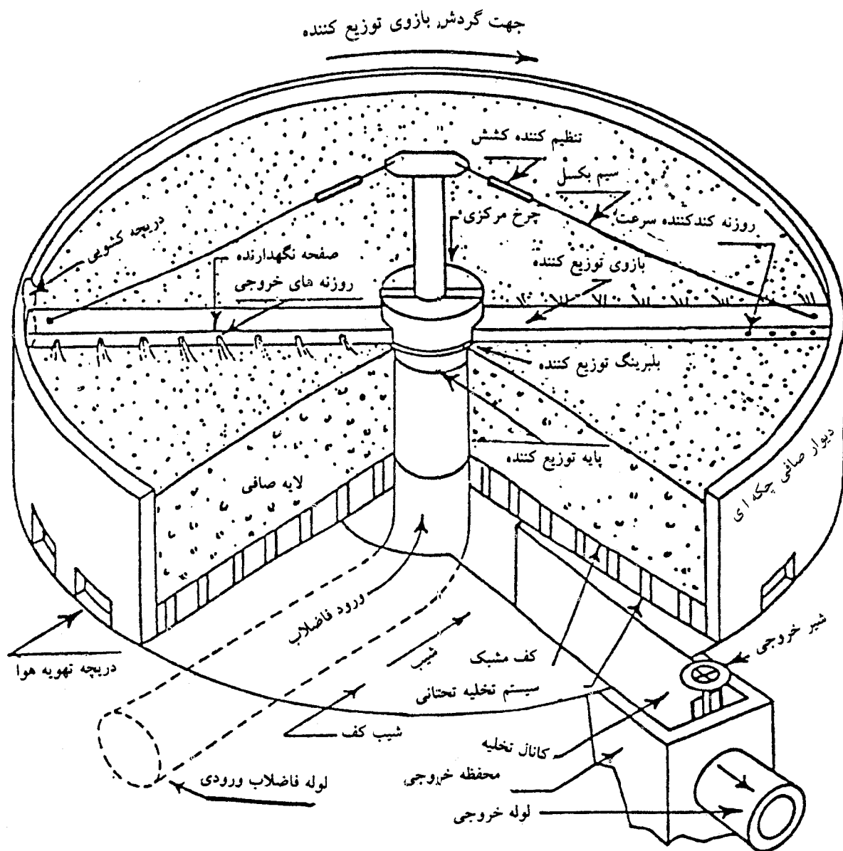
شکل ۳-۱- ساختمان یک صافی چک ای
