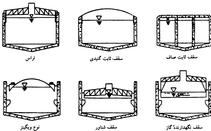
ج ( انواع سقف هاضم غیر هوازی
