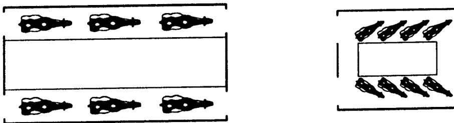
(شکل شماره ۱۷) مقطع سالن شیردوشی و گود ایستادن کارگر
