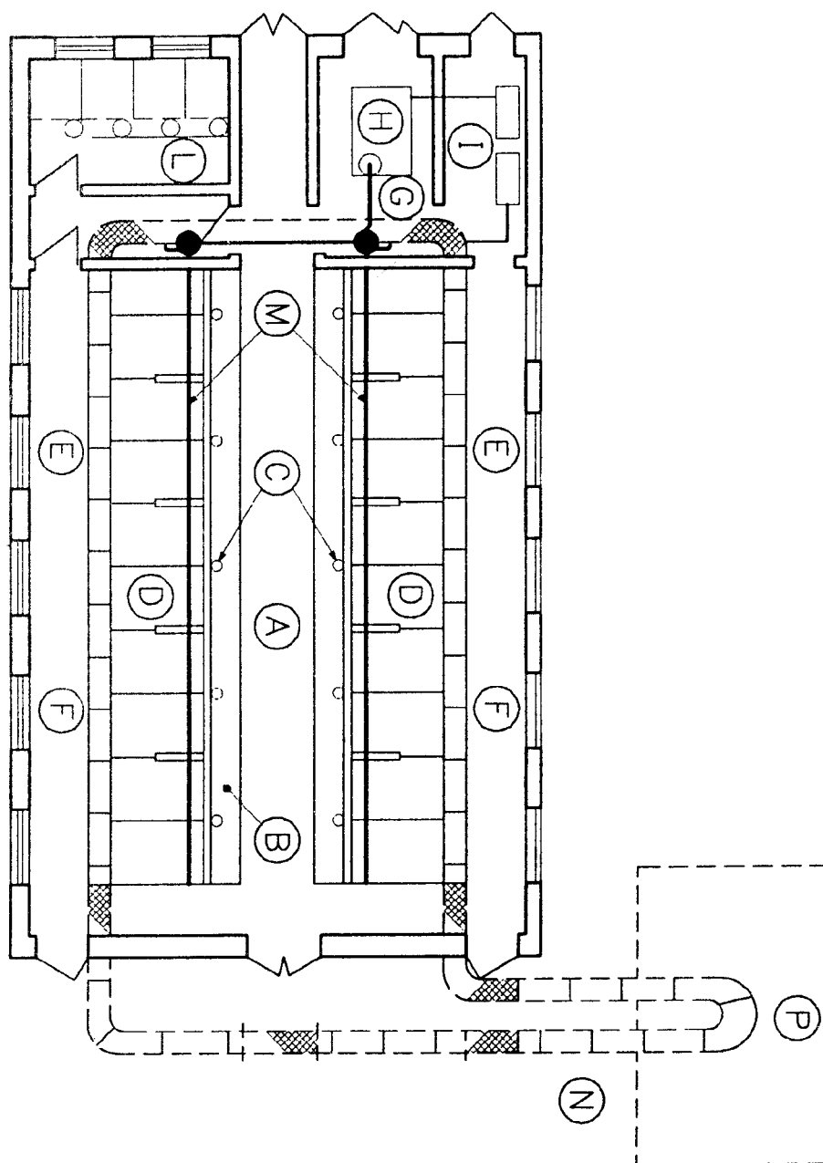
(شکل ۶) ساختمان جایگاه نگهداری سربه سر در سیستم بسته
