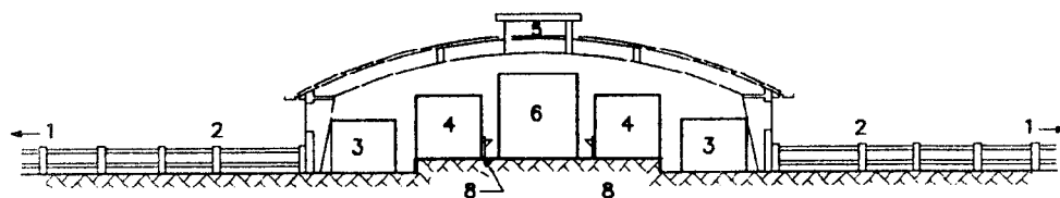
(شکل شماره ۱۲) سیستم تلفیقی (شمای کلی)
