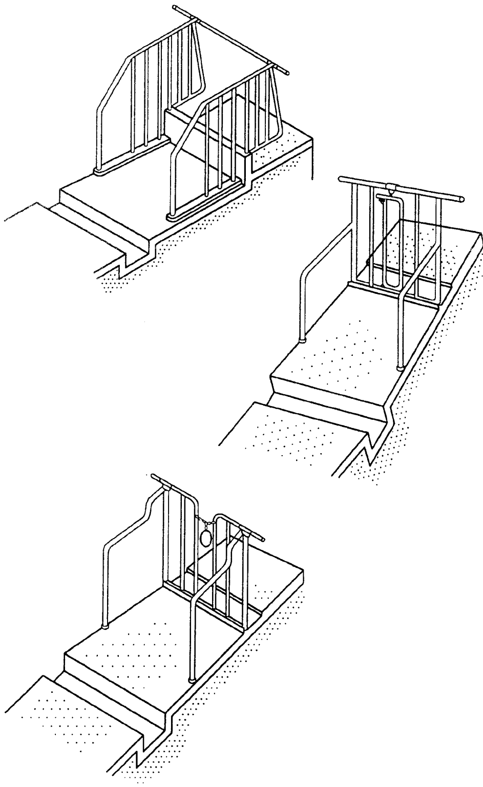
(شکل شماره ۴) سه نوع جایگاه انفرادی "استال"
