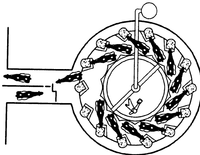
سالن شیردوشی دوار
