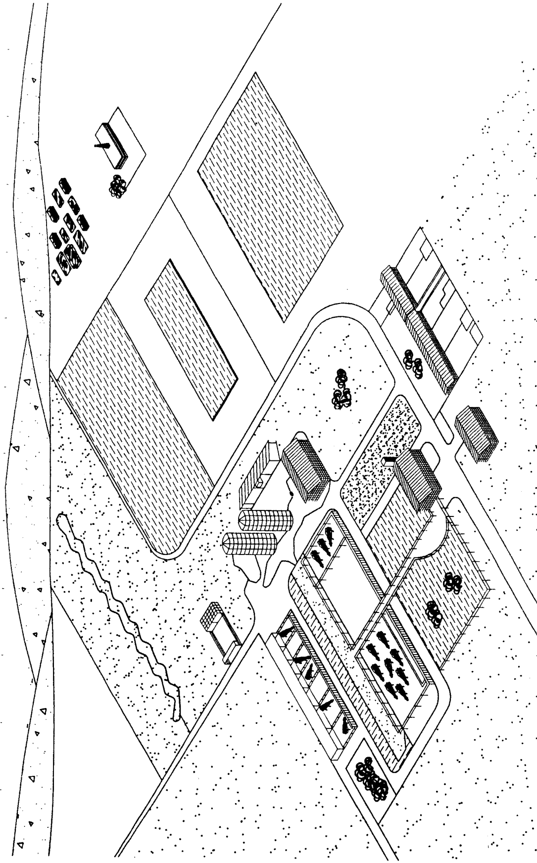
(شکل ۴-۲) نمای کلی ساختمانها و ارتباطات در یک محوطه گاوداری
