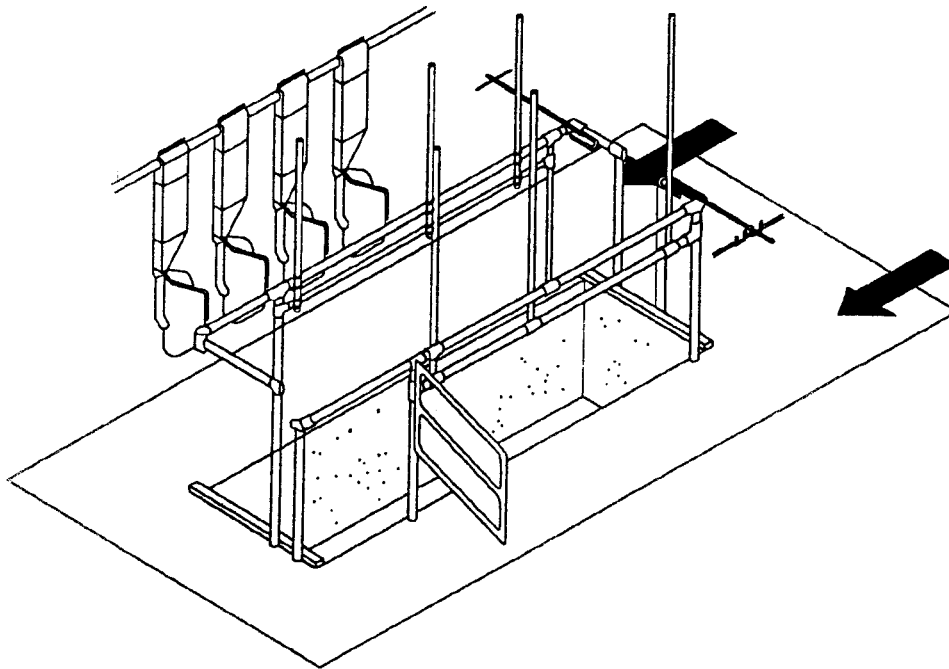
(شکل شماره ۱۹) اشکال گوناگون سالن شیردوشی و اشکال گوناگون گود شیردوشی
