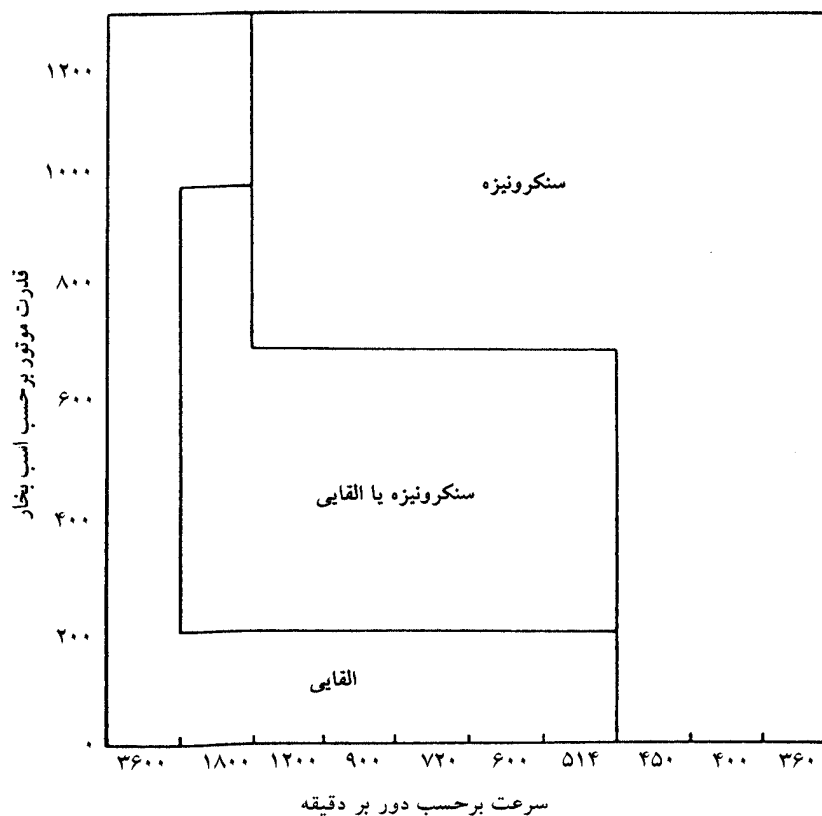
نمودار ۳- راهنمای انتخاب نوع موتور
