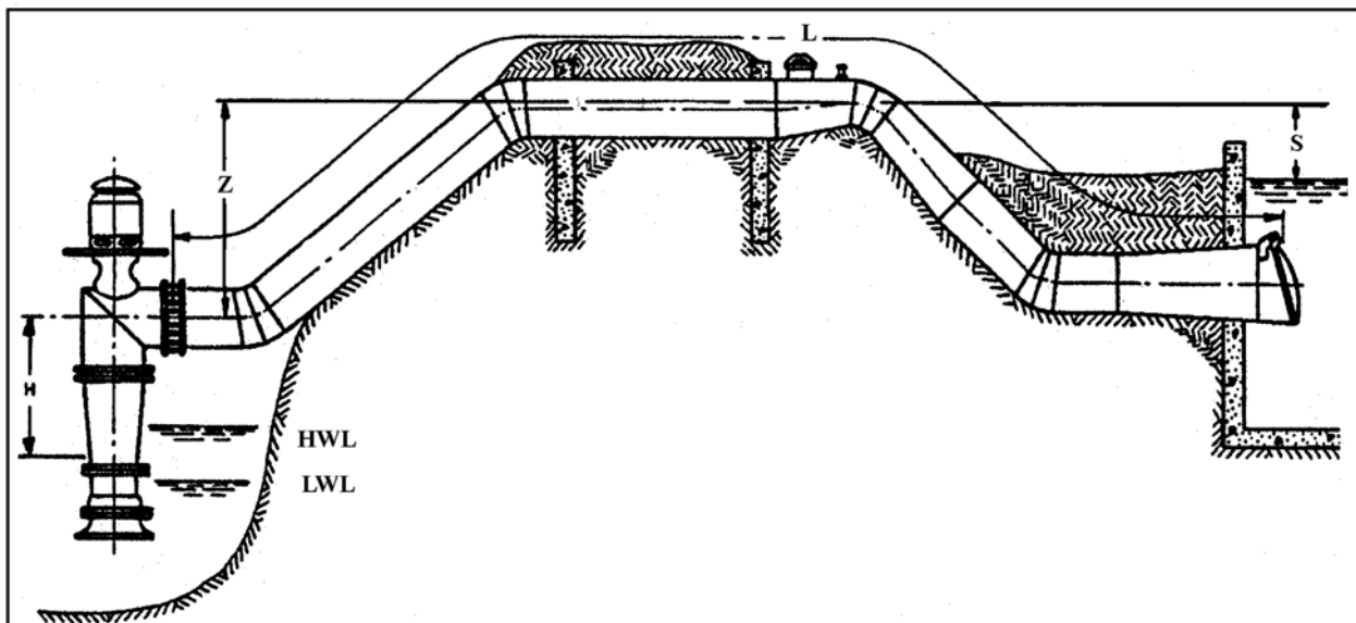
شکل ۵- انواع جاگذاری و نصب پمپ‌ها، HWL، LWL معادل سطح آب حداکثر و حداقل، L طول، H ارتفاع تا محور لوله آبده و Z بلندی لوله آبده، D قطر لوله آبده، و S متوسط ارتفاع سیفونی لوله آبده
