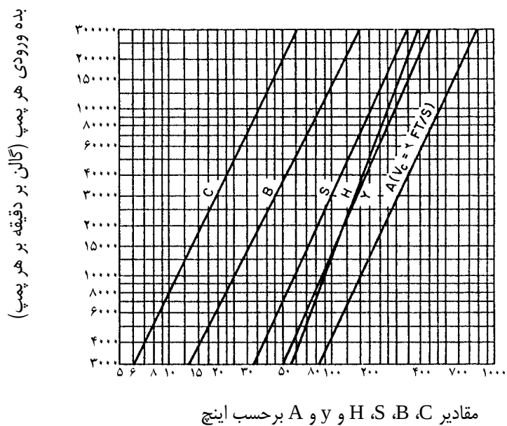
نمودار ۱- ابعاد حوضچه مکش در رابطه با بده پمپ
