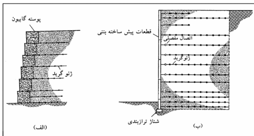
شکل ۱۳-۴- دیوارهای مسلح شده با ژئوگرید. (الف) پوسته گابیون، (ب) پوسته با قطعاعات پیش ساخته بتنی
