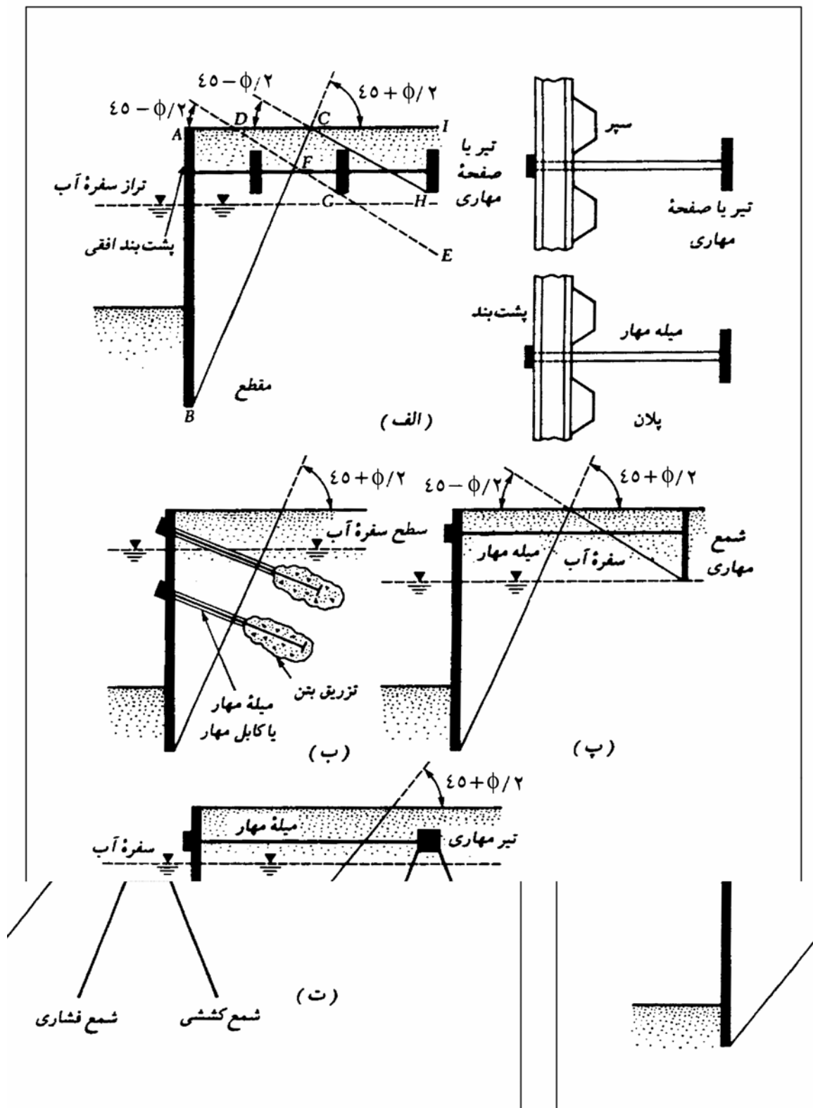
شکل ۱۰-۲۰- انواع مختلف مهار سپرها. (الف) تیر یا صفحه مهار، (ب) مهار با انتهای تزریق شده، (پ) شمع مهار قائم، (ت) تیر مهار با شمع های مایل.
