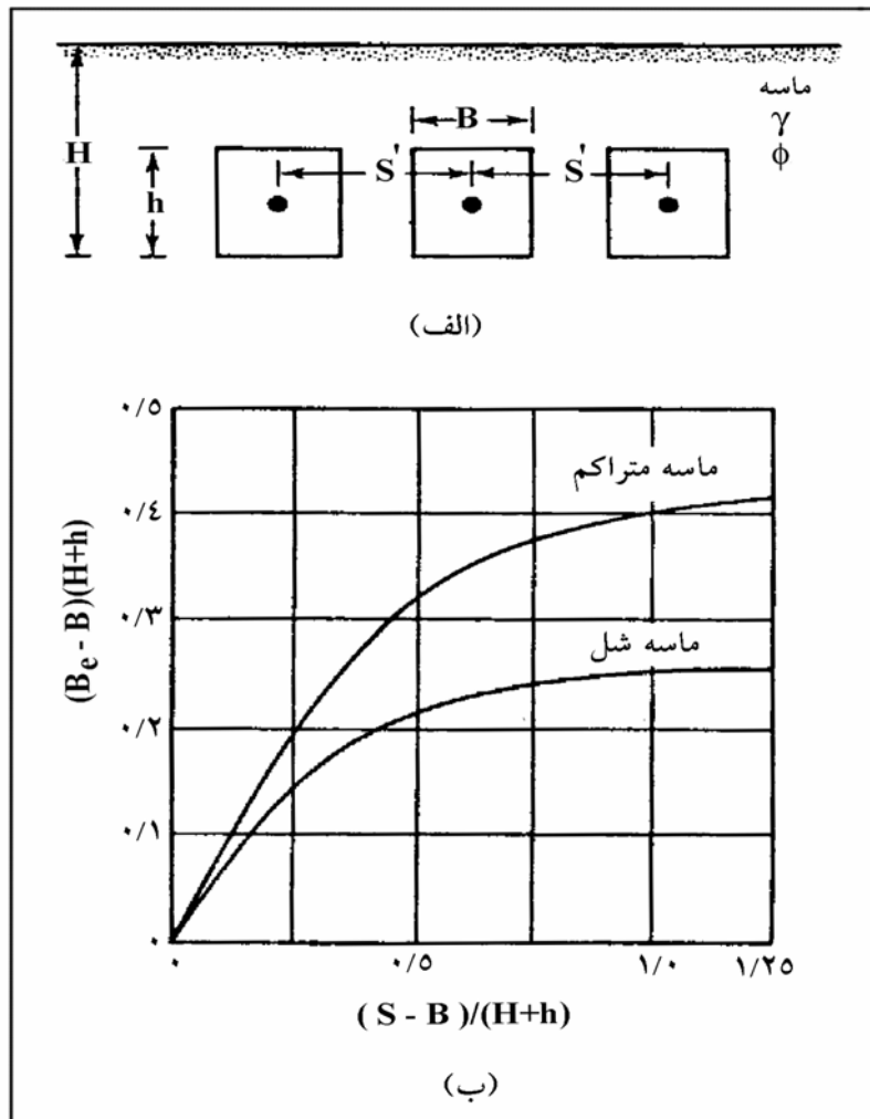
شکل ۱۰-۲۵ - (الف) حالت واقعی نصب مهاریه‌ها، (ب) تغییرات (B_e - B)/(H + h) در مقابل (S' - B)/(H + h) بر پایه تحلیل اوسن و استرومن
