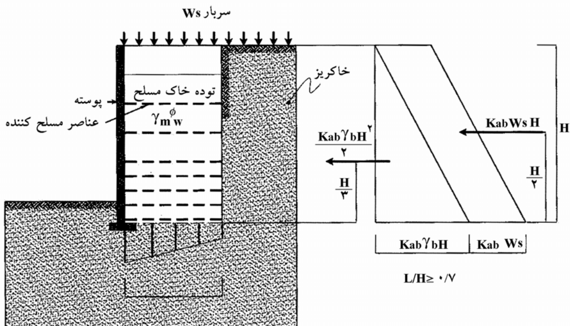
شکل ۱۲-۱۵- نیروهای وارد بر سازه خاک مسلح
