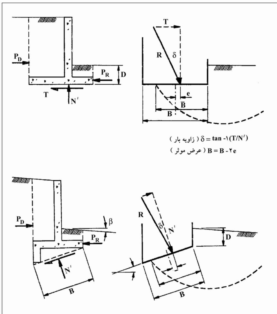
شکل ۵-۲- پارامترهای به کار رفته در رابطه ظرفیت باربری
