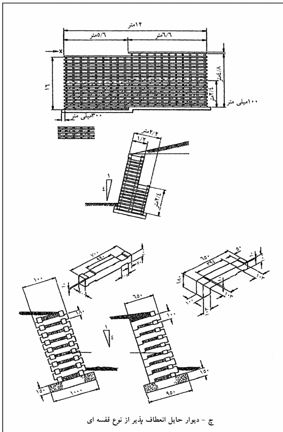
شکل ۱-۲ - انواع دیوارهای حایل (ادامه)
