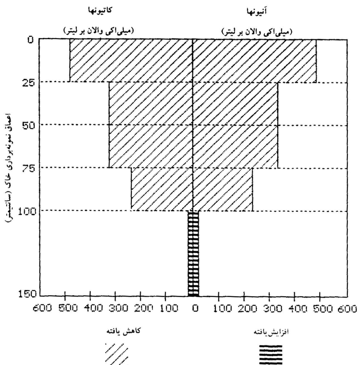
شکل ۷- تغییرات مجموع کاتیونها و آنیونها و انیونهای عصاره اشباع لایه‌های مختلف خاک طی فرآیند آبشویی املاح محلول در آزمایش مثال شماره یک
