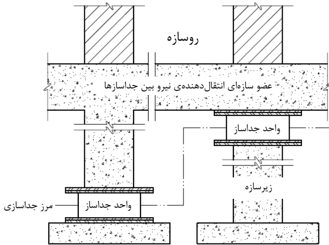
شکل ۹-۲ جداساز و اجزای سازه‌ی متصل
