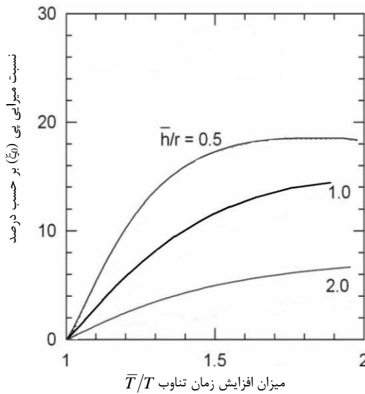
شکل ۵-۳ نسبت میرایی پی
