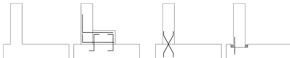
اتصال گیردار
