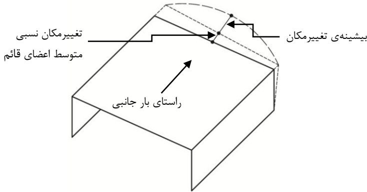
شکل ۳-۴ بررسی صلبیت دیافراگم
