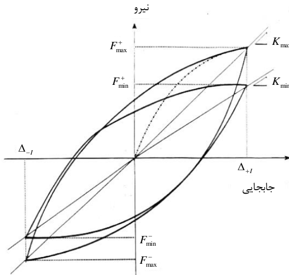
شکل ۳-۹ تاثیر سختی در رفتار چرخه‌ای هر جداساز
