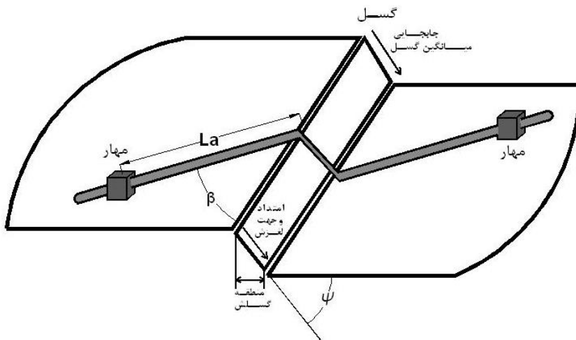
شکل ۳-۱۳ عبور لوله از گسل نرمال
