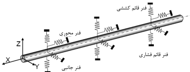
شکل ۱۳-۷ مدل سازی اندرکنش لوله - خاک با فنرهای غیرارجاعی
