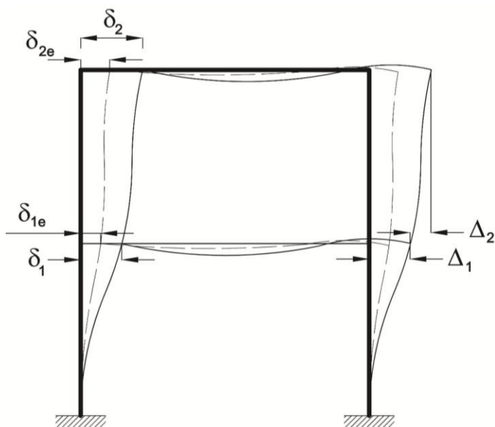
شکل ۶-۴ نمایش جابجایی‌های ارتجاعی و غیرارتجاعی
