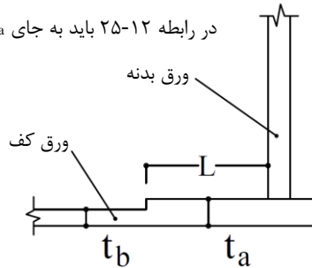
شکل ۱۲-۲ ابعاد ورق‌های بدنه و کف مخزن
