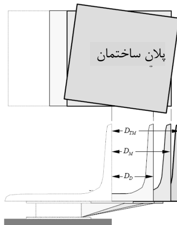
شکل ۹-۱-۹ تعریف جابجایی
