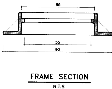
دریچه و قاب چدنی CAST IRON COVER AND FRAME
