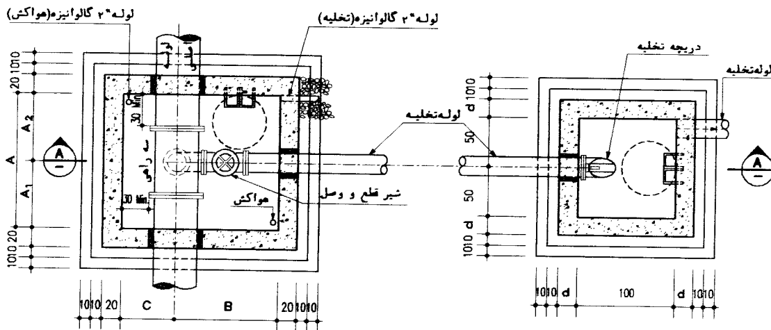
PLAN N.T.S.
