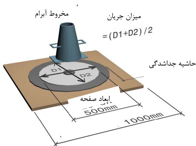
شکل ۳-۱ مشخصات ابزار و وسایل اندازه‌گیری جریان اسلامپ
