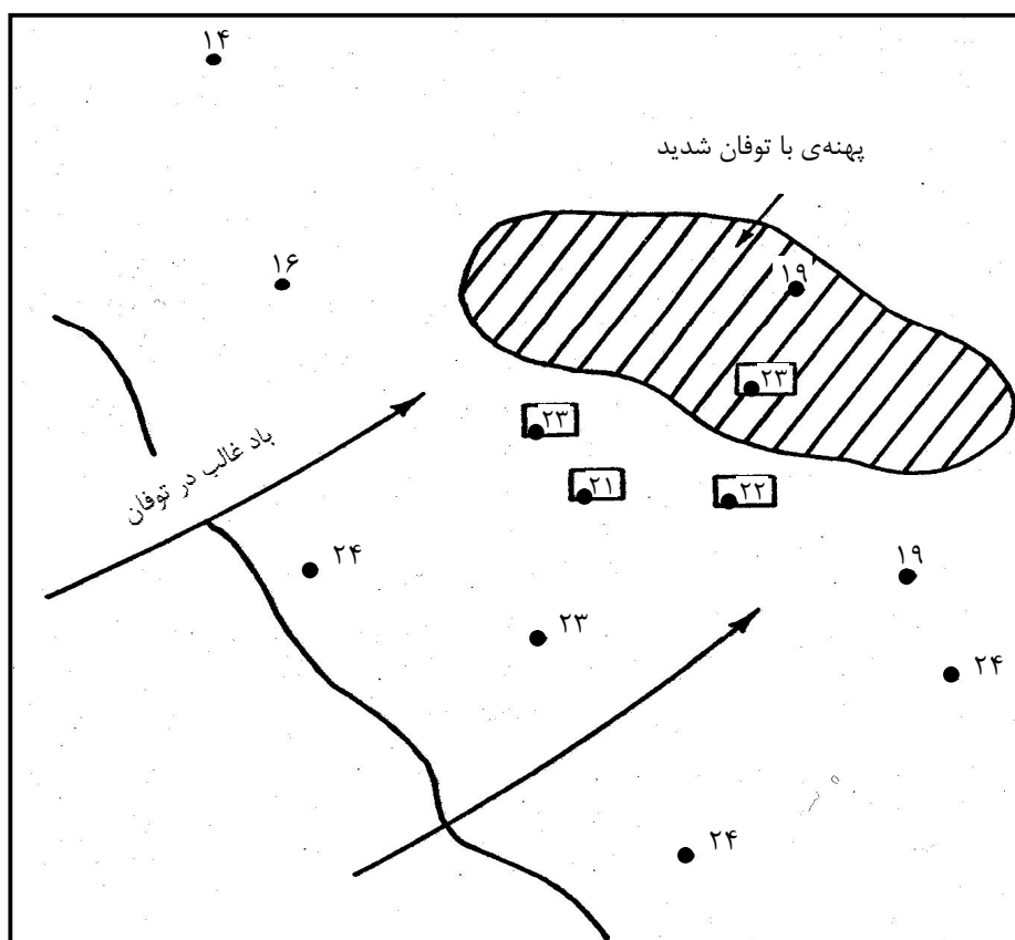
شکل ۴-۲- تعیین نقطه شب‌بم بیشینه در یک توفان، نقطه شب‌بم معرف برای زمان این نقشه برابر با مقادیر میانگین در درون مربع‌ها است.
