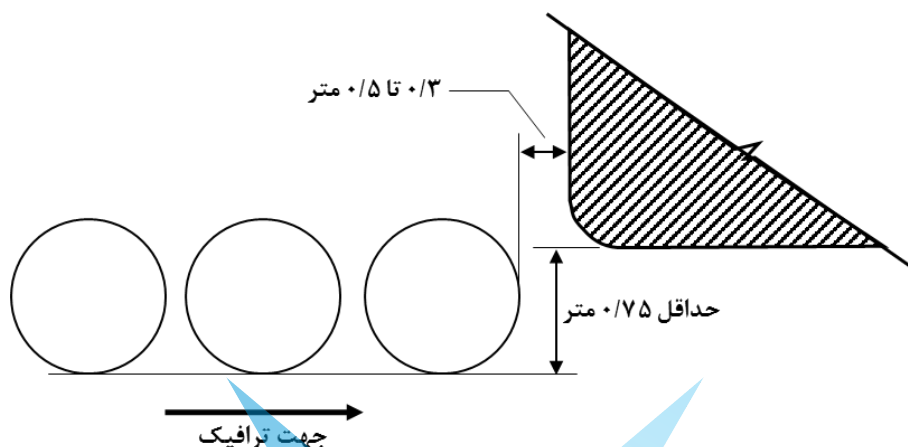
شکل ۶-۱۰- موقعیت سه ردیف آخر بشکه‌های ماسه نسبت به مانع
