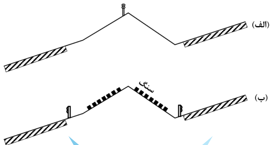
شکل ۵-۱۱- مقطع نوع سه برای میانه‌های شیب‌دار
