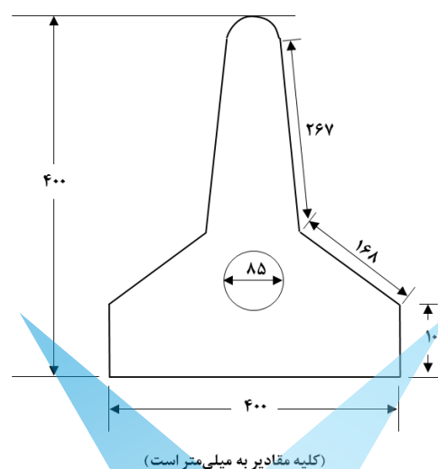
شکل ۷-۹- مشخصات هندسی جداکننده بتنی (مینی نیوجرسی)
