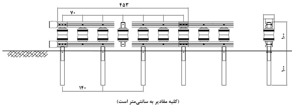
شکل ۳-۲- جزئیات طراحی حفاظ‌های غلتکی
