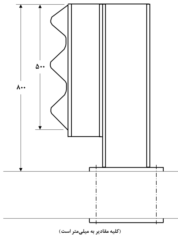
شکل ۳-۱۲- جزئیات طراحی حفاظ سه موجی برای پل
