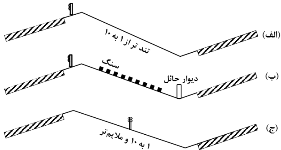
شکل ۵-۱۰- مقطع نوع دو برای میانه‌های شیب‌دار
