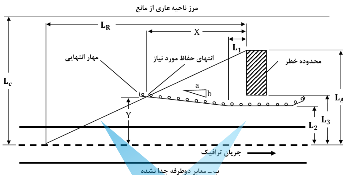
شکل ۵-۱۲- متغیرهای لازم برای تعیین حداقل طول حفاظ
