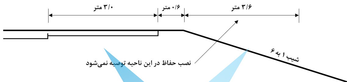
شکل ۵-۲- نمونه‌ای از محدوده نامناسب برای نصب حفاظ در سطح شیب‌دار
