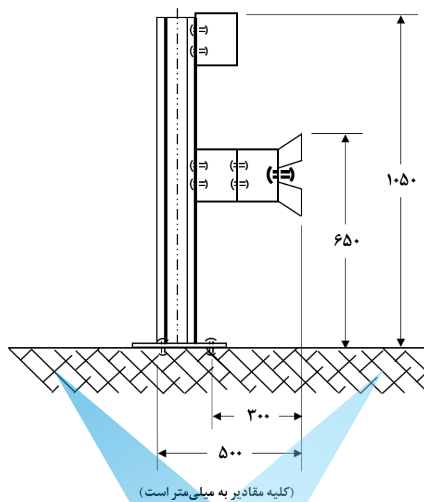
شکل ۳-۱۳- جزئیات طراحی حفاظ سوپر ریل برای پل
