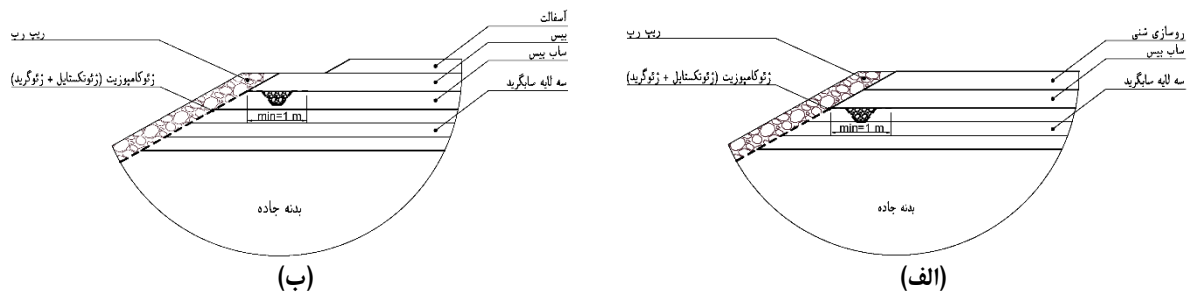
شکل ۴-۱۲ جزئیات اجرای روش ریپرپ در حفاظت جدار در (الف) جاده شنی و (ب) جاده آسفالتی
