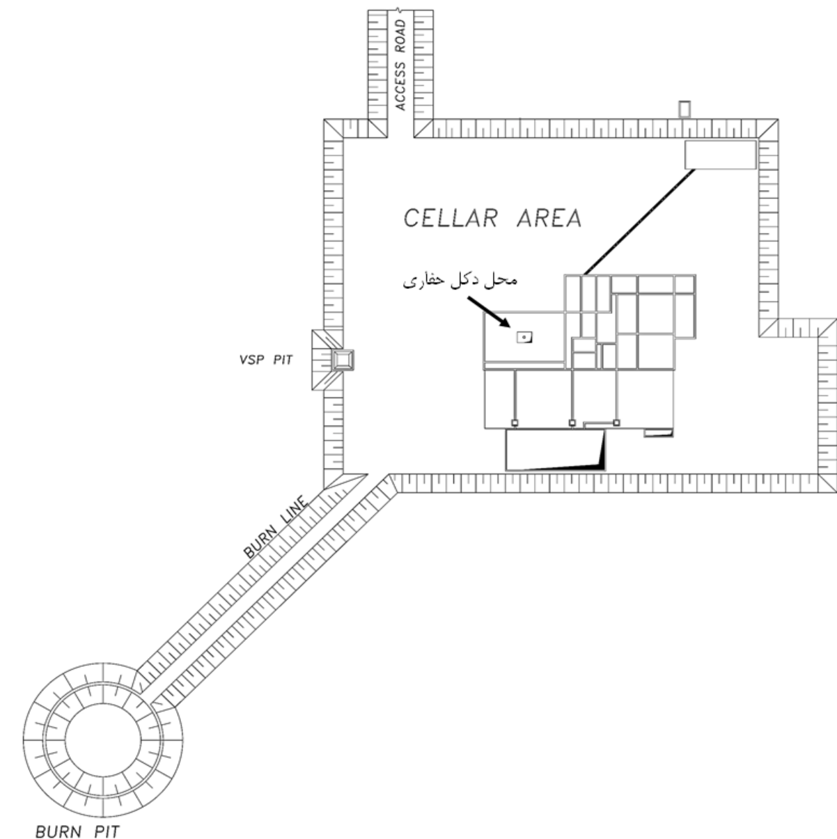
شکل ۱-۵ پلان شماتیک محوطه سر و گودال سوخت
