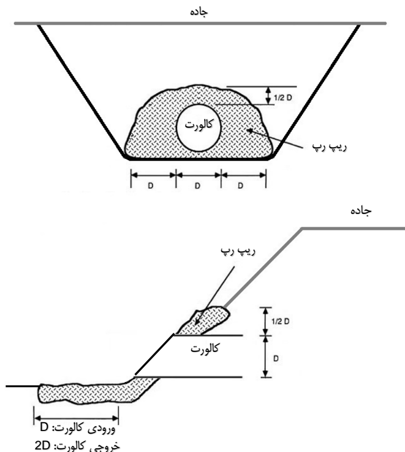
شکل ۴-۱۵ جزئیات حفاظت سطحی اطراف ورودی و خروجی کالورت با استفاده از ریپ‌رپ
