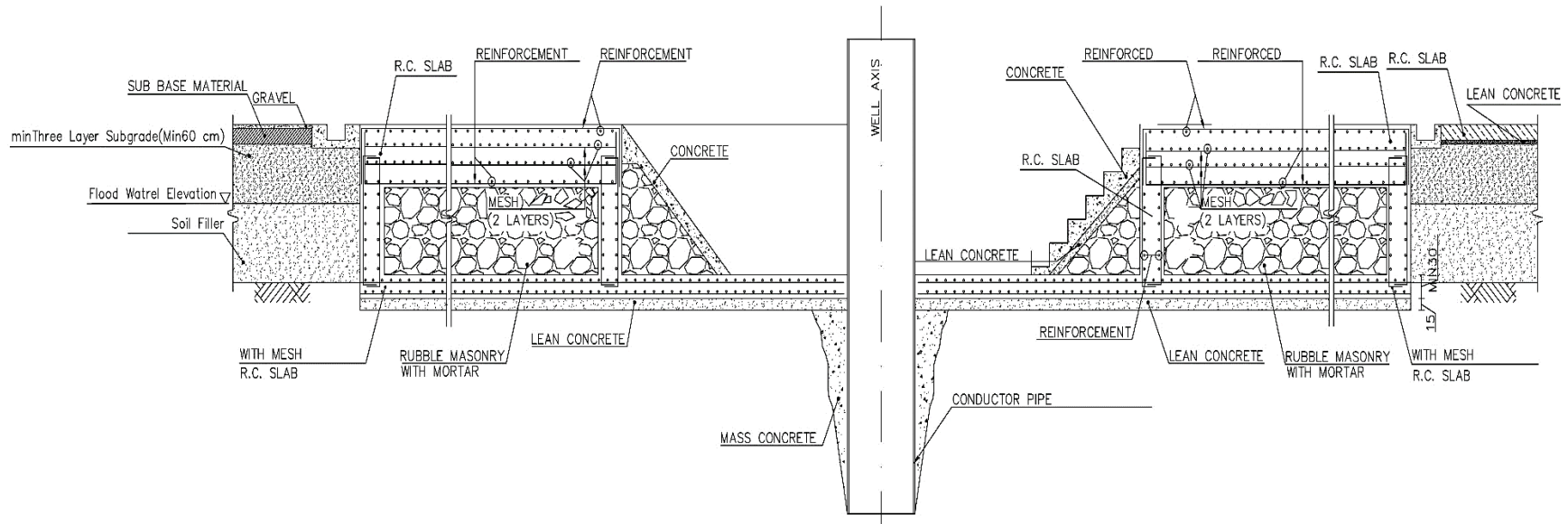
شکل ۵-۵ شکل شماتیک برای اجرای بخش پی گسترده زیر دکل حفاری
