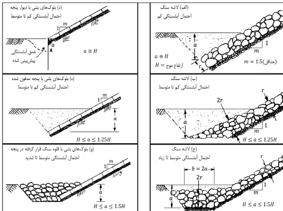
شکل ۴-۱۳ حفاظت از پنجه ریپرپ طبق مرجع (USACE, 1995) EM 1110-2-1614
