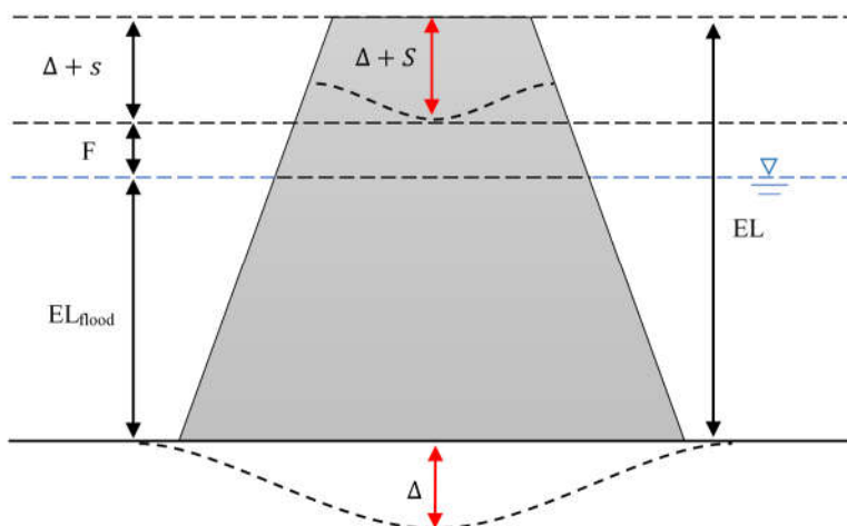
شکل ۴-۸ نشست رخ داده در خاکریز سلرها و جاده‌ها
