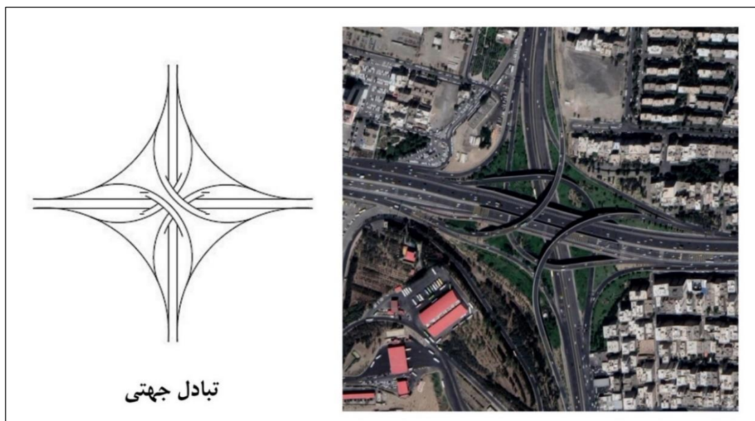
شکل ۵-۵- نمونه ای از یک تبادل جهتی (تهران)
