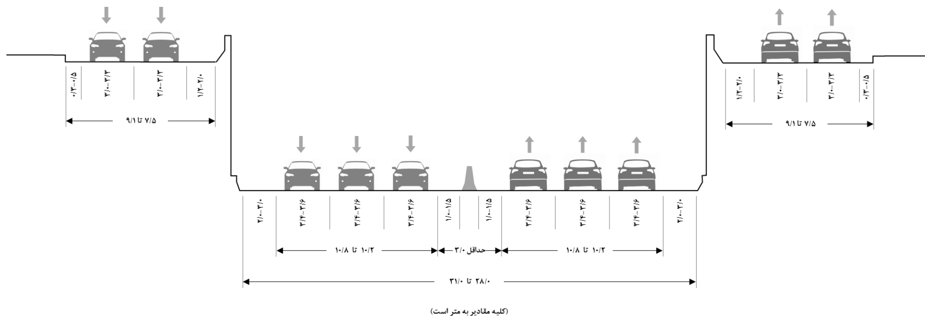
شکل ۳-۱۱- نمونه نیم‌رخ عرضی یک آزادراه پایین‌گذر
