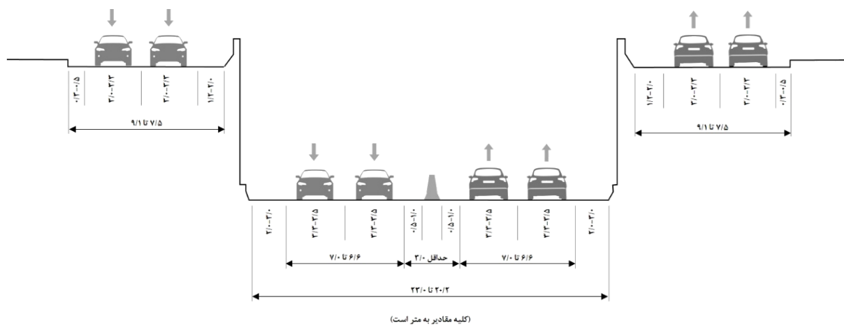
شکل ۸-۴- نمونه نیمرخ عرضی یک بزرگراه شهری پایین‌گذر
