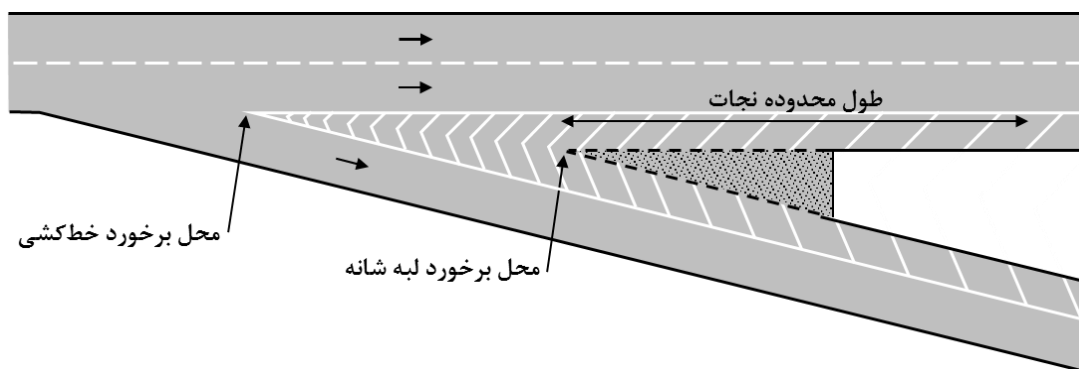
شکل ۵-۶- تعریف محدوده نجات در محل اتصال رابط خروجی
