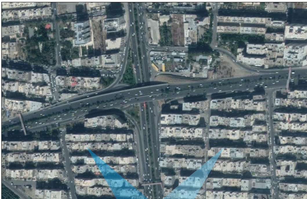
شکل ۵-۸- نمونه تبادل لوزی شکل با حذف تقاطعهای انتهای رابط (تهران)
