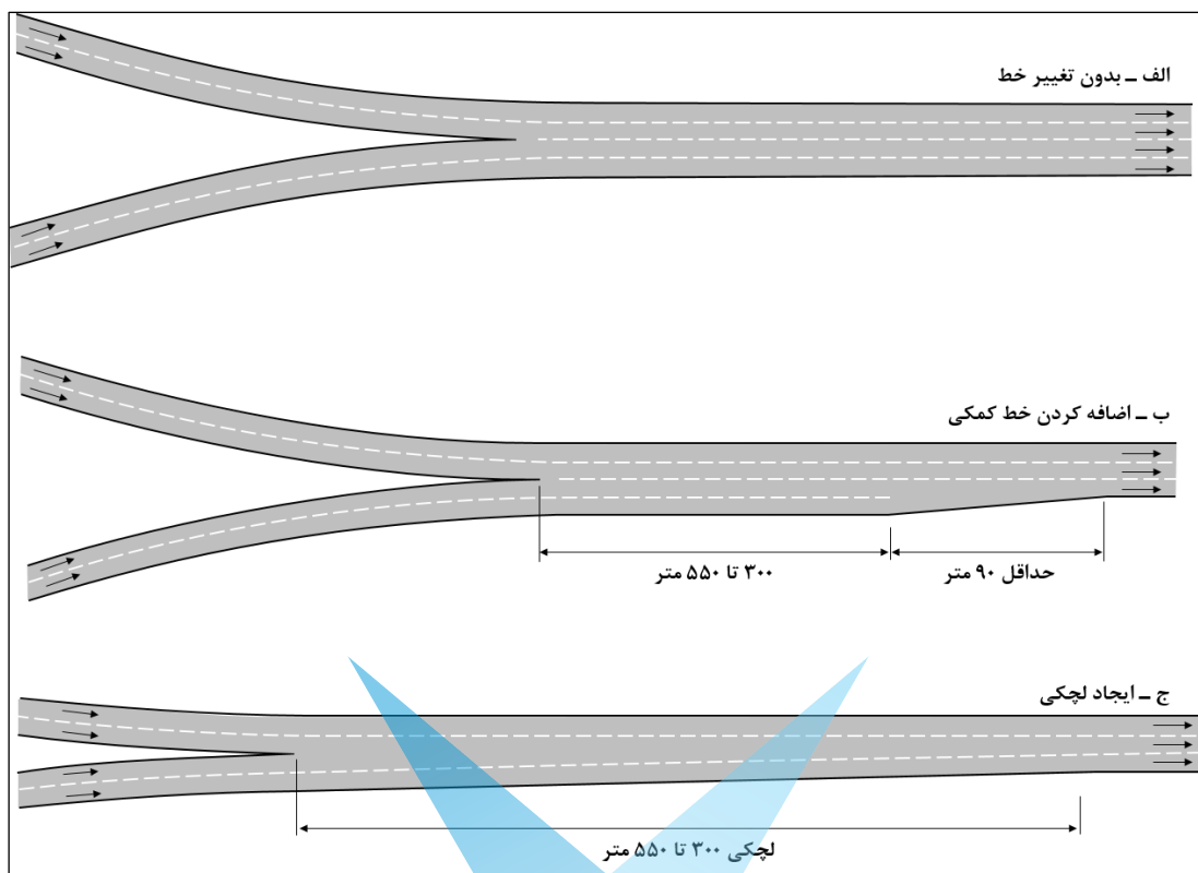
شکل ۷-۹- نمونه حالت‌های اتصال ورودی دو شاخه
