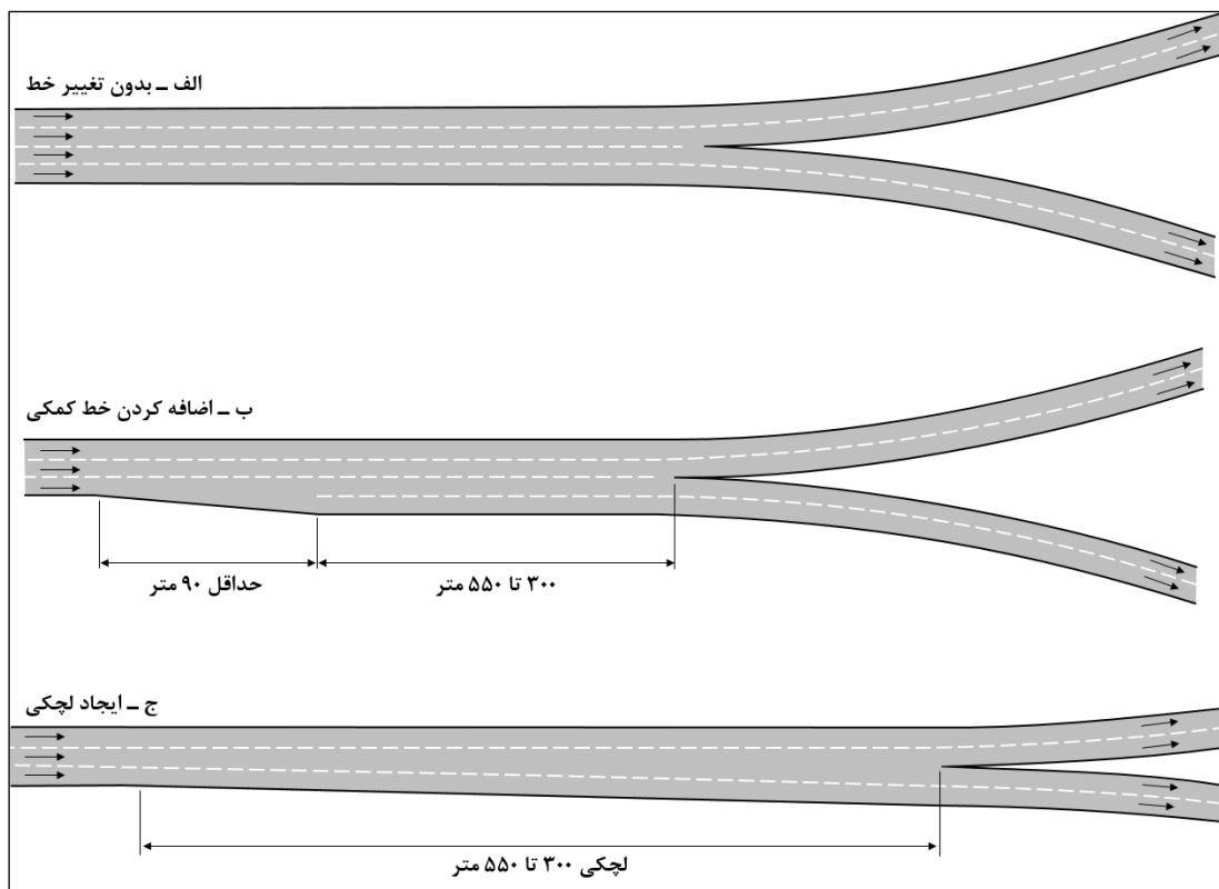
شکل ۷-۸- نمونه حالت‌های اتصال خروجی دو شاخه
