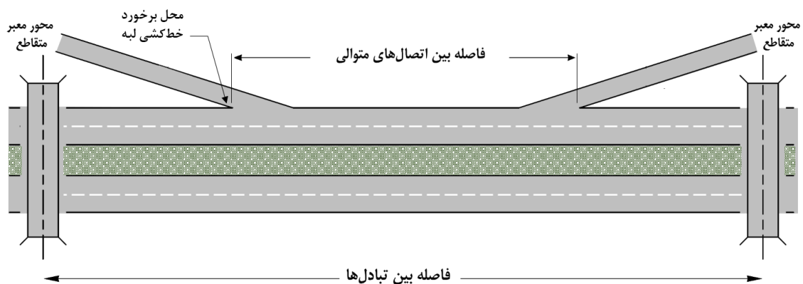
شکل ۳-۲- نحوه تعیین فاصله بین اتصال‌ها و تبادله‌ها در آزادراه‌های شهری
