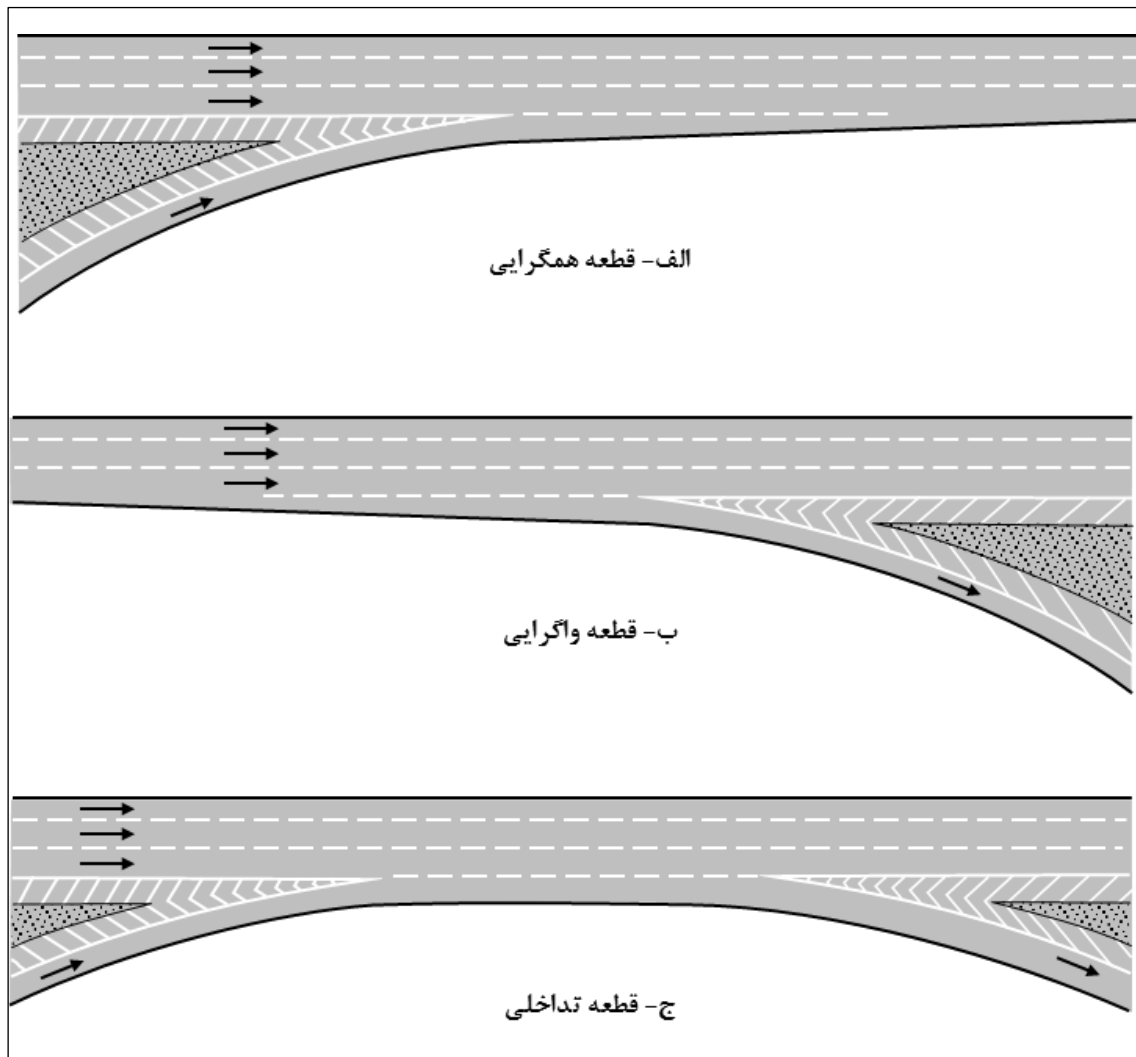
شکل ۹-۱- انواع قطعات تندرایی به منظور تحلیل سطح خدمت
