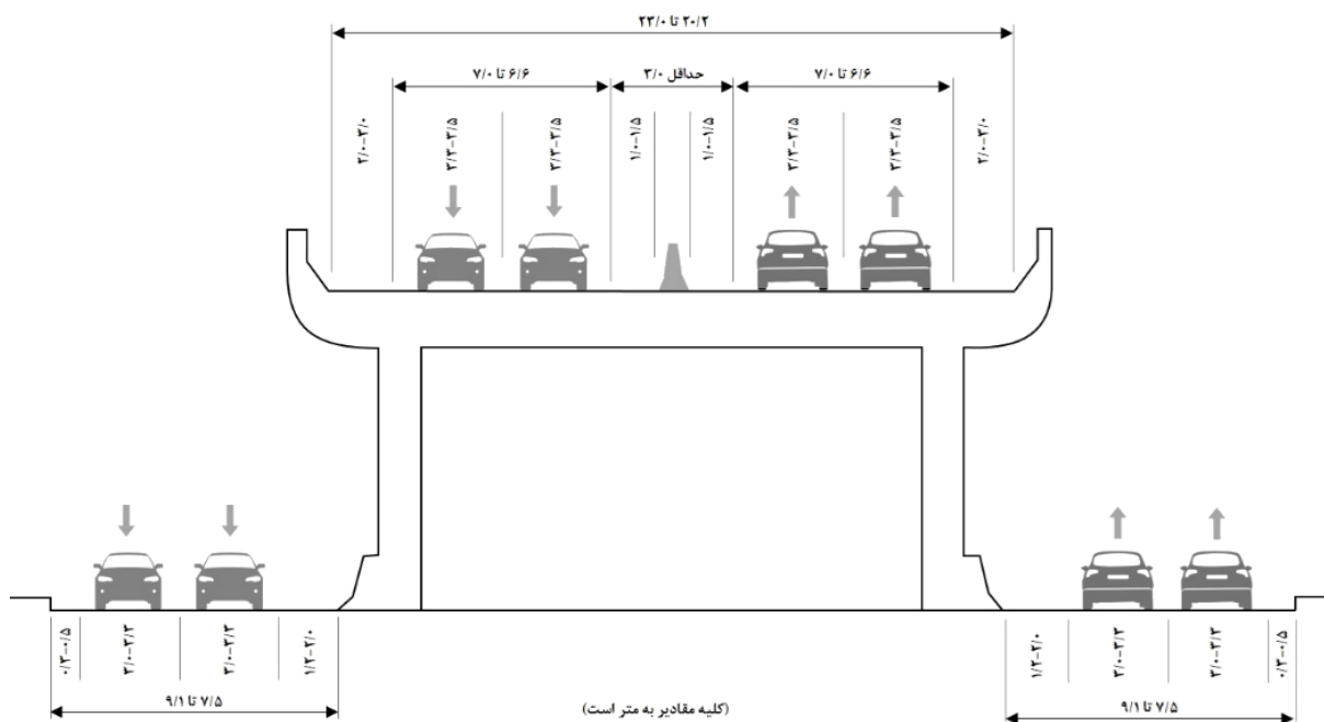
شکل ۹-۴- نمونه نیمرخ عرضی یک بزرگراه شهری بالاگذر
