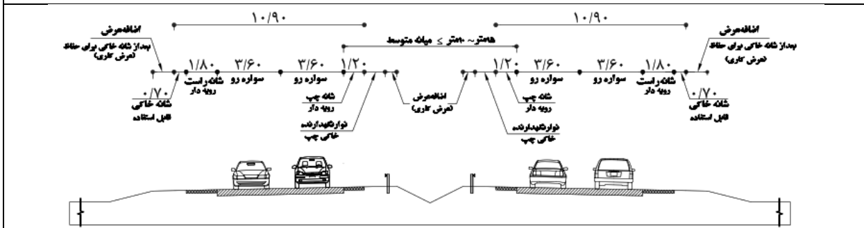
A5- راه شریانی جدادشه چهار خطه با میانه متوسط
