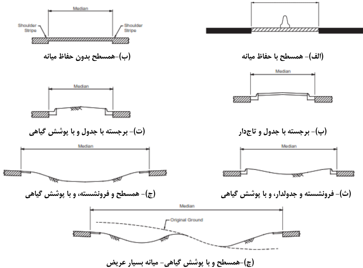
شکل ۶-۸- انواع میانه در راه‌های جداشده
