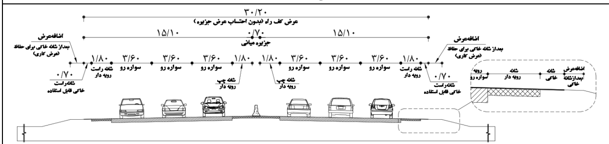
A2- راه شریانی جدادشه شش خطه
