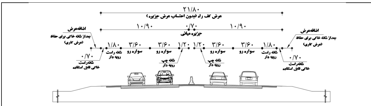
A1- راه شریانی جدادشه چهار خطه
