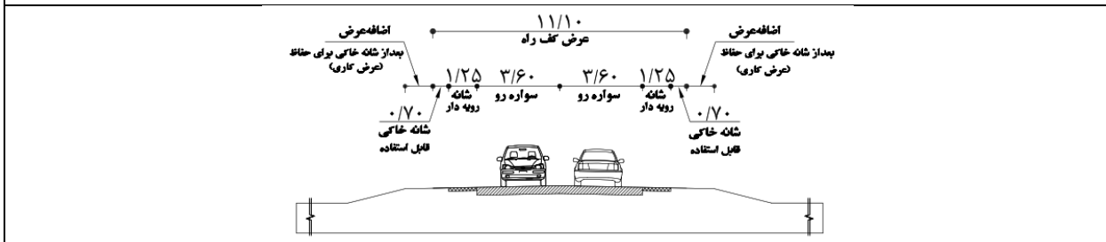
A3- راه شریانی دو خطه با ADT کمتر و برابر ۲۵۰
