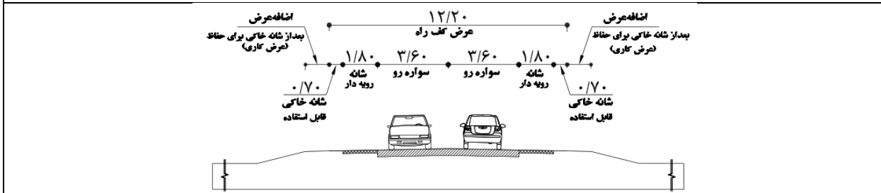
A4- راه شریانی دو خطه با ADT بیشتر از ۲۵۰
