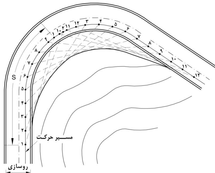
شکل ۶-۵- نحوه تعیین میزان بی‌مانع نمودن محوطه در قوس افقی
