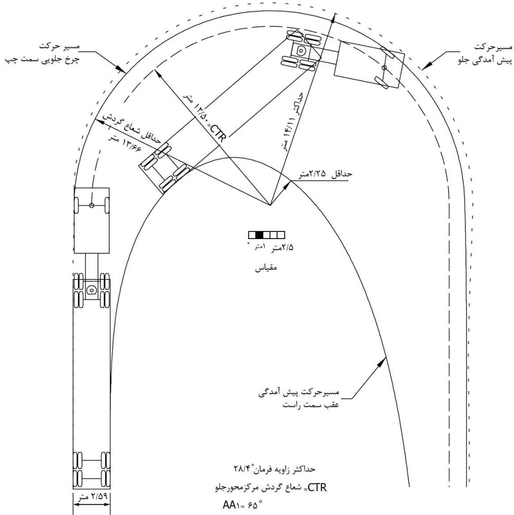
شکل ۴-۸- حد اقل مسیر گردش برای وسیله طرح تریلی نوع ۲
