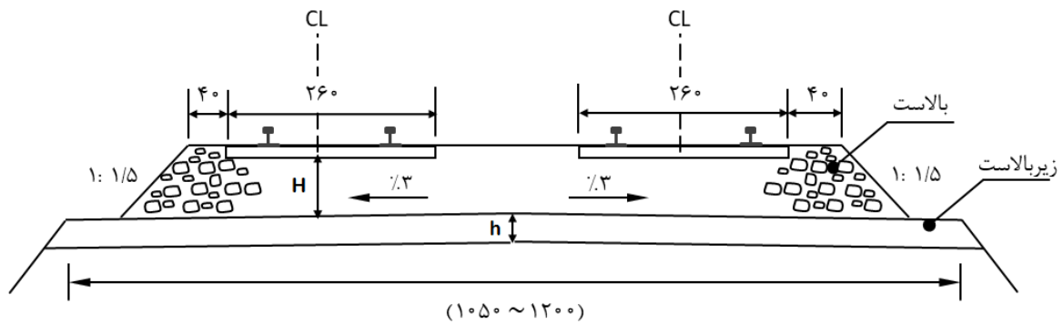
الف: در مسیر مستقیم
