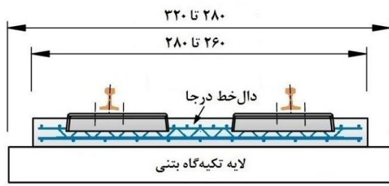
ب: سطح تمام شده بستر
