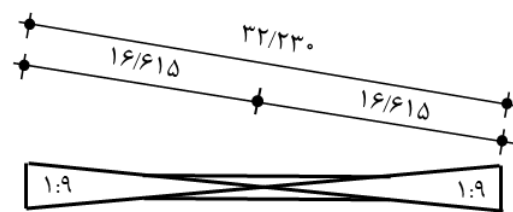
ز: چلیپای مضاعف ۱۹۰ - ۱:۹
