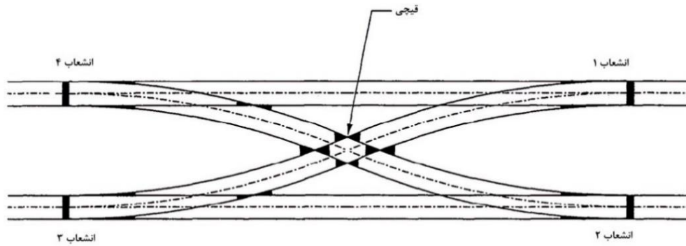
ه: کراس اور دوگانه (قیچی)
