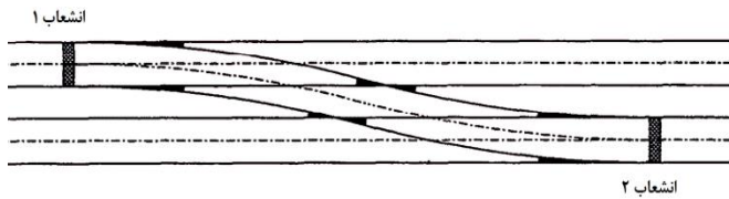
د: کراس اور ساده
