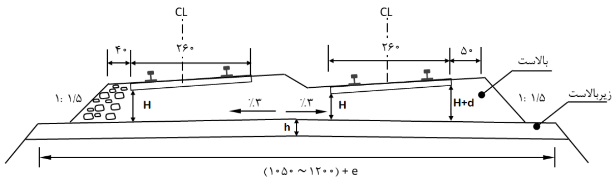
ب: در قوس
