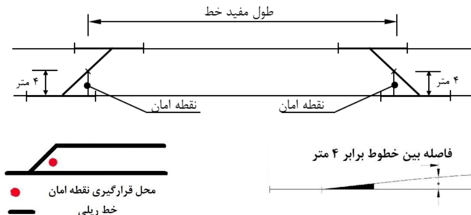
شکل ۵-۱۴ نقطه امان و طول مفید خطوط
