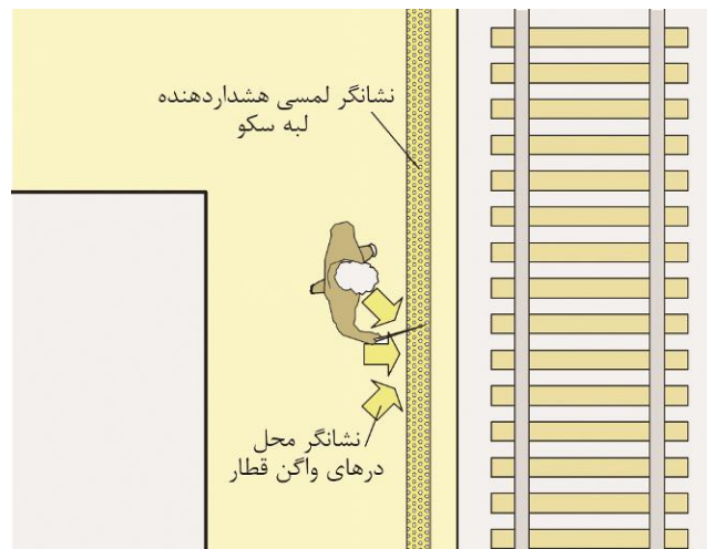
شکل ۲-۱۲۶: علائم هشداردهنده لبه سکو مترو
