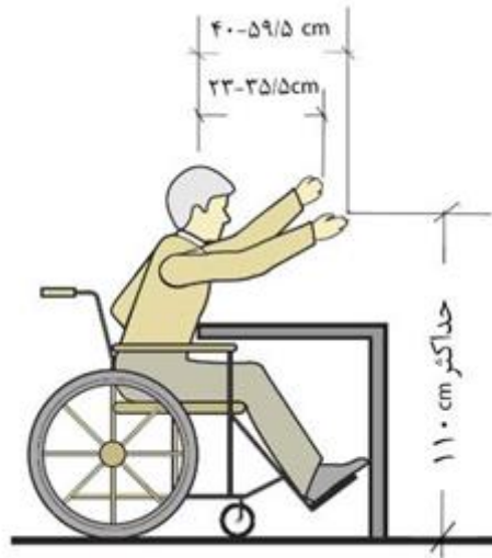
شکل ۱-۱۲: دسترسی مرد دارای معلولیت در حرکت به جلو و بالا با مانع
