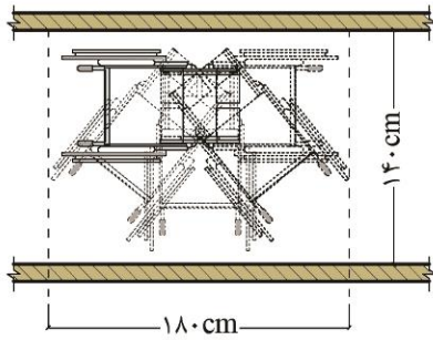
شکل ۱۷-۱: سطح مورد نیاز برای گردش ۱۸۰ درجه‌ای صندلی چرخدار
