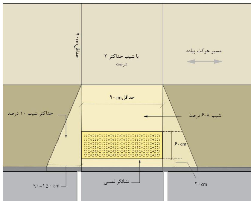
شکل ۲-۵۴: مشخصات رمپ جدول (پلان)
