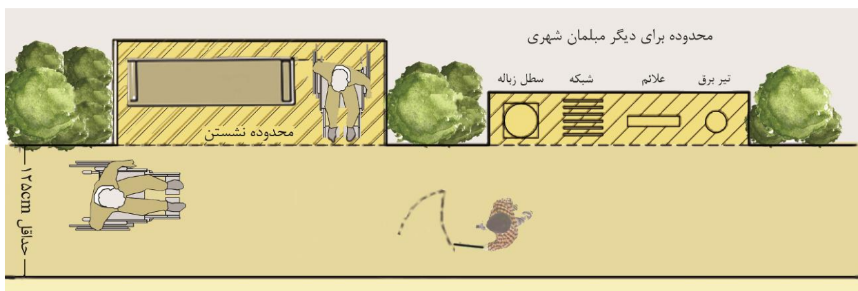
شکل ۲-۱۳۳: قرارگیری محل استراحت خارج از محدوده پیاده‌روی
