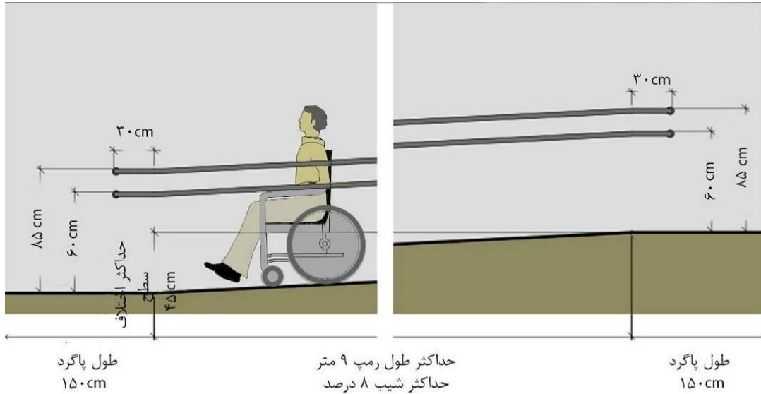
شکل ۸۱-۲: سطح شیب‌دار در فضای خارجی
