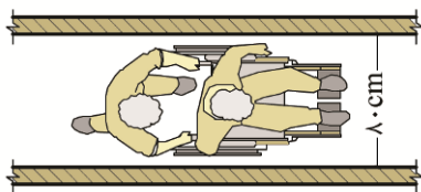
شکل ۲۱-۱: فضای مورد نیاز برای حرکت مستقیم صندلی چرخدار با همراه
