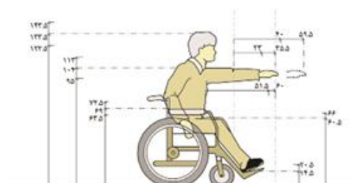
شکل ۱-۵: اندازه‌ها و دسترسی‌های مرد دارای معلولیت در حرکت به جلو
