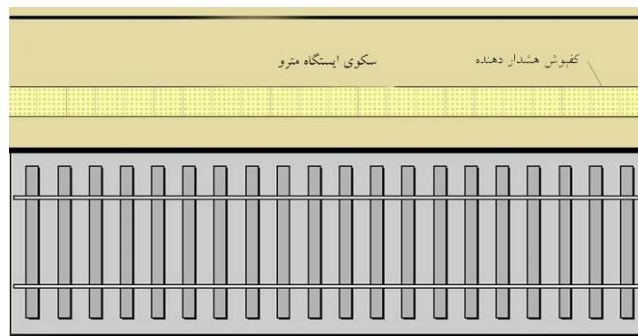
شکل ۲-۱۲۷: علائم هشداردهنده لبه سکو مترو
