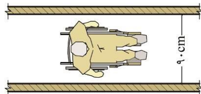
شکل ۲۰-۱: فضای مورد نیاز برای حرکت مستقیم صندلی چرخدار بدون همراه
