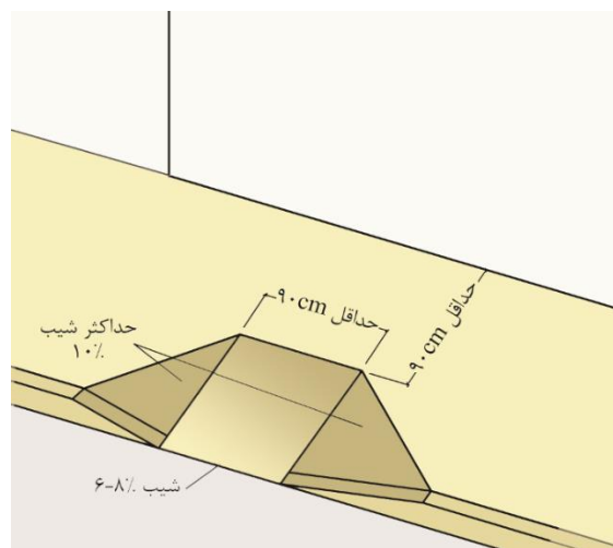
شکل ۲-۵۰: رمپ‌جدول
