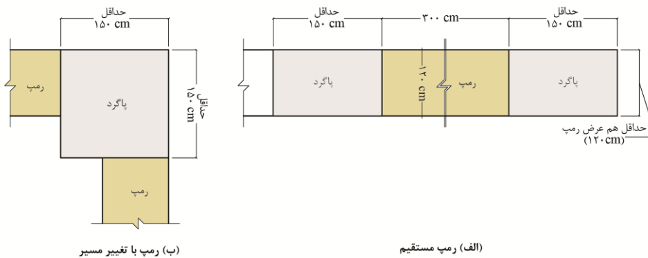
شکل ۸۲-۲: ابعاد رَمپ و پاگرد
