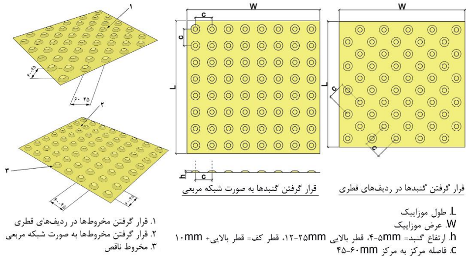
شکل ۲-۲۷: چیدمان، فواصل و ابعاد کفیوش سکه‌ای
