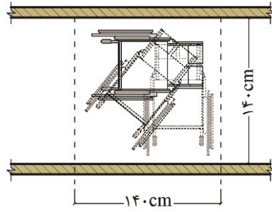
شکل ۱۶-۱: سطح مورد نیاز برای گردش ۹۰ درجه‌ای صندلی چرخدار
