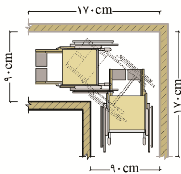
شکل ۱۹-۱: سطح مورد نیاز برای چرخش صندلی چرخدار از زاویه ۹۰ درجه
