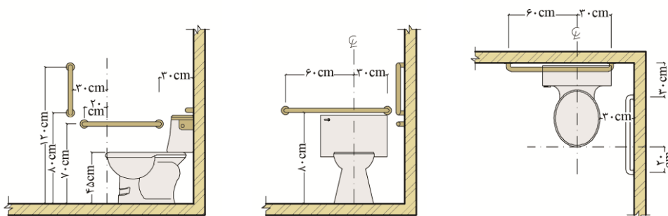
شکل ۲-۱۶۲: ابعاد سرویس بهداشتی فرنگی و میله دستگرد بر دیوار پشت و مجاور آن
