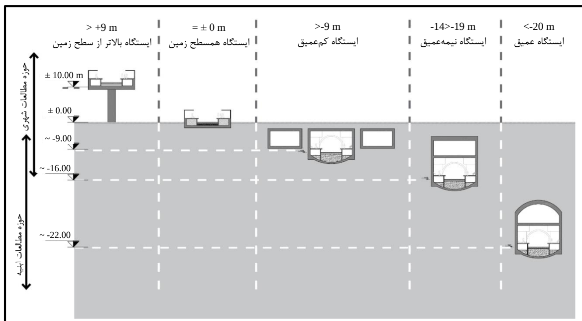
شکل ۴-۱- دیگرام سطح مداخله مطالعات شهری و ابنیه در تعیین پروفیل مسیر و ایستگاه‌ها
