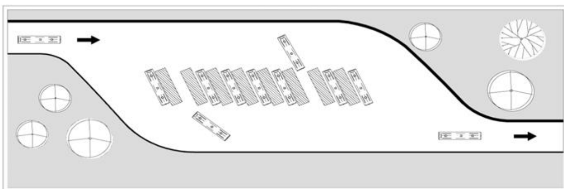
شکل ۸-۳- نمونه چیدمان میان گذر سکوها پایانه
