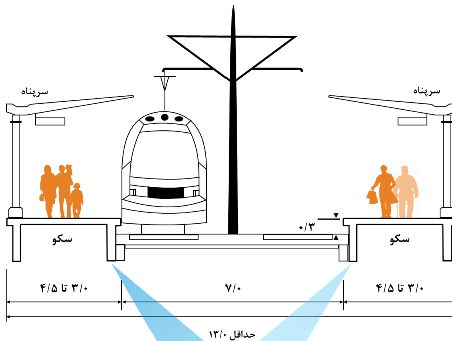
شکل ۱۰-۶- نیمرخ عرضی ایستگاه‌های قطار شهری با سکوهای کناری
