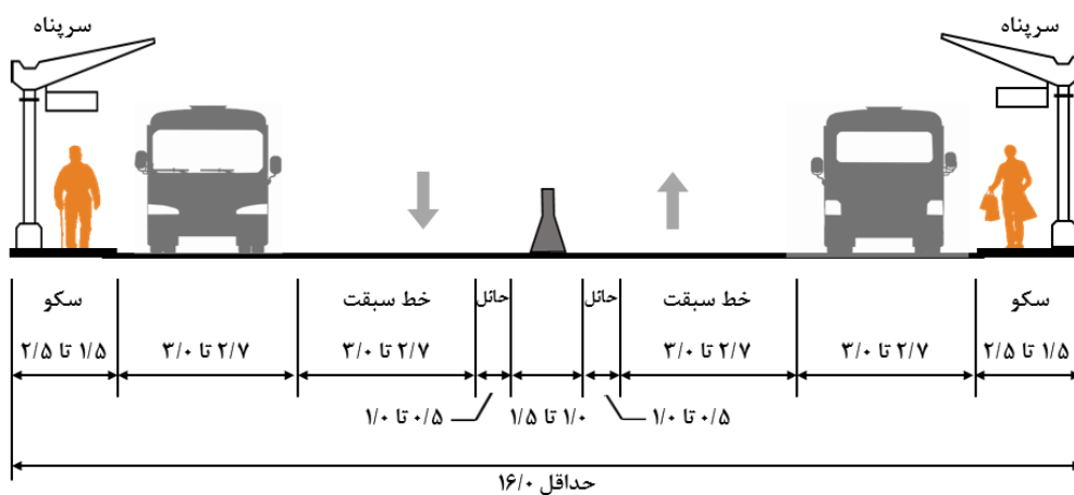
شکل ۴-۶- نیمرخ عرضی ایستگاه‌های مینی‌بوس دارای قابلیت سبقت واقع در میانه با سکوه‌های کناری
