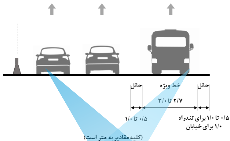
شکل ۴-۴- مشخصات هندسی خط ویژه مینی‌بوس جدا شده با خط‌کشی در سمت راست معبر
