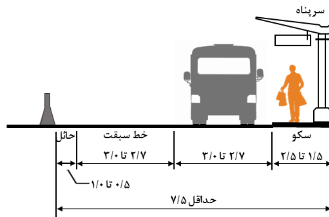
شکل ۶-۲- مقطع عرضی یک ایستگاه مینی‌بوس واقع در سمت راست خط ویژه کناری
