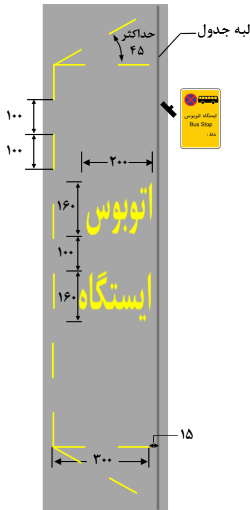
شکل ۷-۸- الگوی خط کشی مناسب در ایستگاه های کناری اتوبوس
