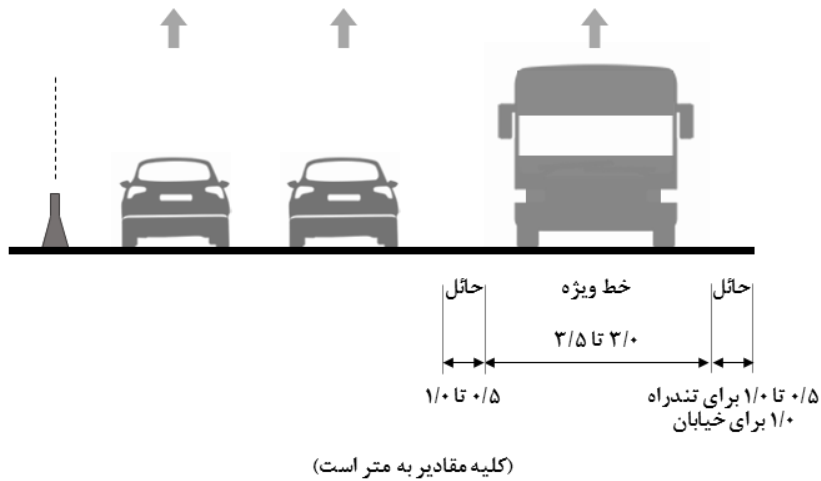
شکل ۳-۴- مشخصات هندسی خط ویژه اتوبوس جدا شده با خط‌کشی در سمت راست معبر
