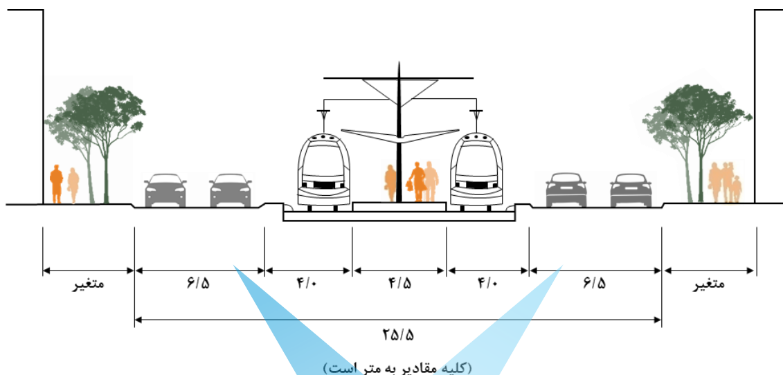
شکل ۱۰-۴- نمونه نیم‌رخ عرضی خیابان شریانی دوطرفه دارای قطار شهری با ایستگاه‌های میانی
