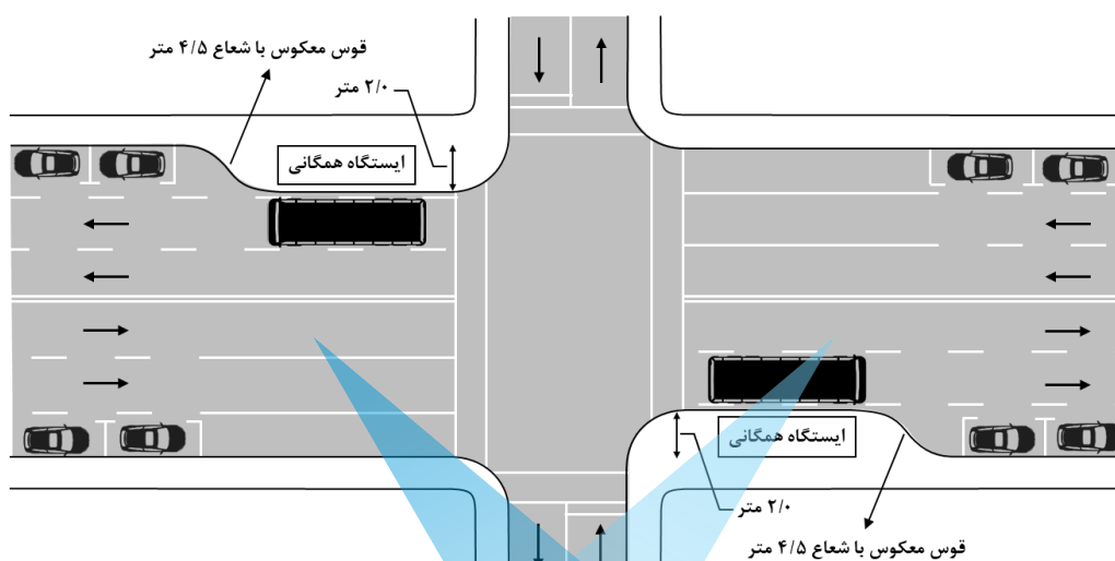
شکل ۴-۵- ایستگاه پیش‌آمده بعد از تقاطع
