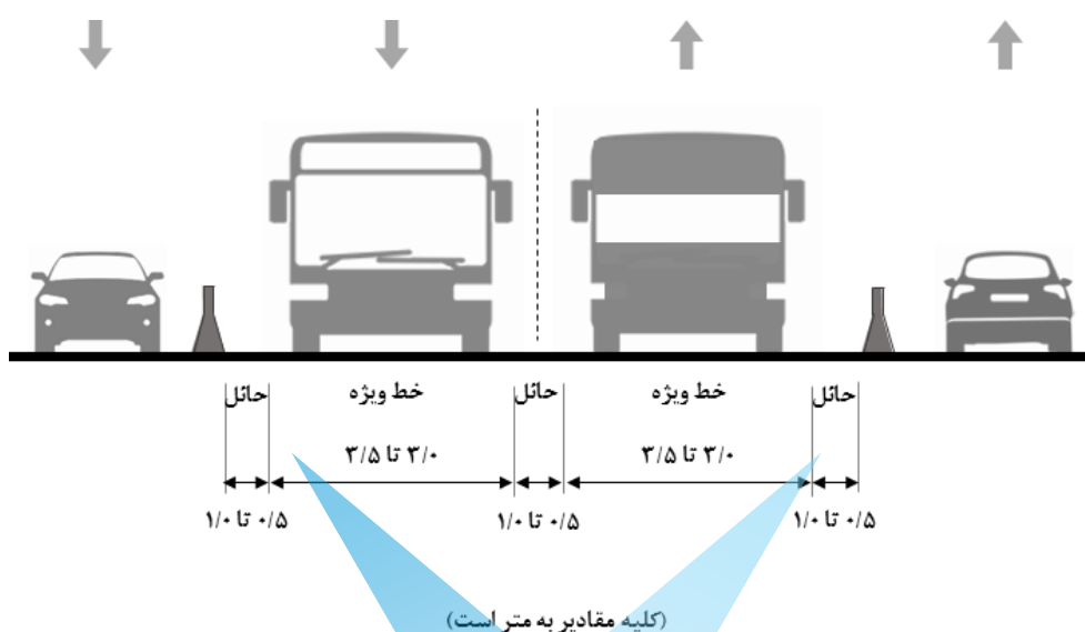
شکل ۴-۵- مشخصات هندسی خط ویژه اتوبوس جدا شده با مانع فیزیکی در میانه معبر
