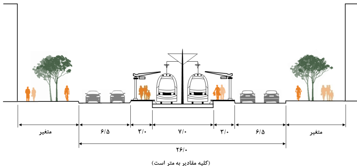
شکل ۹-۴- نمونه نیم‌رخ عرضی خیابان شریانی دوطرفه دارای قطار شهری با ایستگاه‌های کناری
