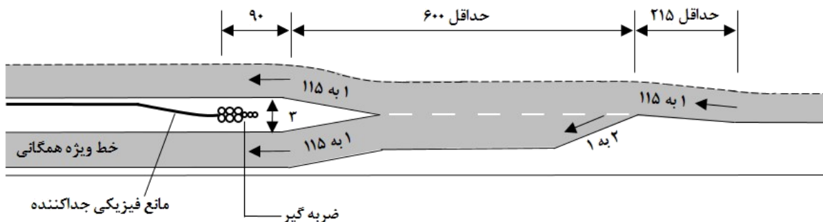
شکل ۷-۵- مشخصات هندسی ابتدای خط ویژه میانی جدا شده با موانع فیزیکی
