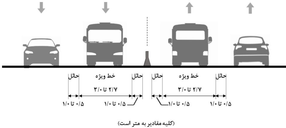
شکل ۲-۴- مشخصات هندسی خط ویژه مینی‌بوس جدا شده با خط‌کشی در میانه معبر
