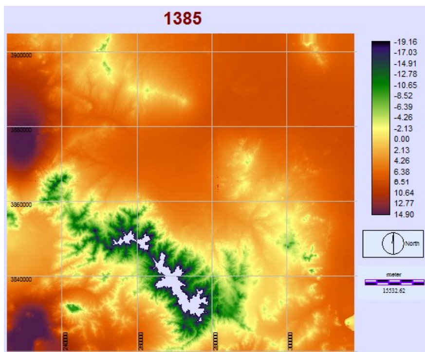
شکل پ.۱-۱۱- د- نقشه هم دمای حوزه در سال ۱۳۸۵ (دنباله)
