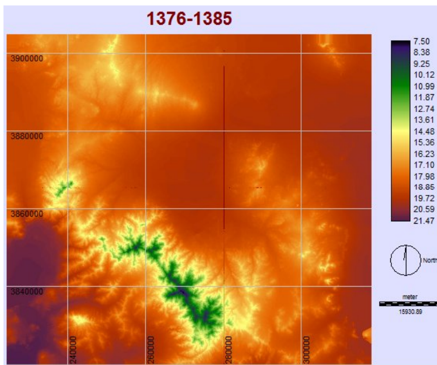
شکل پ.۱-۱۱-الف- نقشه هم دمای حوضه در سال‌های ۱۳۸۵-۱۳۷۶
