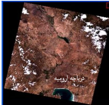
شکل ۵-۲۵- تصویر طبیعی سنجنده ETM+ ماهواره Landsat بخشی از منطقه دریاچه ارومیه، آذربایجان شرقی، آذربایجان غربی و دریاچه سد ارس
