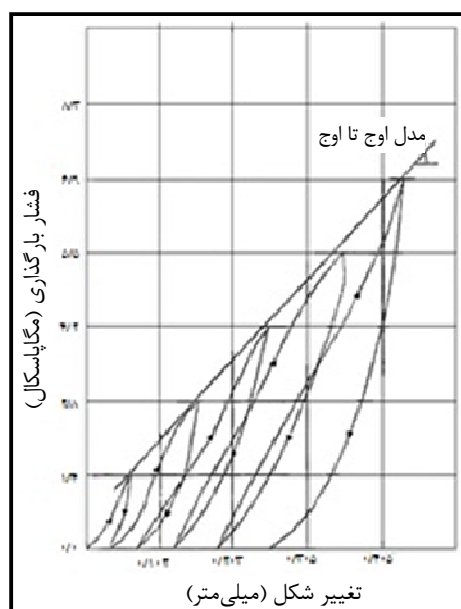
شکل ۹-۳- تغییر شکل سطح سنگ به صورت تابعی از فشار بارگذاری
