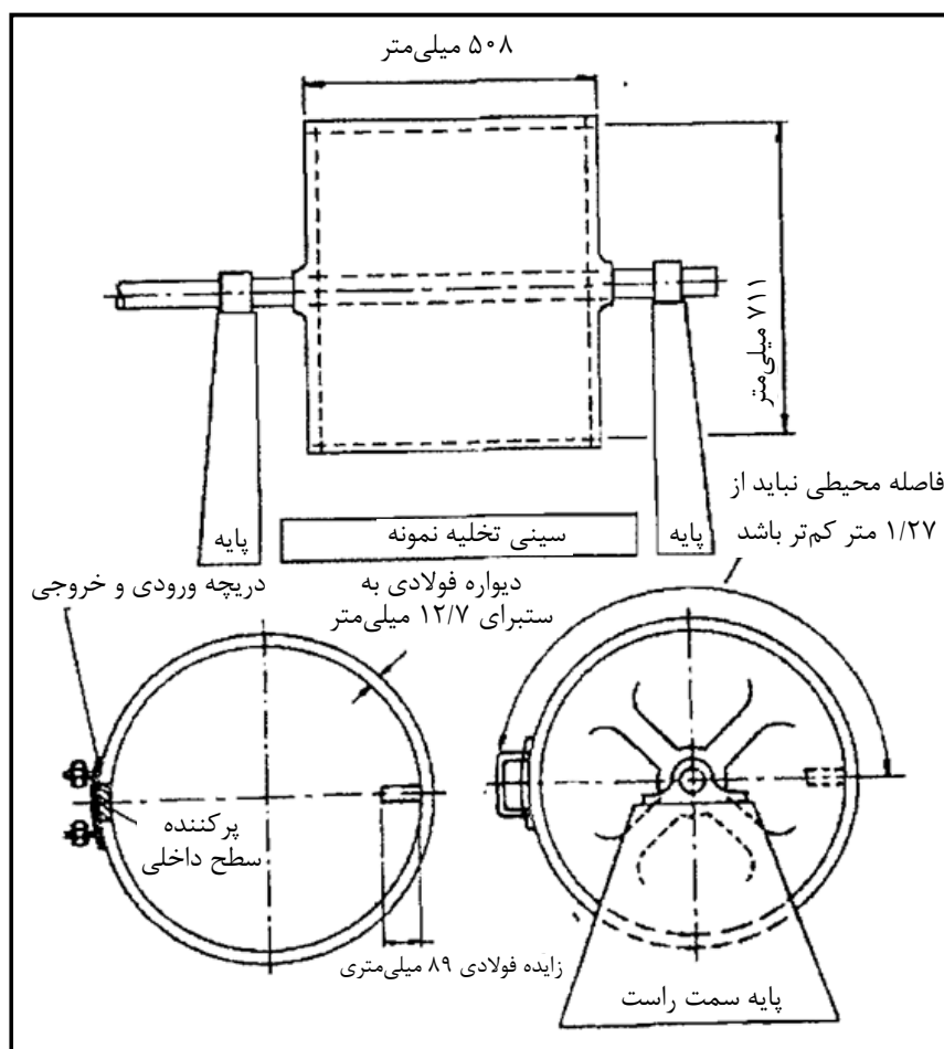
شکل ۱-۳- نمایش شماتیک دستگاه لس آنجلس
