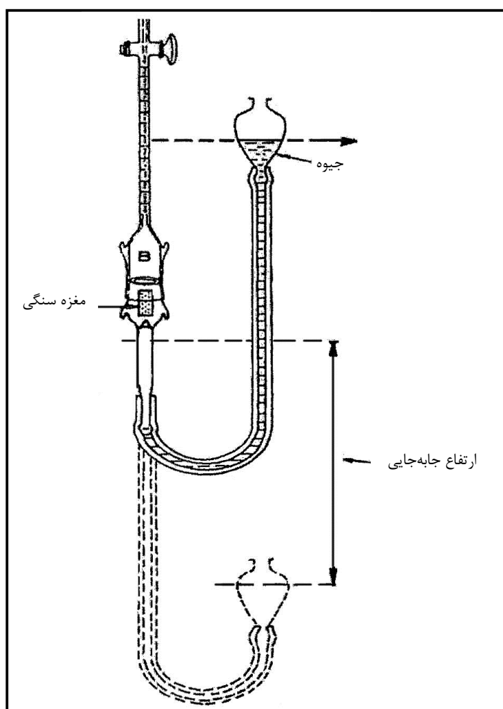
شکل ۱-۱- دستگاه تخلخل‌سنج با روش جابه‌جایی جیوه، انواع واشبرن - بونتینگ ۱
