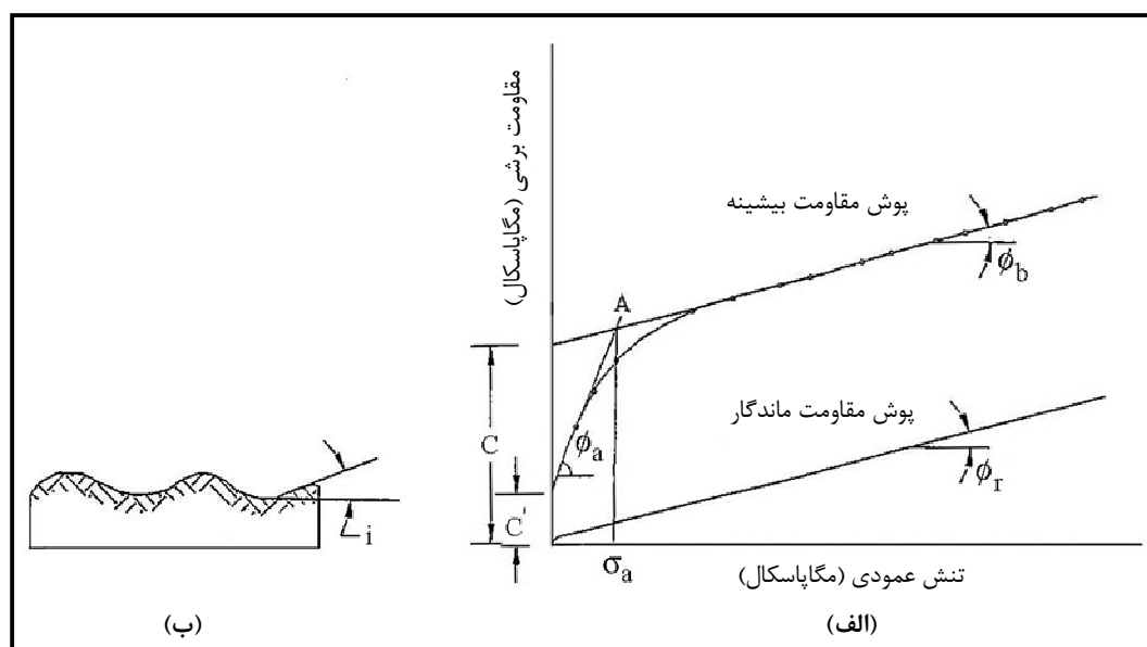
شکل ۳-۲۵- پوش گسیختگی نهایی و ماندگار در آزمایش برجا
