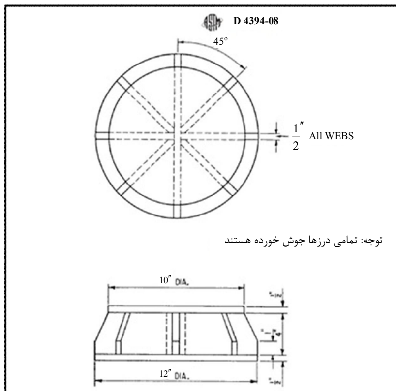
شکل ۳-۷- صفحات بارگذاری صلب با قطر ۱۲ اینچ
