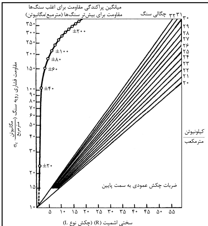
شکل ۲-۱۳- نمودار وابستگی مقاومت فشاری سنگ به عنوان تابعی از شمار سختی و اجتهشی اشمیت و چگالی خشک
