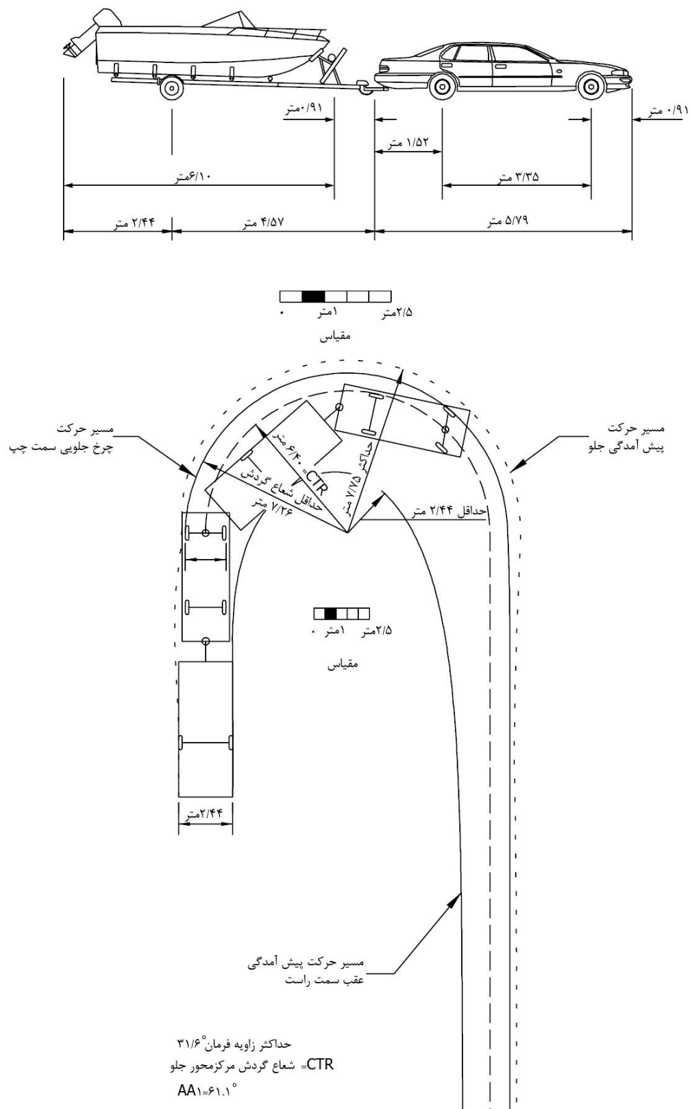
شکل ۴-۱۰- حداقل مسیر گردشی برای وسیله طرح سواری با یدک قایق
