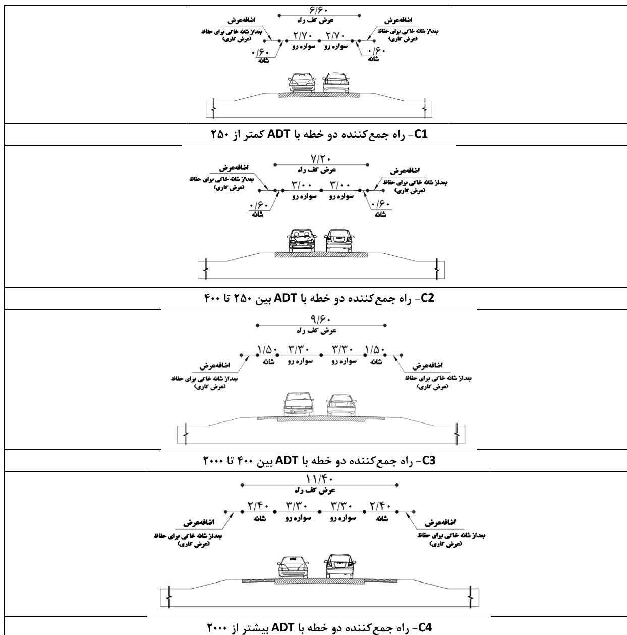
شکل ۶-۳۲ - مقاطع عرضی نمونه برای راه‌های جمع کننده
