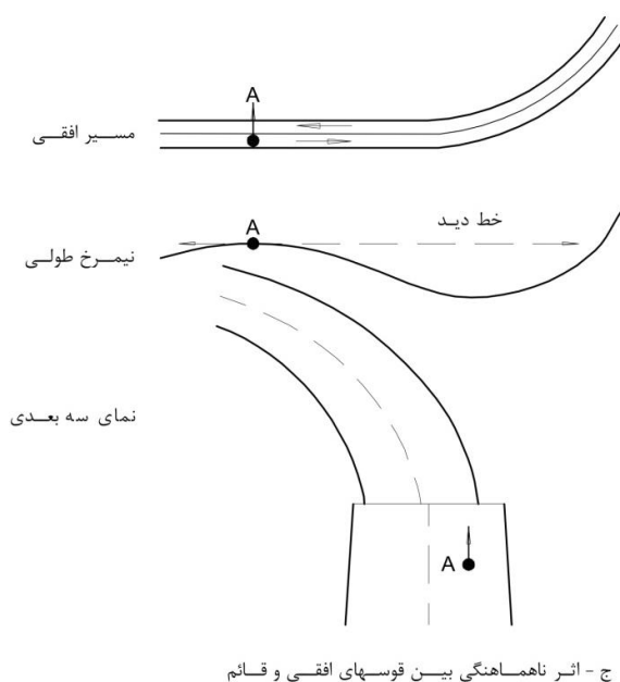
شکل ۵-۲۵- نمونه‌هایی از نحوه هماهنگی پلان و پروفیل طولی راه
