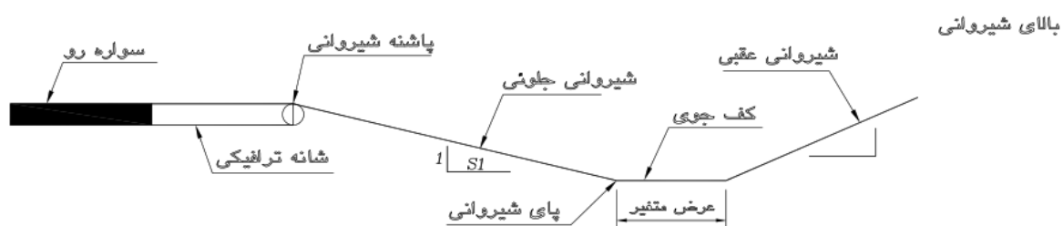
شکل ۶-۷- تقسیم‌بندی نواحی کناره راه
