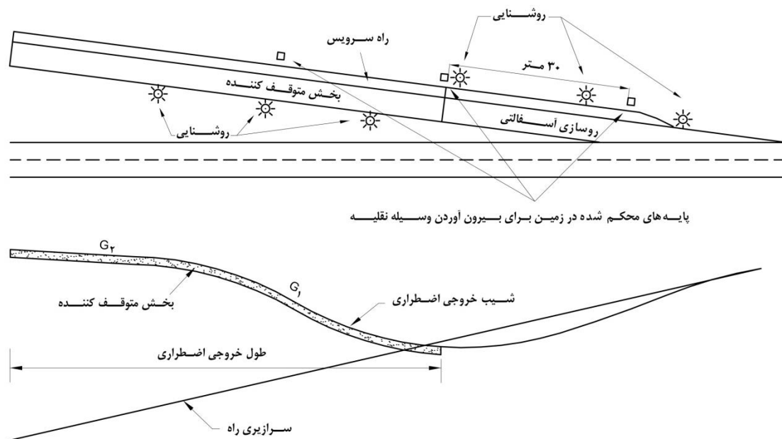
شکل ۵-۲۰- نمونه رمپ فرار اضطراری
