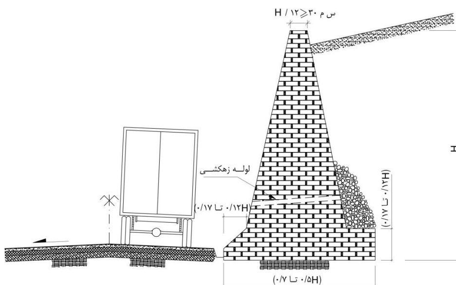
شکل ۶-۲۱- دیوار حائل وزنی
