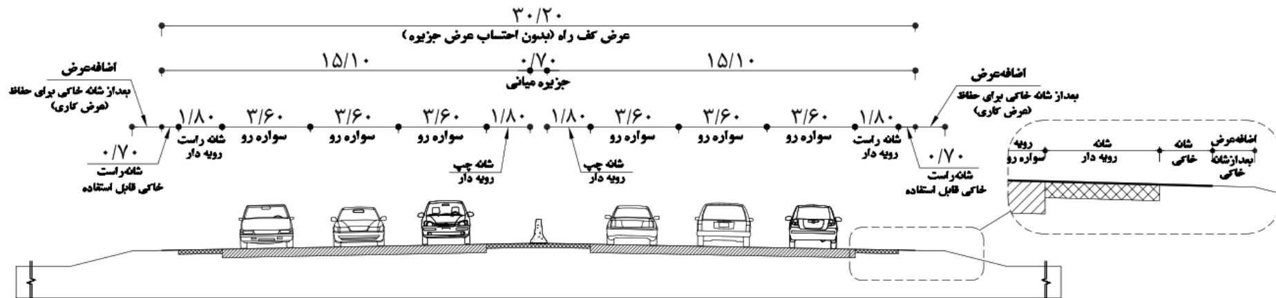
A2- راه شریانی جداشده شش خطه
