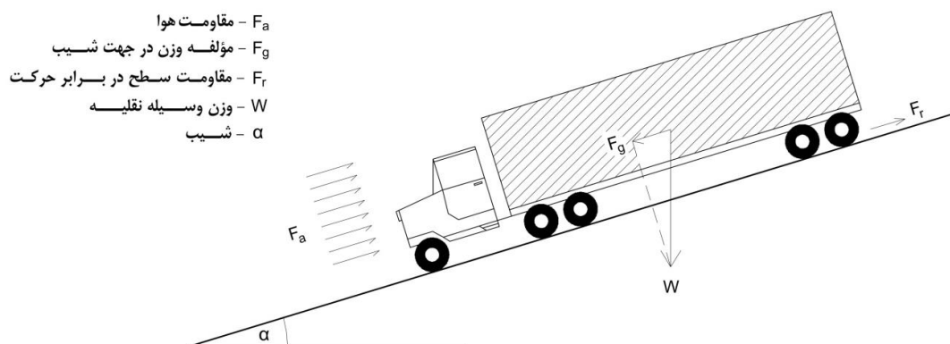
شکل ۵-۱۸- نیروهای وارده بر وسیله در حال حرکت در سرازیری
