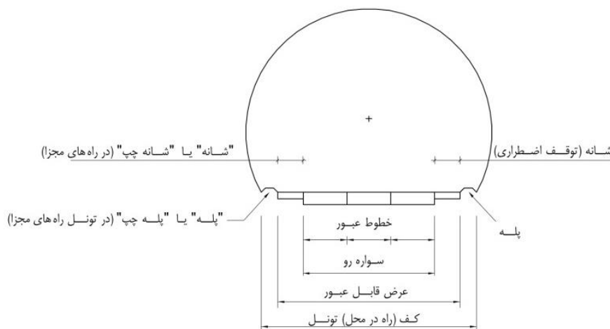
شکل ۶-۲۷- اجزاء مقطع عرضی تونل
