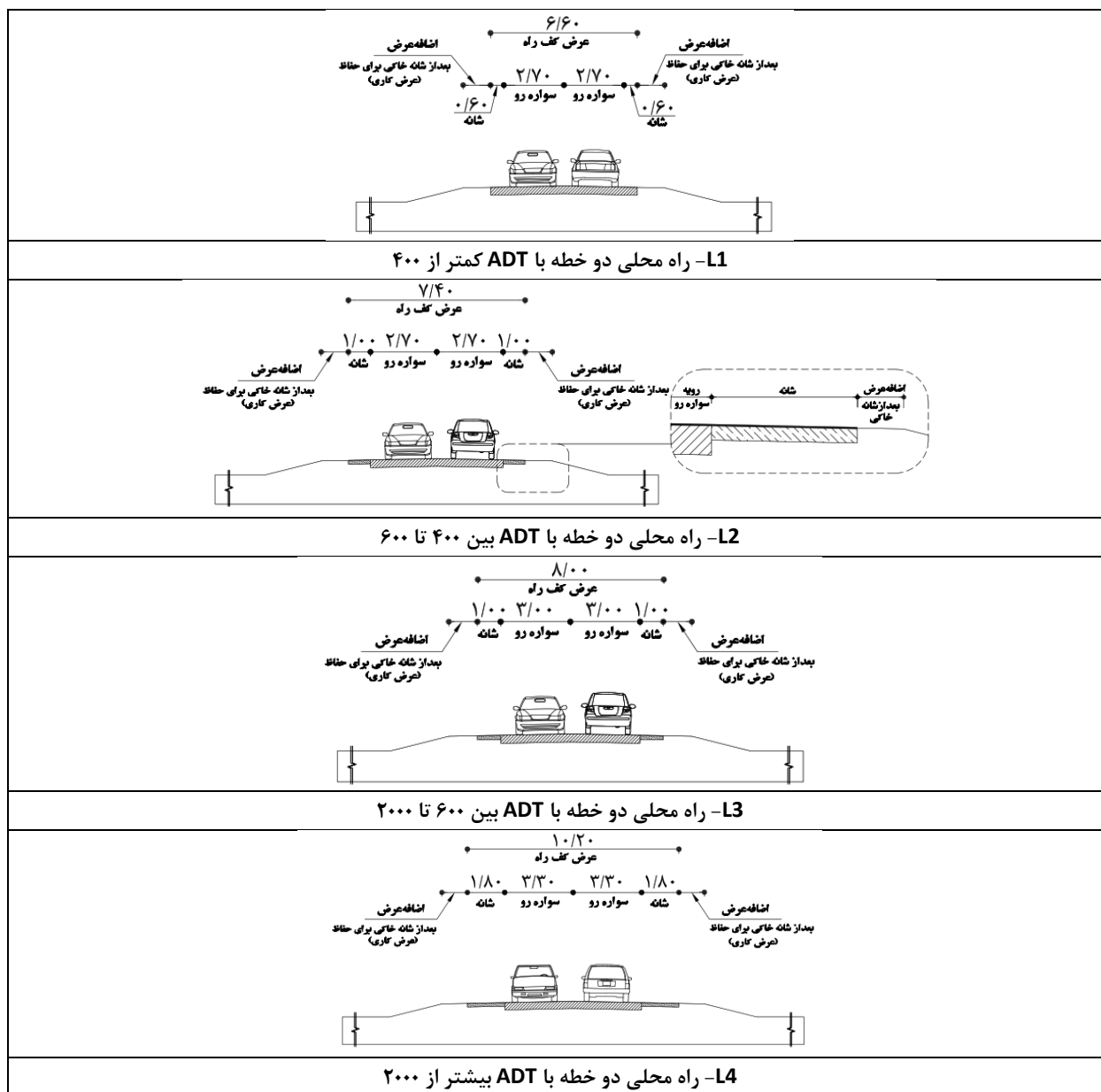
شکل ۶-۳۳- مقاطع عرضی نمونه برای راه‌های محلی - روستایی
