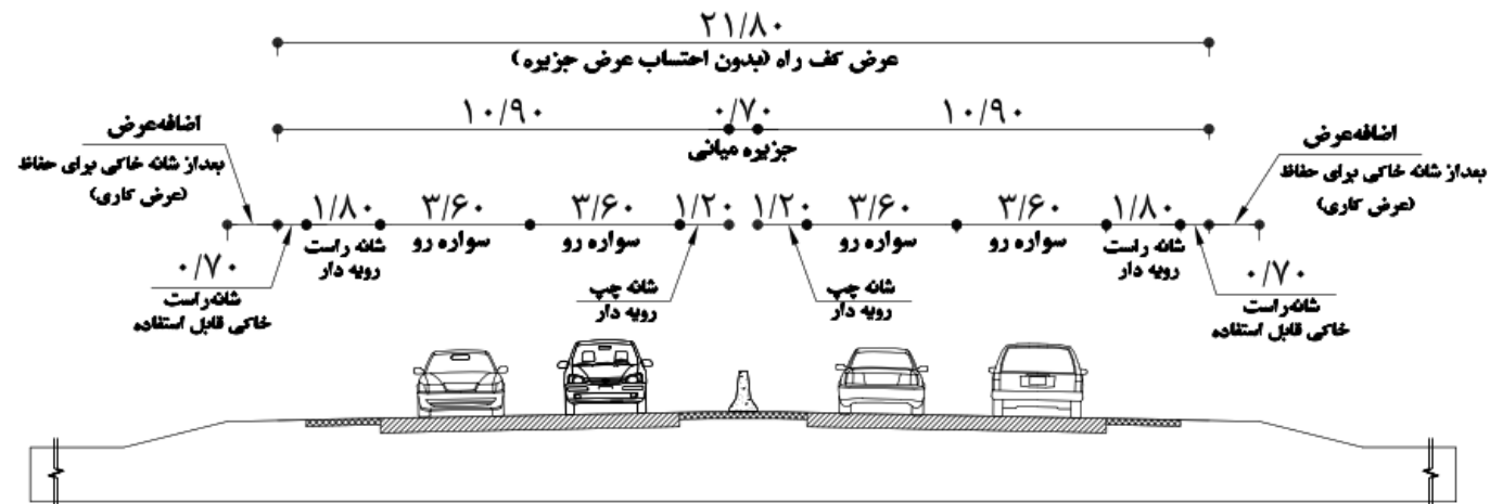
A1- راه شریانی جداشده چهار خطه
