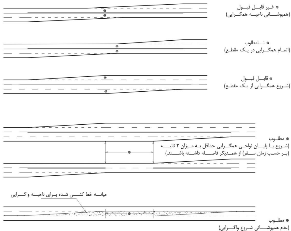
شکل ۵-۱۷- نمونه‌هایی از طرح‌های خط سبقت
