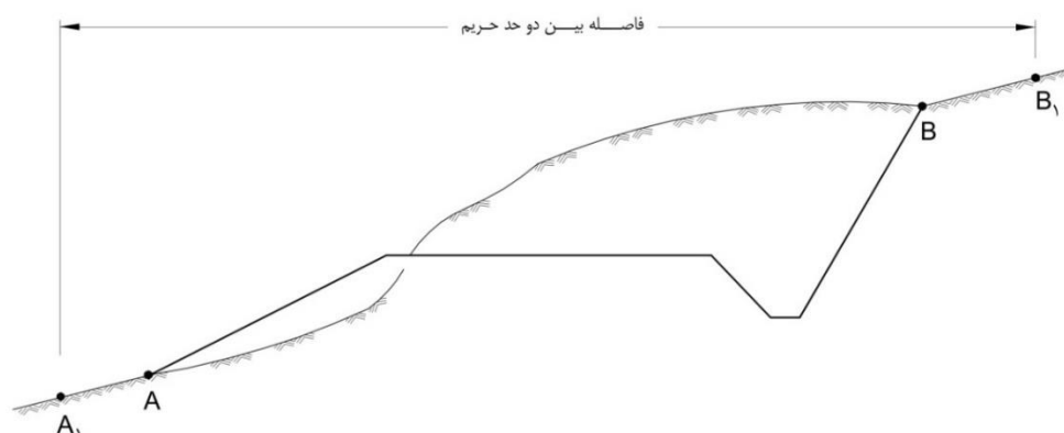
شکل ۶-۱۸- حریم راه
