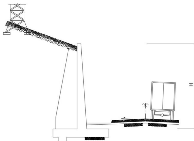
شکل ۶-۲۳- دیوار حائل با پشت بند
