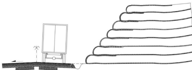
شکل ۶-۲۶- خاک مسلح با ژئوگرید
