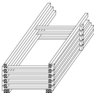
شکل ۶-۲۴- دیوار حائل صندوقه‌ای
