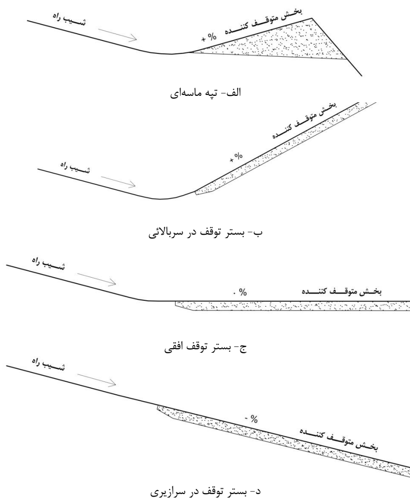
شکل ۵-۱۹- انواع رمپ‌های فرار اضطراری
