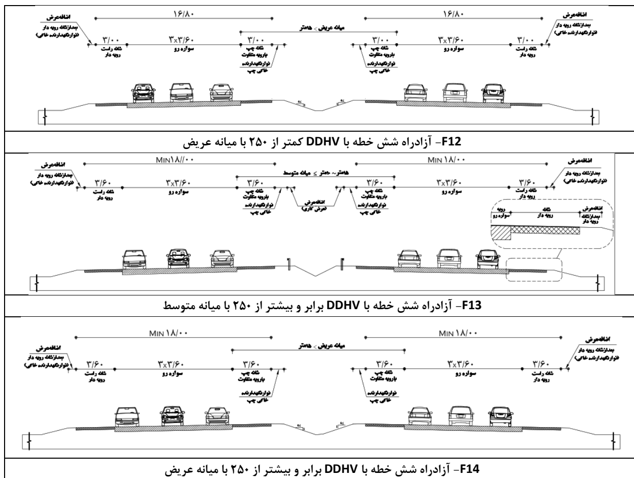
شکل ۶-۳۰- مقاطع عرضی نمونه برای آزادراه‌ها
