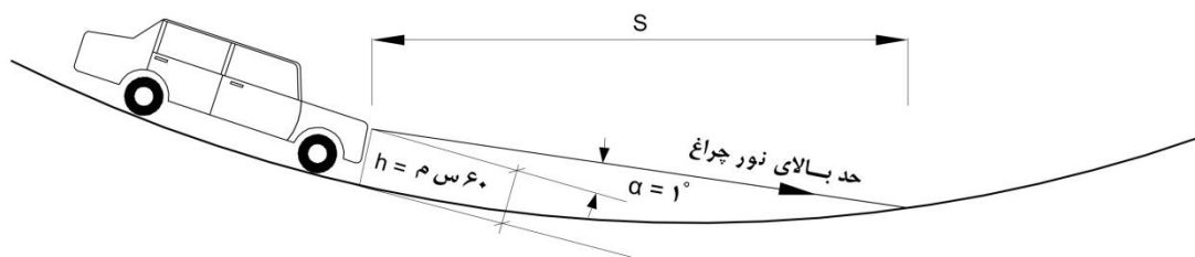
شکل ۵-۲۳- محدودیت دید در قوس قائم کاسه‌ای و در تاریکی شب
