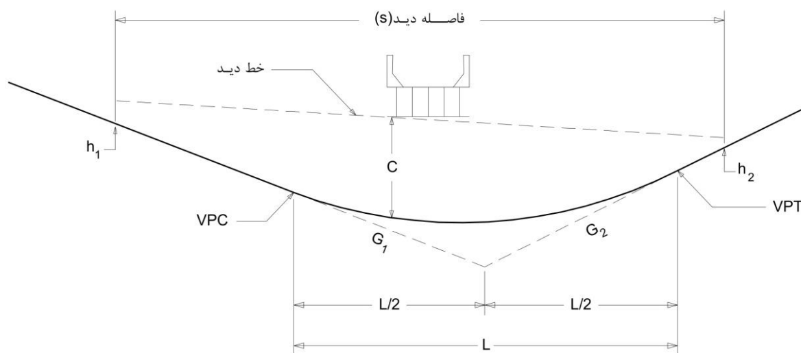
شکل ۵-۲۴- خط دید در خم کاسه‌ای
