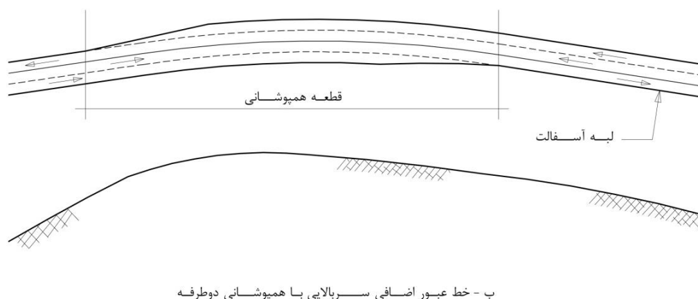
شکل ۵-۱۵- خط‌های کمکی سربالایی در راه‌های دو خطه دو طرفه
