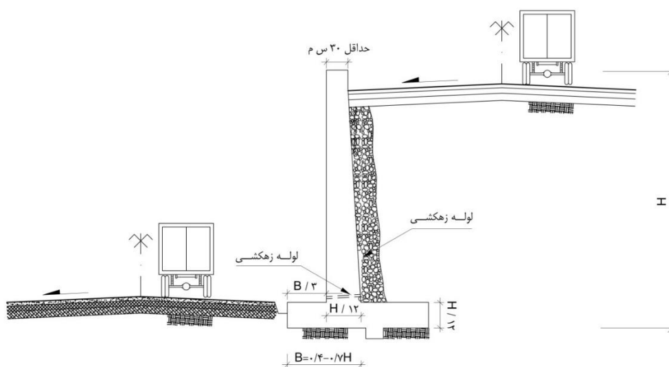
شکل ۶-۲۱- دیوار حائل وزنی
