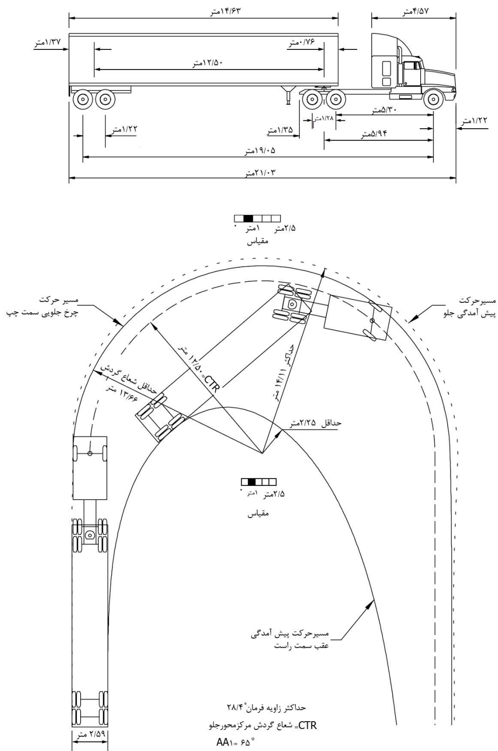
شکل ۴-۸- حداقل مسیر گردش برای وسیله طرح تریلی نوع ۲
