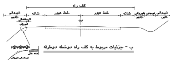
شکل ۶-۲- اجزای مقطع عرضی در راه‌های دو خطه و چهار خطه
