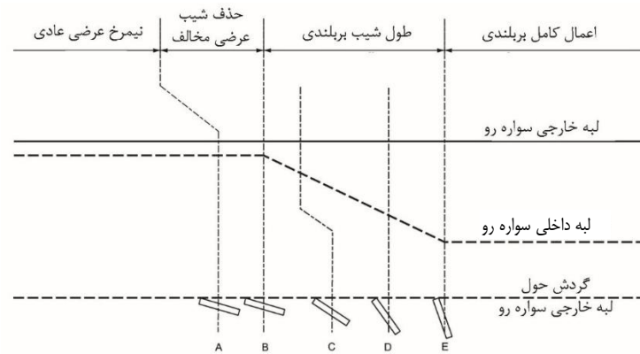
اعمال بر بلندی در سواره روی با شیب عرضی یک طرفه
