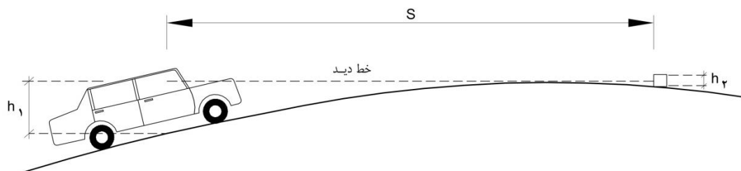
شکل ۵-۲۲- محدودیت دید در قوس قائم گنبدی
