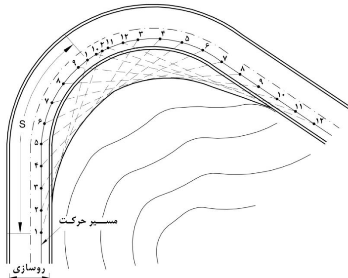
شکل ۵-۷- نحوه تعیین میزان بی‌مانع نمودن محوطه در قوس افقی
