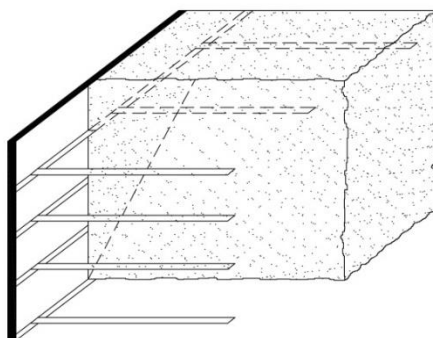
شکل ۶-۲۵- خاک مسلح
