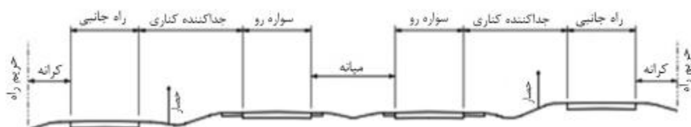
شکل ۶-۱۶- نمونه‌ای از مقطع عرضی راه شریانی جداشده با احتساب راه‌های جانبی
