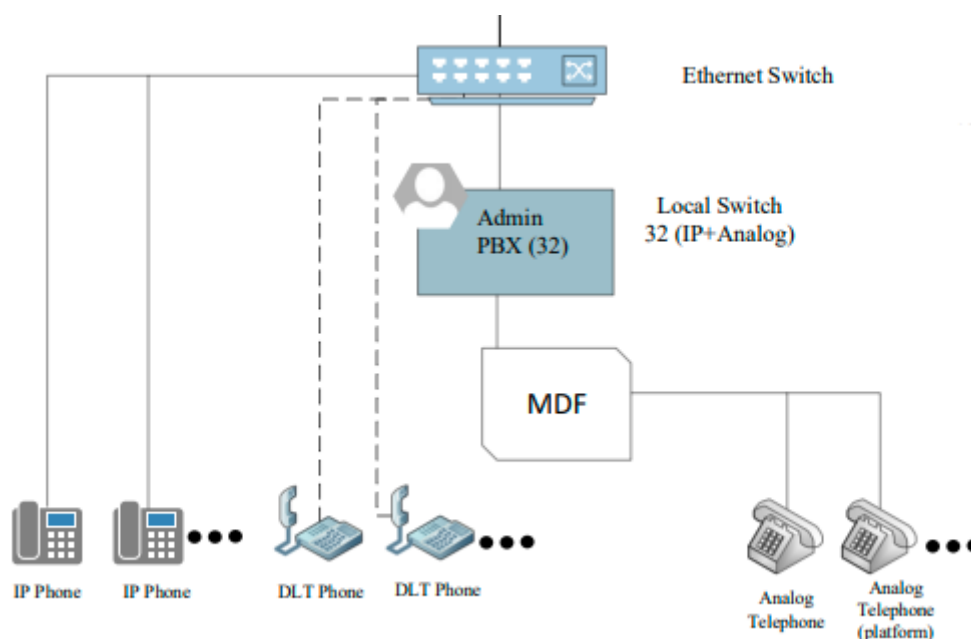
شکل ۳-۴ سیستم تلفن PABX
