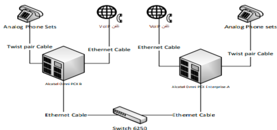
شکل ۳-۱ یک سیستم تلفن PABX
