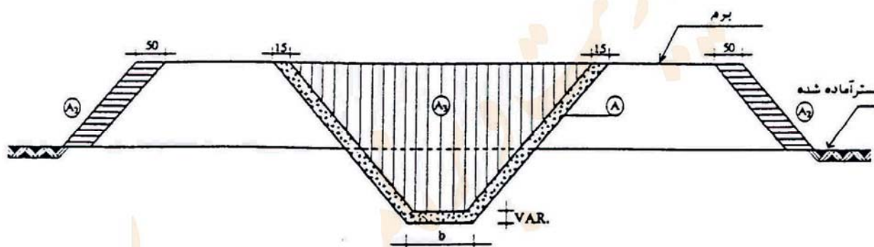
شکل ۳-۶. شمای مقطع خاکبرداری
