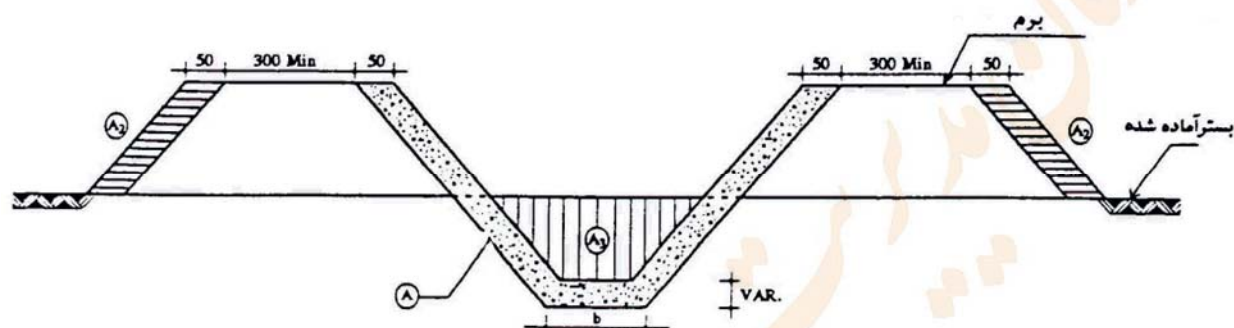
شکل ۵-۶. شمای مقطع خاکبرداری
