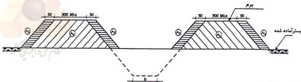
شکل ۴-۶. شمای مقطع خاکریزی
