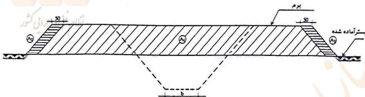
شکل ۲-۶. شمای مقطع خاکریزی
