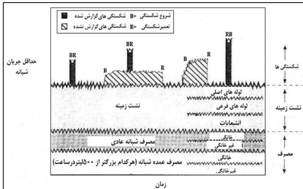
شکل ۱-۵-۱- اجزای حداقل جریان شبانه [۳۰]
