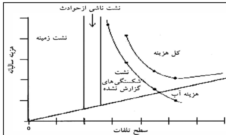
شکل ۳-۴- نمودار سطح اقتصادی کنترل نشت سالانه
