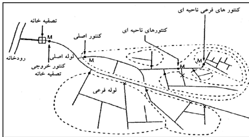
شکل ۱-۶-۱- تصویر عمومی یک منطقه مجزا
