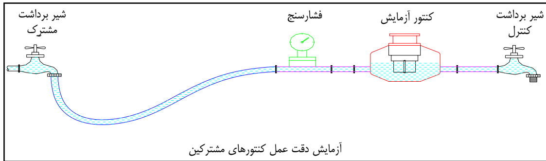
شکل ۲-۲- ابزار آزمایش کنتور در محل
