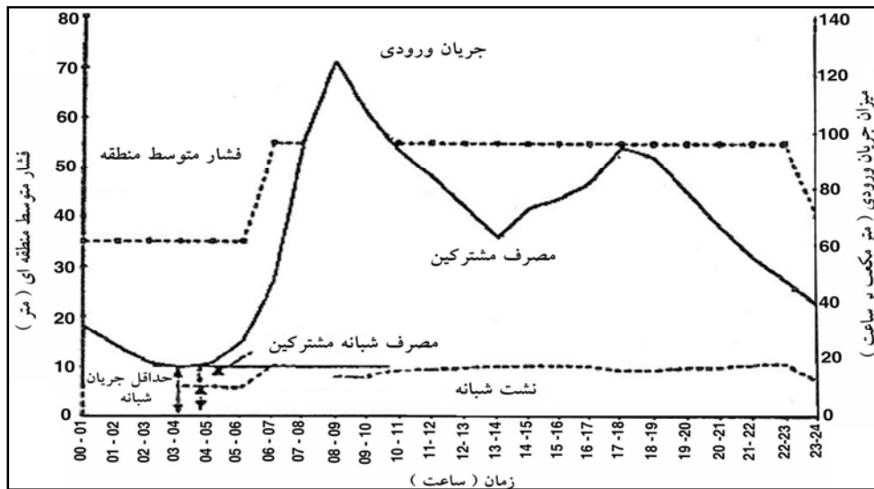
شکل ۱-۱۰- اجزای اصلی جریان ورودی به سامانه توزیع پس از مدیریت فشار [۱۸] (محور افقی متوسط زمان بین دو ساعت را نشان می دهد)
