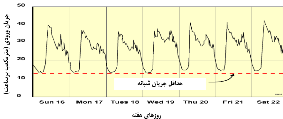
شکل ۱-۷-۱- حداقل جریان شبانه در یک شبکه
