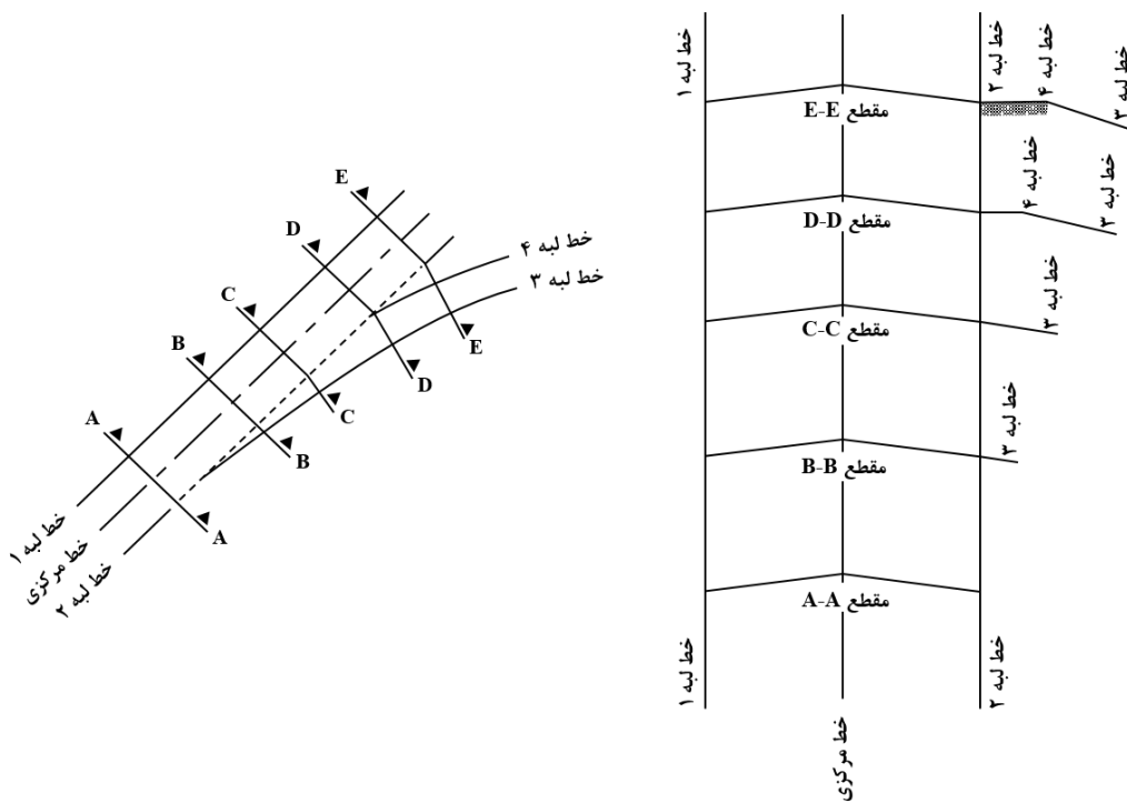
شکل ۳-۶- نحوه اعمال برابندی در خط گردش مماس بر خط اصلی مستقیم
