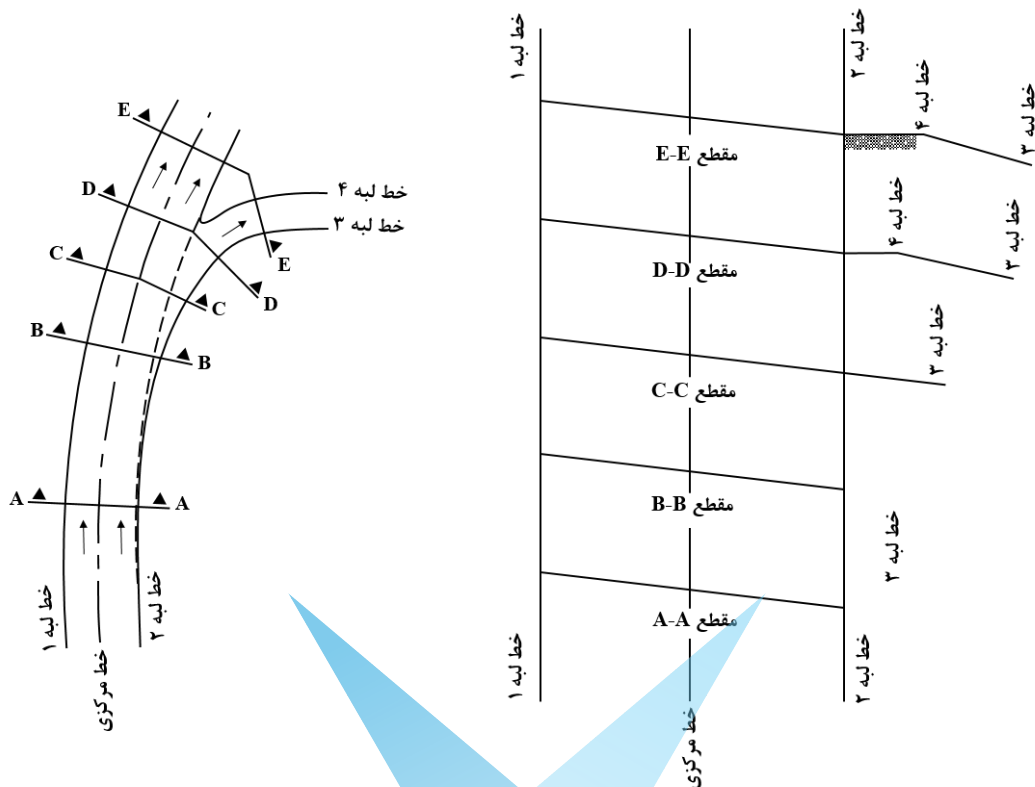
شکل ۳-۷- نحوه اعمال برابندی در خط گردش هم‌جهت با شیب خط اصلی در قوس افقی
