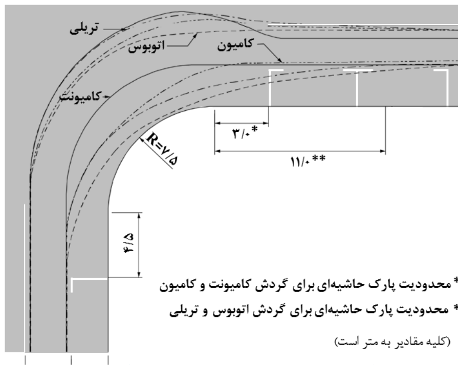
شکل ۳-۱۱- تأثیر وجود پارکینگ حاشیه‌ای بر مسیر گردش وسایل نقلیه و طراحی قوس گوشه تقاطع
