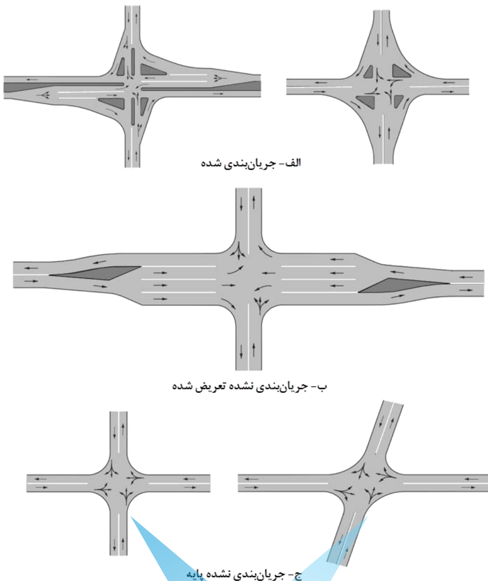
شکل ۱-۴- تقسیم‌بندی تقاطع‌ها به لحاظ جریان‌بندی ترافیک
