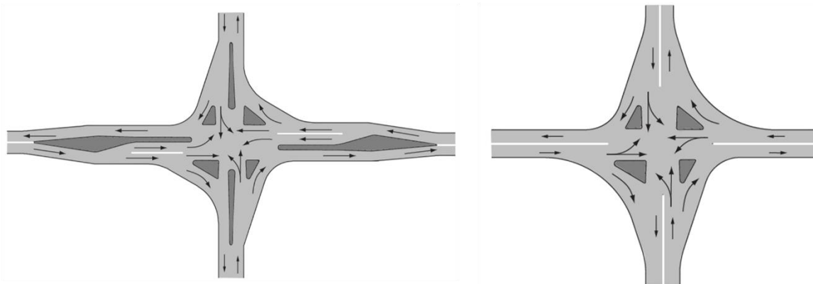
ب- تفکیک جریان‌ها به کمک خط‌کشی و تعریض
