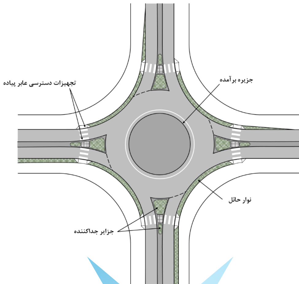
شکل ۱-۱- نمونه‌ای از میدان‌ها
