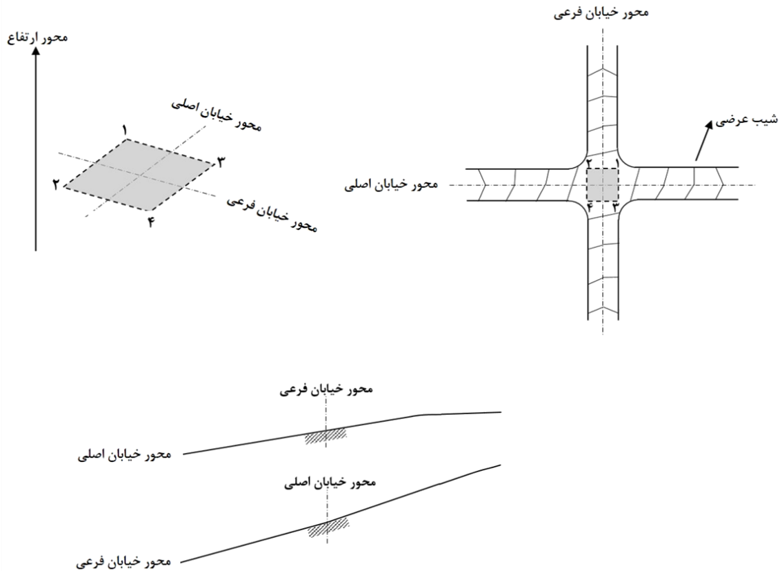
شکل ۱-۱۳- تغییر توأمان نیمرخ‌های عرضی و طولی خیابان‌های اصلی و فرعی در محل تقاطع
