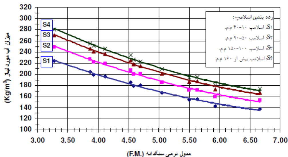
شکل پ-۲-۴- رابطه مقدار آب آزاد بتن و ضریب (مدول) نرمی سنگدانه هنگامی که به آب زیاد نیاز است (به دلیل تیزگوشگی سنگدانه‌ها)
