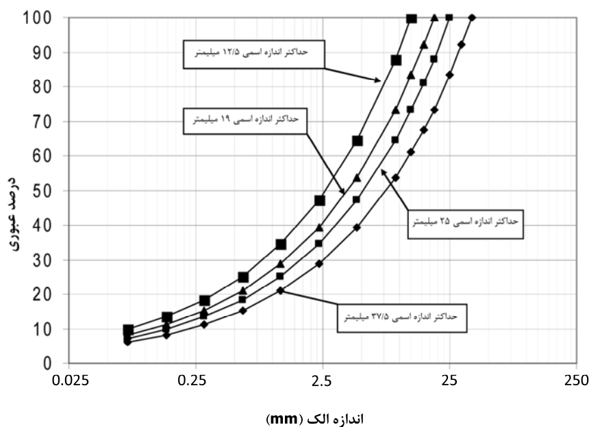
شکل ۳-۴۶- منحنی فولر-تامسون برای سنگ‌دانه با اندازه متفاوت
