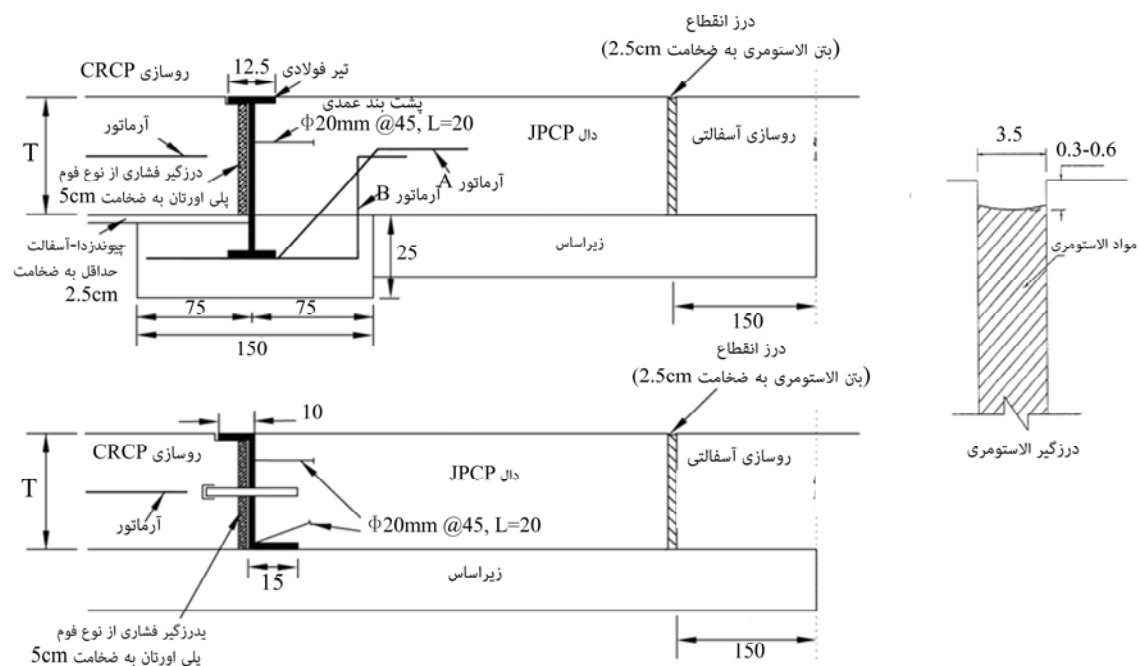
شکل ۳۶-۲- ناحیه انتقال برای اتصال روسازی بتنی مسلح پیوسته (CRCP) به روسازی آسفالتی (AC) با استفاده از بتن الاستومری (درخصوص جزئیات تیرهای فولادی و آرماتورهای A و B به شکل‌های (۳۷-۲) و (۳۸-۲) مراجعه شود)
