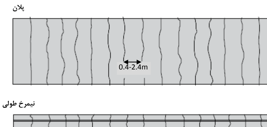
شکل ۹-۱- نمای کلی روسازی بتنی مسلح پیوسته
