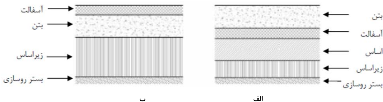
شکل ۲۱-۱- دو تیپ مختلف از روسازی‌های ترکیبی (الف - روسازی ترکیبی با رویه بتنی، ب - روسازی ترکیبی با رویه آسفالتی)
