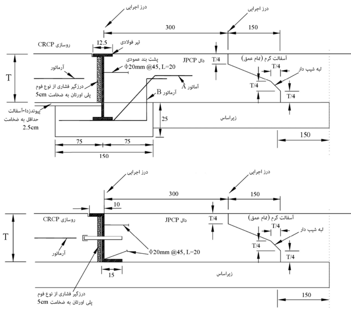
شکل ۳۵-۲- ناحیه انتقال برای اتصال روسازی بتنی مسلح پیوسته (CRCP) به روسازی آسفالتی (AC) با استفاده از دال با ضخامت متغیر (درخصوص جزئیات تیرهای فولادی و آرماتورهای A و B به شکل‌های (۲-۳۷) و (۲-۳۸) مراجعه شود)
