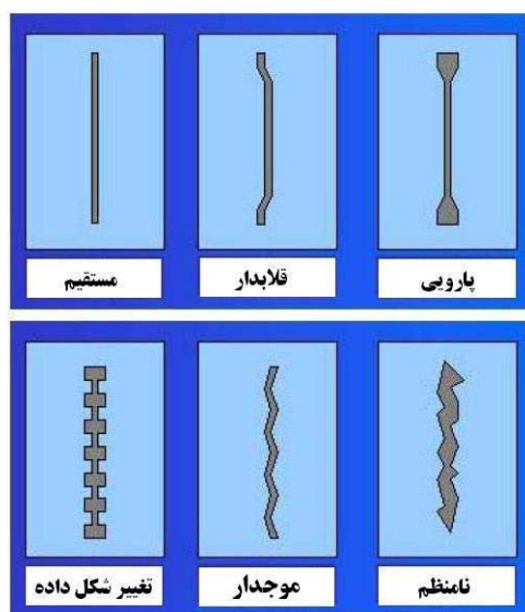
شکل ۱-۱۷- انواع مختلف الیاف فولادی
