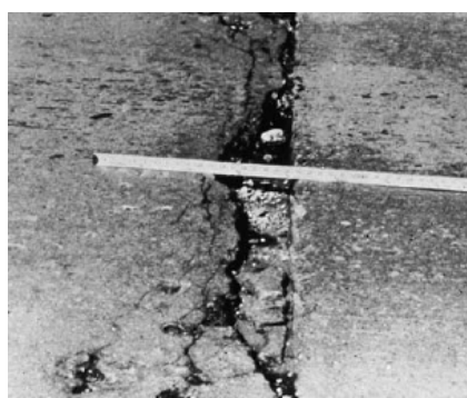
خردشدگی درز با شدت زیاد
