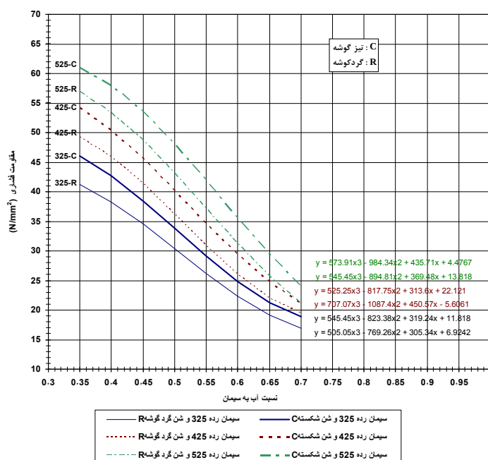
شکل پ-۲-۱- رابطه نسبت آب به سیمان و مقاومت فشاری بدون مصرف روان کننده
