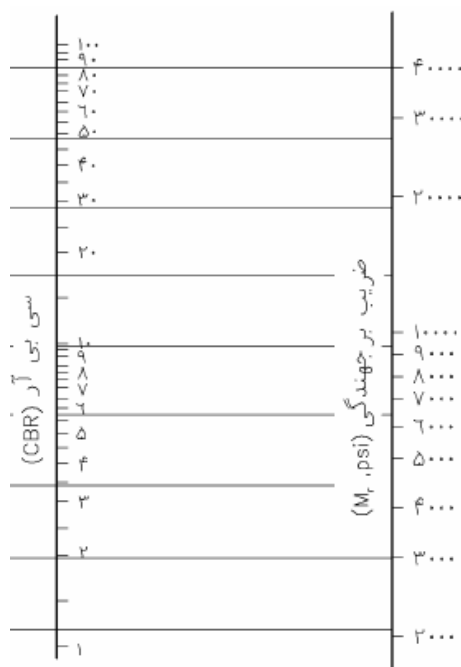
شکل ۲-۷- نمودار تعیین ضریب برجهندگی خاک بستر روسازی با استفاده از مقادیر CBR (1psi=6.89 kPa)
