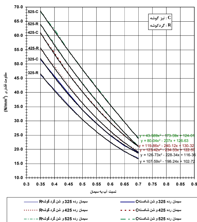
شکل پ-۲-۲- رابطه نسبت آب به سیمان و مقاومت فشاری با توجه به مصرف روان کننده
