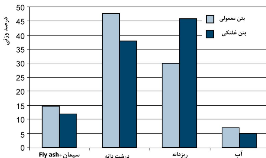
شکل ۱-۲- مقایسه درصد مصالح تشکیل‌دهنده بتن غلتکی و بتن معمولی
