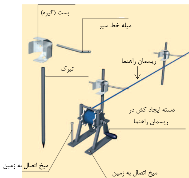
شکل ۳-۲۶- اجزای مربوط به عملیات نصب ریسمان راهنما
