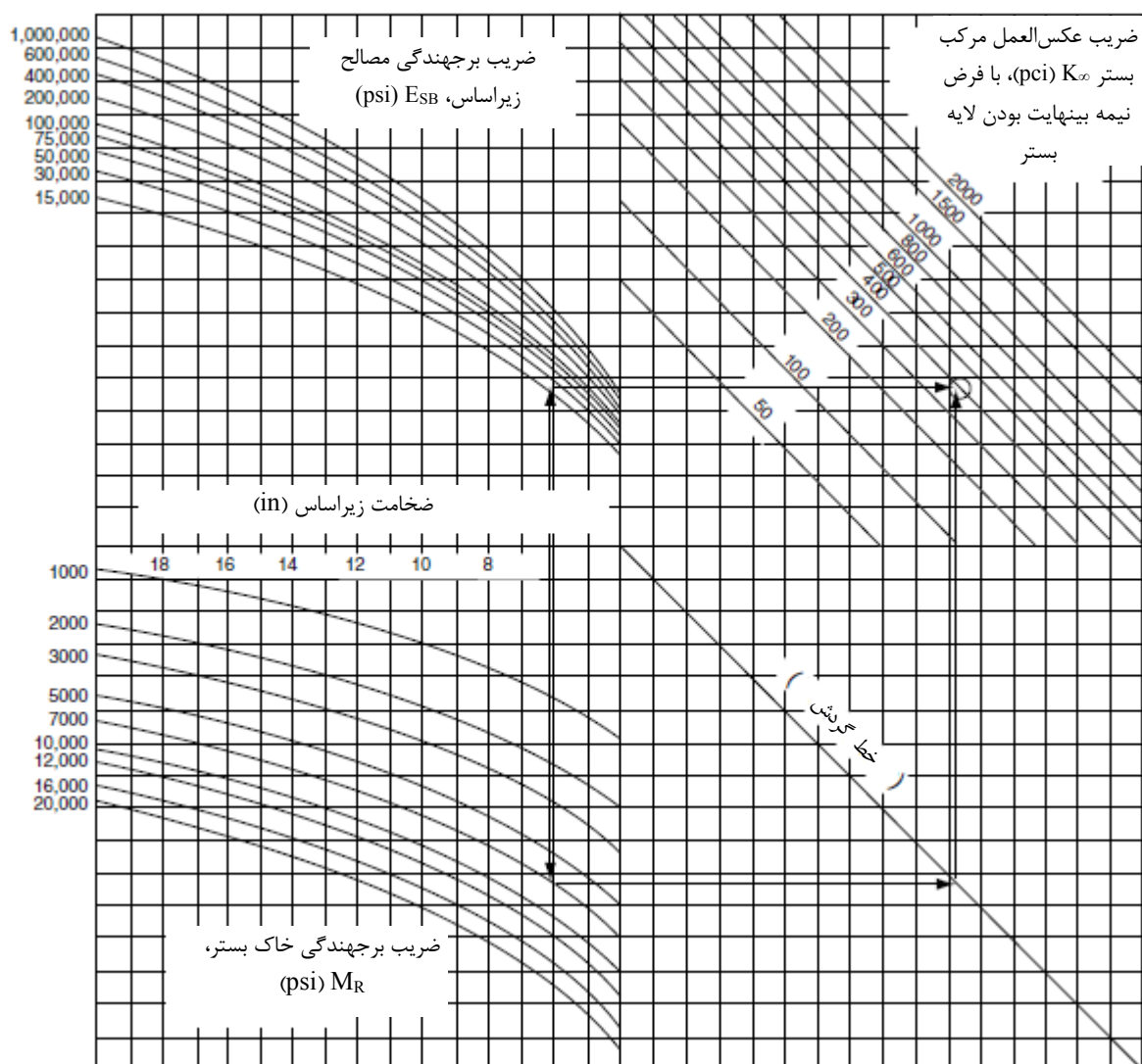
شکل ۲-۹- تعیین ضریب عکس‌العمل مرکب بستر (به علت وجود لایه زیراساس)
