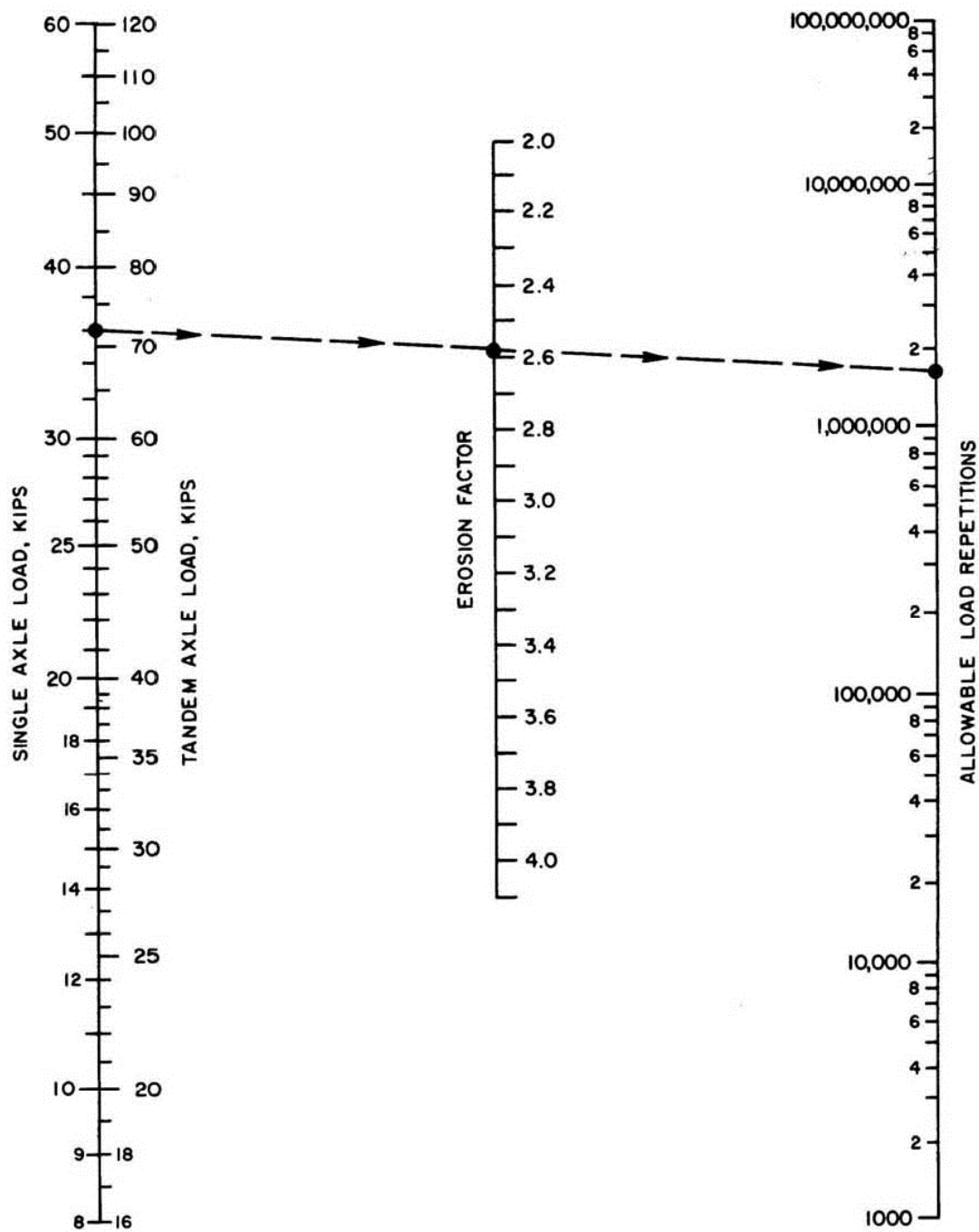
شکل پ-۱-۹-الف- محاسبه تعداد مجاز تکرار بار برای دال‌های بدون شانه بتنی در تحلیل فرسایش
