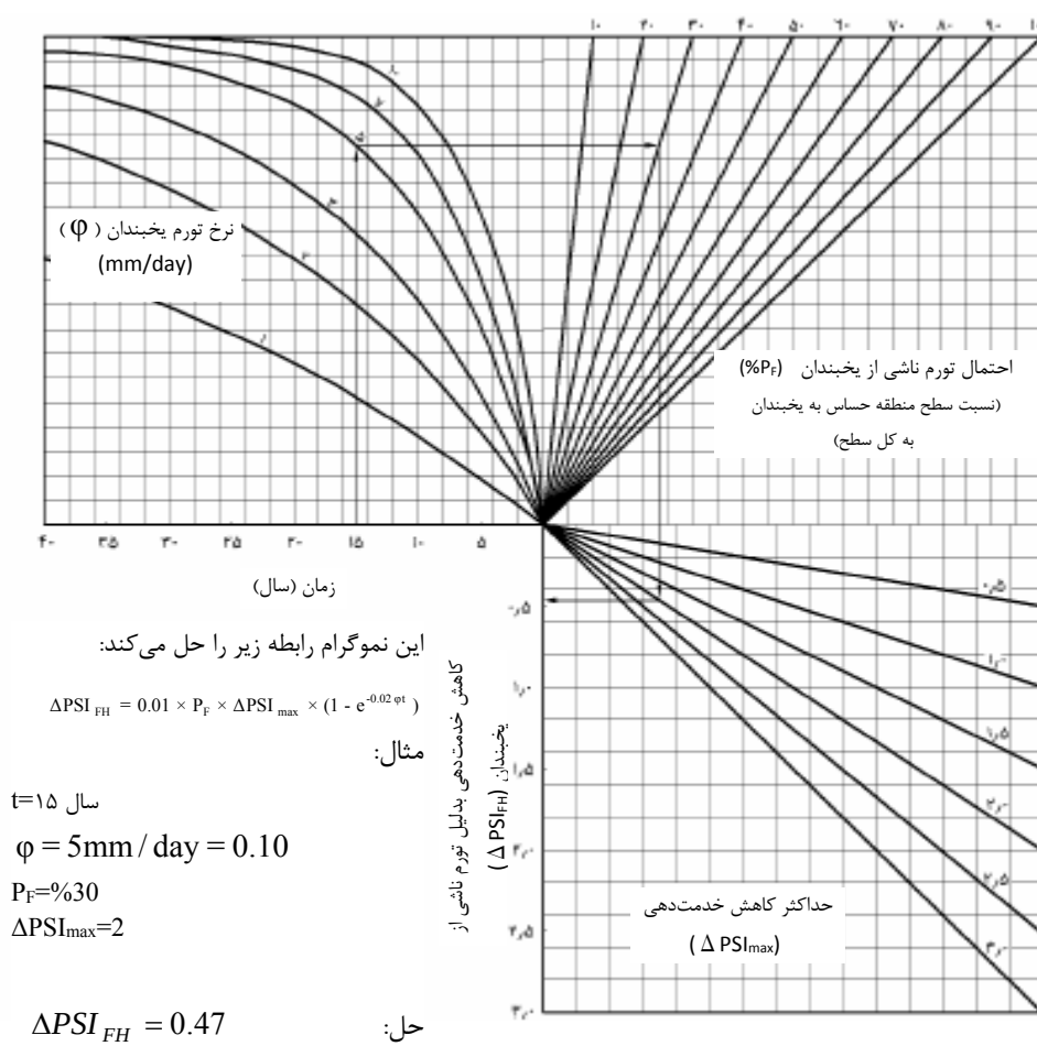
شکل ۲-۴ - نمودار تخمین کاهش نشانه خدمت‌دهی به دلیل بالا آمدگی ناشی از یخبندان
