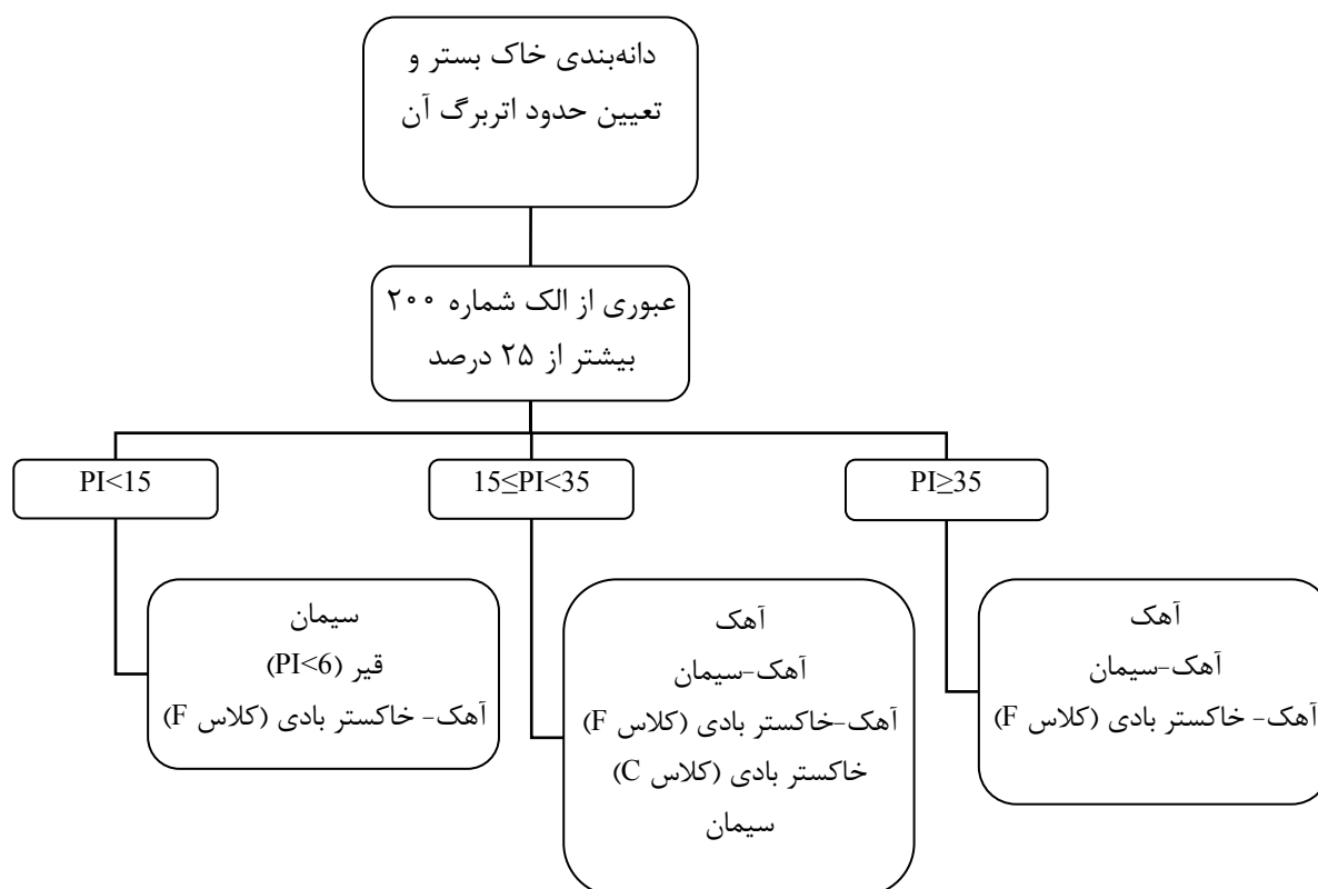
شکل ۳-۱- انتخاب ماده تثبیت کننده بستر
