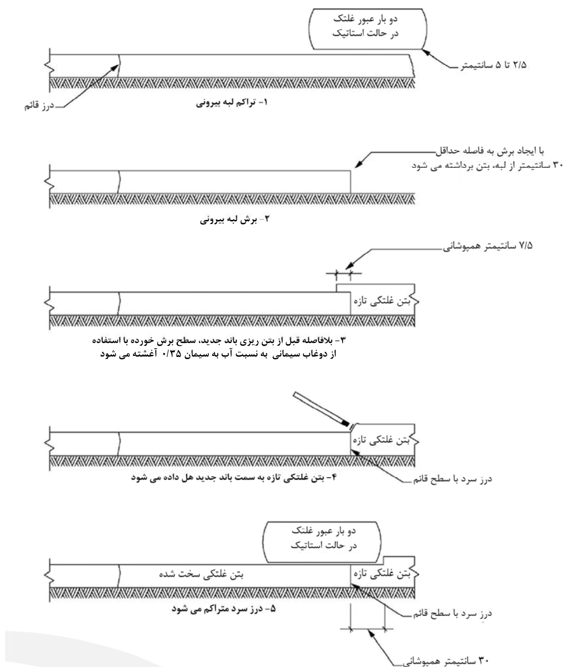
شکل ۳-۵۱- نحوه اجرای درز سرد در روسازی بتن غلتکی
