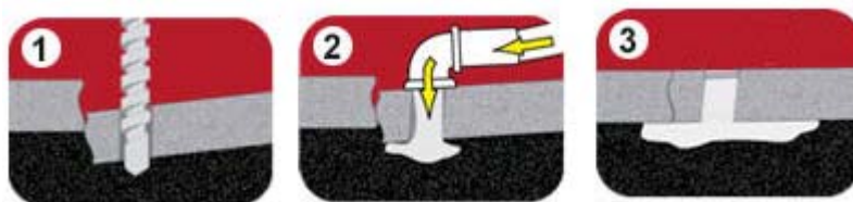
شکل ۴-۴۴- نمایی کلی از عملیات بالا آوردن دال
