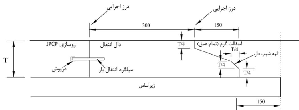
شکل ۲-۲۲- ناحیه انتقال برای اتصال روسازی بتنی ساده درزدار (JPCP) به روسازی آسفالتی (AC) با استفاده از دال با ضخامت متغیر
