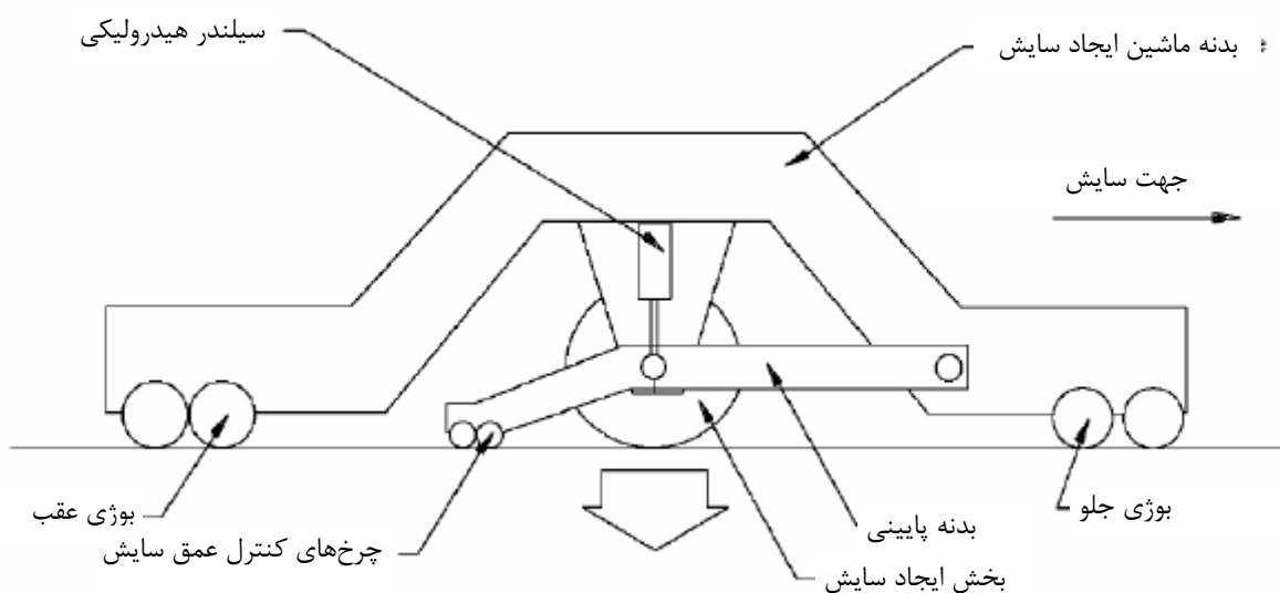
شکل ۴-۳۴- نمای شماتیک از ماشین ایجاد سایش
