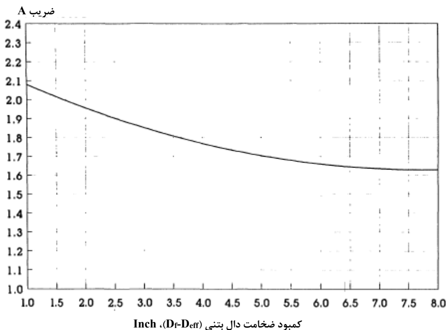
شکل ۴-۵۴- تغییرات ضریب A برحسب کمبود ضخامت ( D_f - D_{eff} ) (1in=۲۵/۴ mm)
