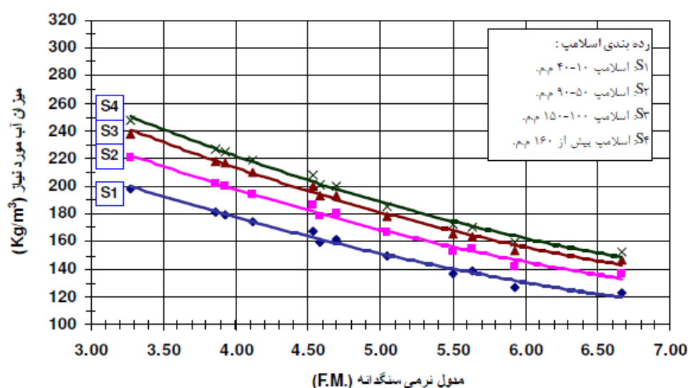
شکل پ-۲-۳- رابطه مقدار آب آزاد بتن و ضریب (مدول) نرمی سنگدانه هنگامی که به آب کم نیاز است (به دلیل گردگوشگی سنگدانه‌ها)
