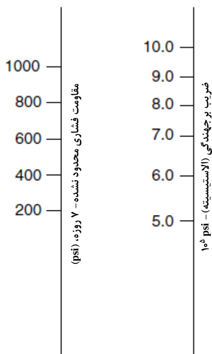
شکل ۱۰-۲- نمودار تعیین ضریب برجهندگی زیراساس تثبیت شده با سیمان
