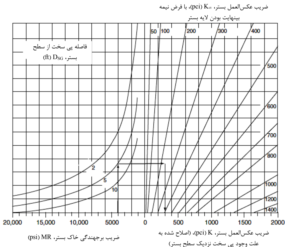
شکل ۲-۱۱- اصلاح ضریب عکس‌العمل بستر به علت وجود پی سخت در فاصله کمتر از ۳ متر از سطح بستر
