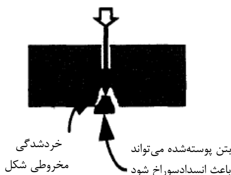
شکل ۴-۴۳- بروز خردشدگی مخروطی شکل هنگام حفر سوراخ در دال بتنی
