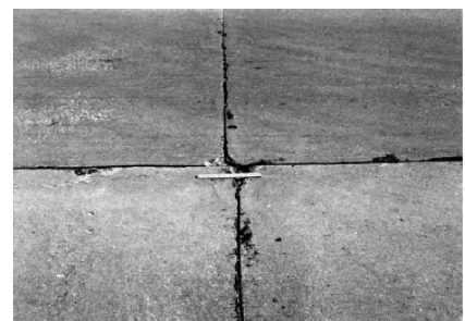
خردشدگی گوشه با شدت کم
