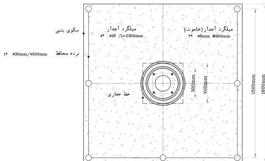
شکل ۳-۱ پیلار روی پی سنگی
