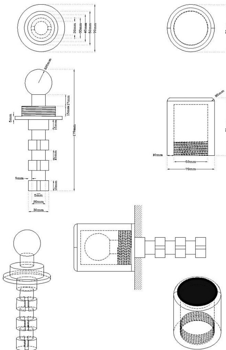
شکل ۳-۱۷ شکل پیشنهادی نقطه ارتفاعی گالری
