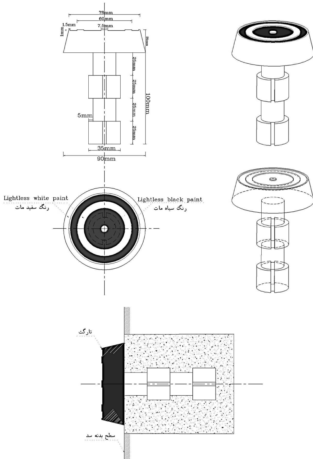
شکل ۹-۰ نقطه نشانه غیر قابل دسترس
