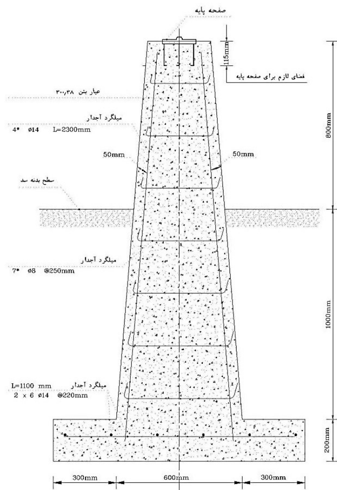
Sec. A-A
