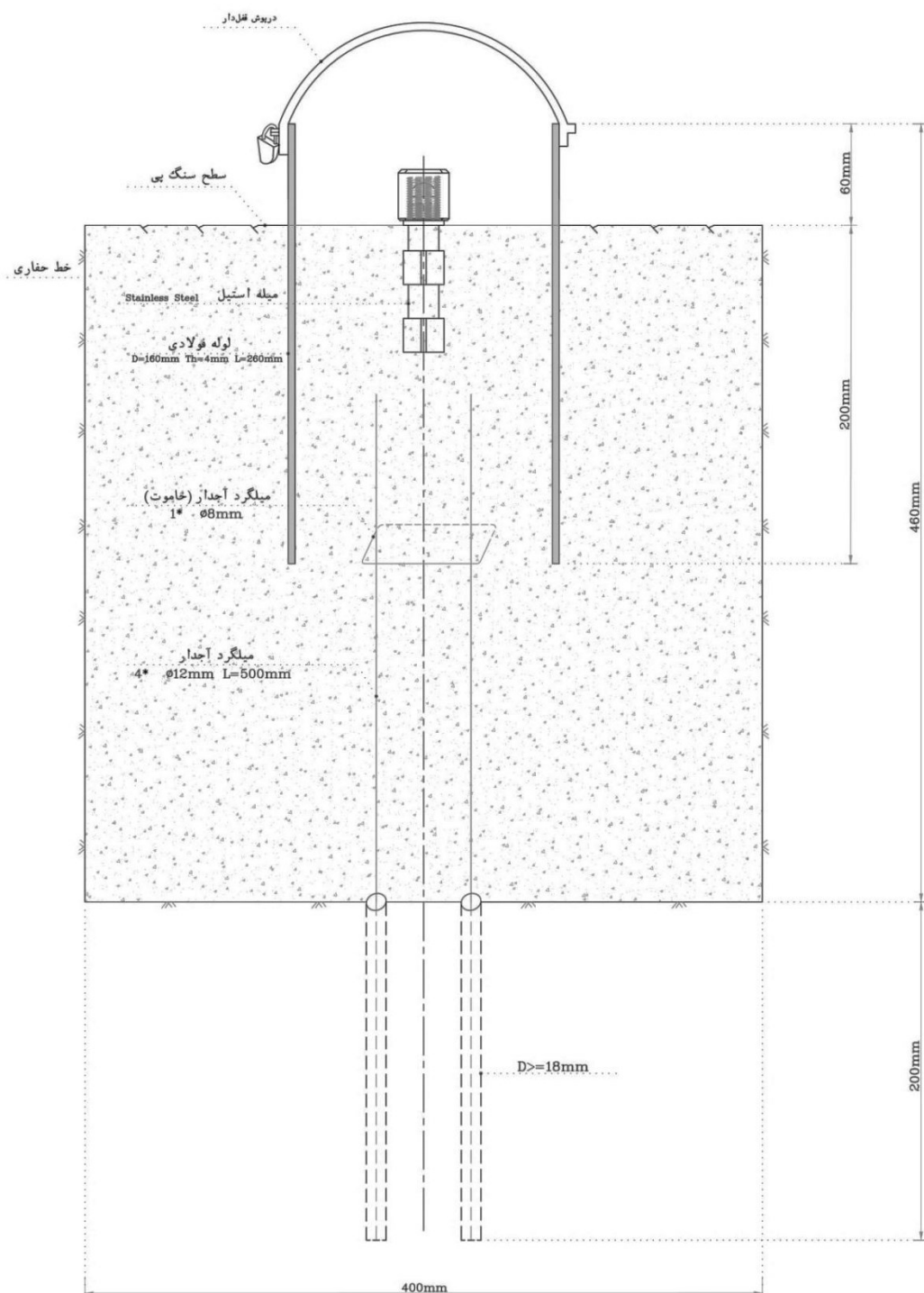
شکل ۴-۰ نقطه مبنای ارتفاعی روی پی سنگی
