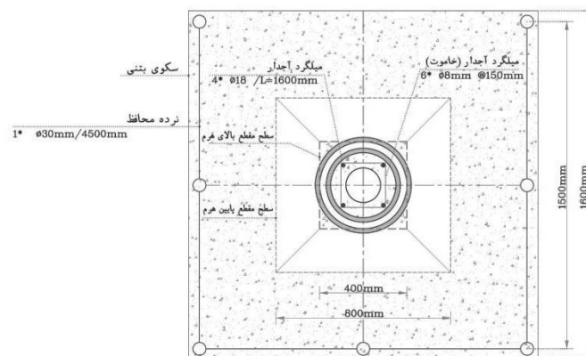
شکل ۳-۳ پیلار روی پی غیر سنگی یا روی تاج سد خاکی
