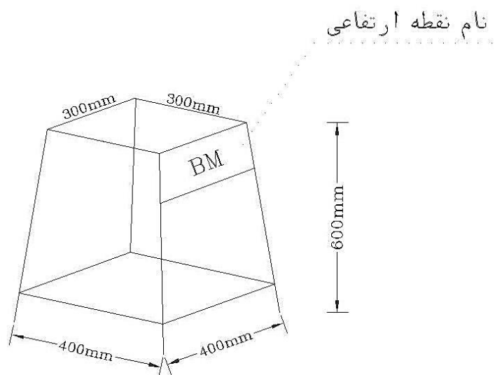
شکل ۶-۵ تابلو چهارپایه
