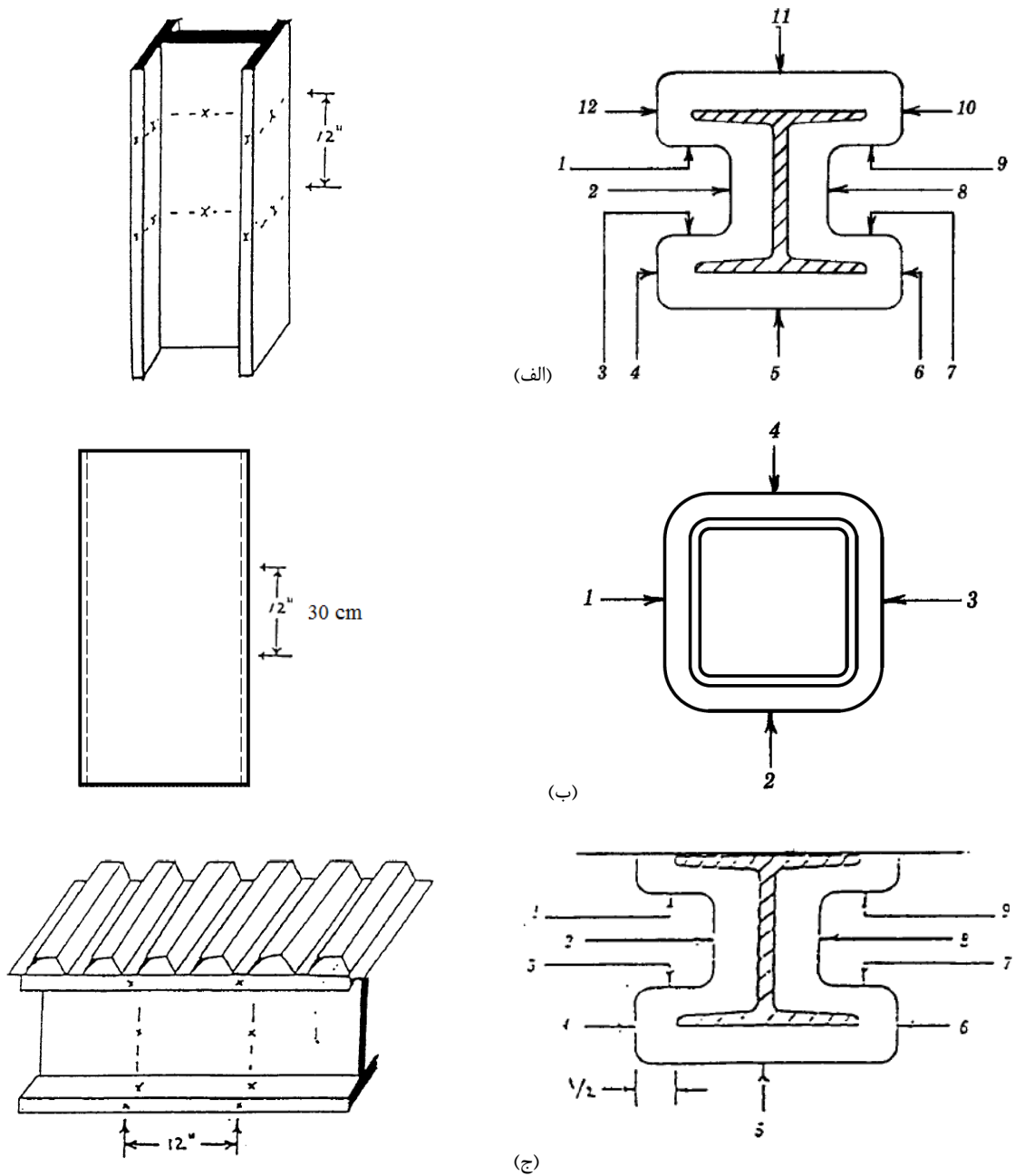
شکل ۴-۹- نقاط کنترل ضخامت پوشش محافظ حریق: (الف) ستون فولادی با مقطع I شکل؛ (ب) ستون فولادی با مقطع مستطیلی توخالی و (ج) تیر فولادی با مقطع I شکل همراه با دال بتنی
