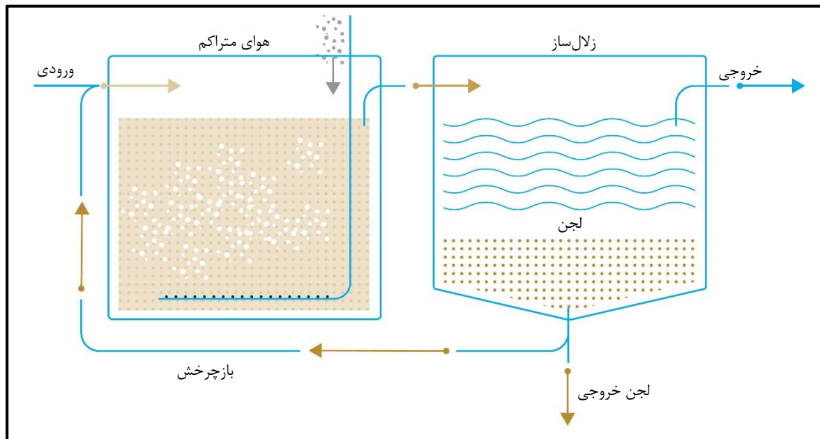
شکل ۸-۱۲- لجن فعال - هوادهی گسترده
