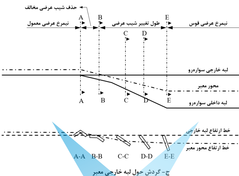
شکل ۳-۲ - شیوه‌های مختلف اعمال بر بلندی
