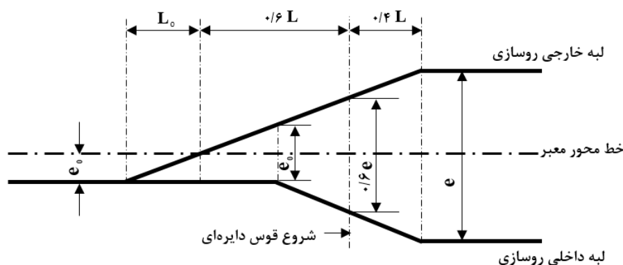
شکل ۳-۴- نحوه تغییر مقطع عرضی و اعمال بر بلندی قبل از قوس‌های ساده
