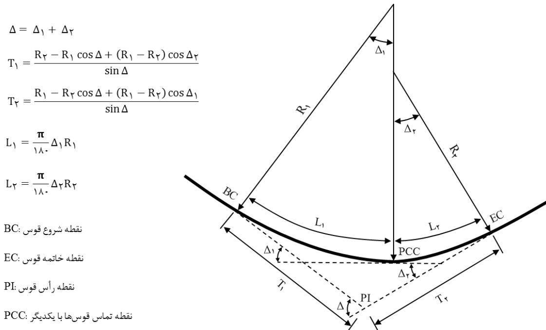
شکل ۱-۲- مشخصات هندسی قوس افقی مرکب دو مرکزی
