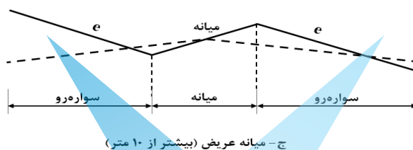
شکل ۳-۳ - حالت‌های مختلف نحوه اعمال برابندی در معابر دارای میانه
