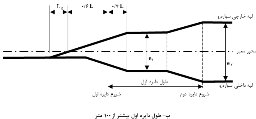
شکل ۳-۵- نحوه تغییر مقطع عرضی و اعمال بریلندی قبل از قوس‌های مرکب
