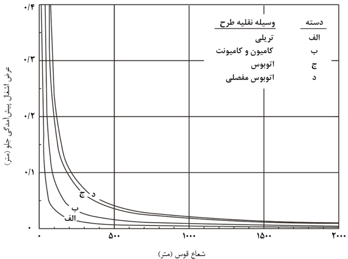
شکل ۷-۳- عرض اشغال پیش آمدگی جلو انواع وسایل نقلیه در قوس‌های افقی
