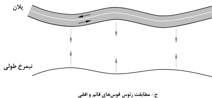
شکل ۵-۲- نمونه‌های وجود هماهنگی بین پلان و نیمرخ طولی
