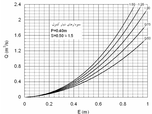
شکل ۲-۶ نمودارهای طراحی مقطع شیار کنترل
