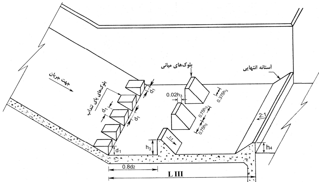
شکل ۴-۵ حوضچه آرامش نوع USBR-III ( Fr_1 > 4.5, V_1 < (15-16) \text{ m/s} )
