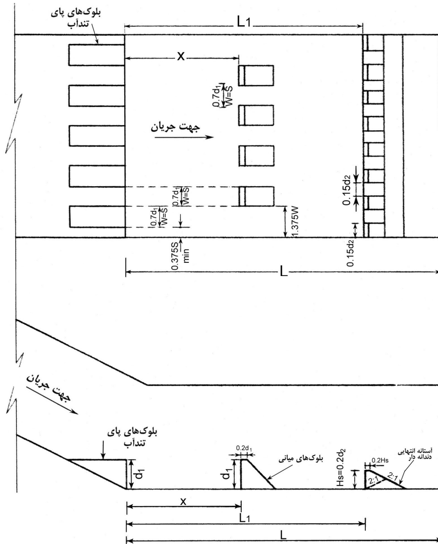
شکل ۴-۱۱- پلان و مقطع حوضچه آرامش نوع اصلاح شده و ابعاد بلوک‌های پای تندآب، بلوک‌های میانی و آستانه انتهایی دندانه‌دار
