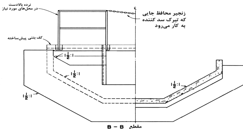
شکل ۲-۲ تلفیق نوعی شیب شکن قائم و سازه تنظیم سطح آب برای بده کم تر از ۲ متر مکعب بر ثانیه و ارتفاع ۰/۵ متر (نوع USBR)
