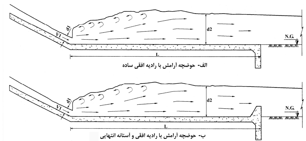
شکل ۳-۴ حوضچه آرامش نوع USBR-I ( 1.7 < Fr_1 < 2.5 )
