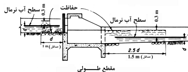
شکل ۲-۴ حفاظت در برابر فرسایش برای شیب‌شکن‌های قائم
