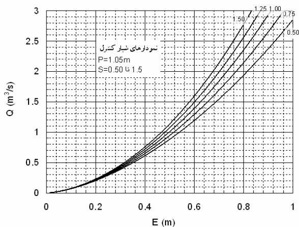
ادامه شکل ۲-۶ نمودارهای طراحی مقطع شیار کنترل
