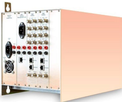
شکل ۲-۲۲- یک نمونه مبدل تلویزیونی هتلی
