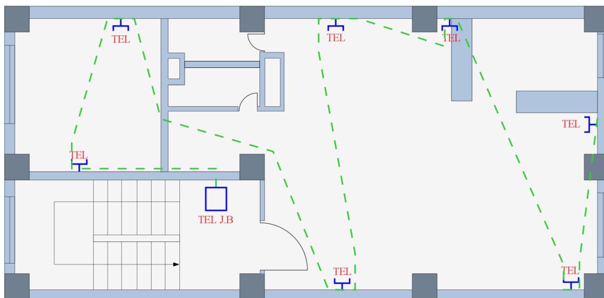
شکل ۱-۱- نقشه سیم‌کشی پریز تلفن
