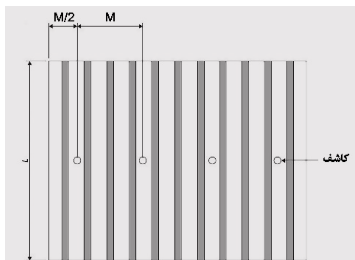
شکل ۴-۴۸- مثال: در این مثال عمق تیر بیش‌تر از 10\% ارتفاع سقف است ( H = 3m ) و از دتکتور دودی استفاده شده است، بنابراین طبق
