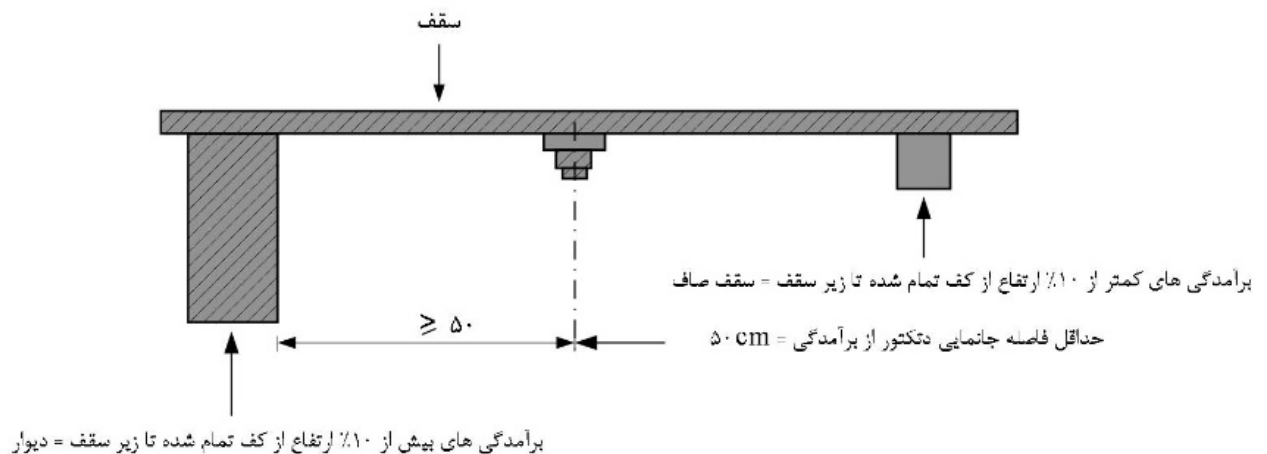
شکل ۴-۴۴- موانع موجود در سقف
