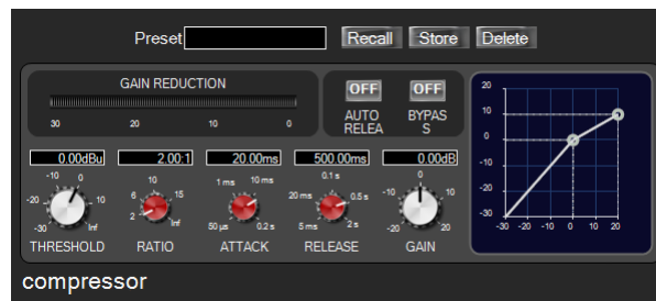
شکل ۷-۵۲ - نمونه کنترل نرم‌افزاری کمپرسور دیجیتال
