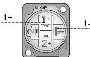
WIRING
