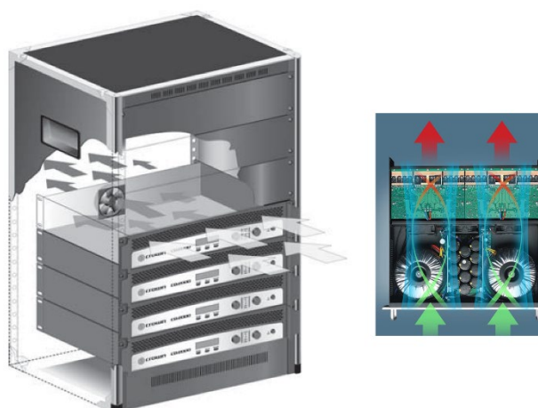
شکل ۷-۸۸- نحوه گردش هوا در تقویت‌کننده‌ها در داخل رک
