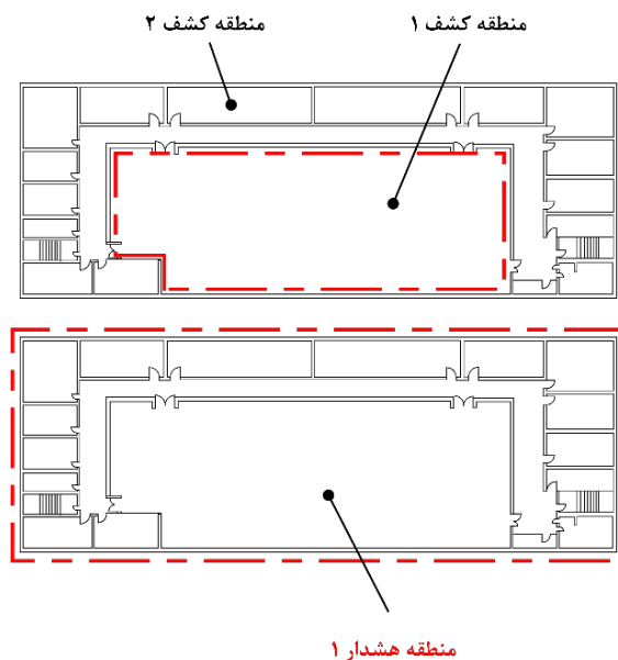
شکل ۴-۱۹- منطقه هشدار
