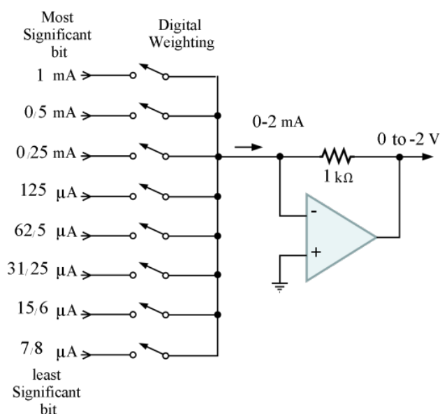
شکل ۷-۱۵- نمونه ساده شده مبدل متعارف نردبانی
