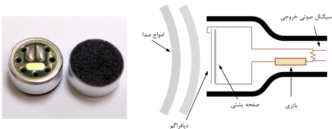
شکل ۷-۲۷- ساختمان داخلی و یک نمونه کپسول میکروفن خازنی
