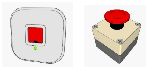
شکل ۳-۷- نمونه‌هایی از دتکتور هشدار سرقت مسلحانه
