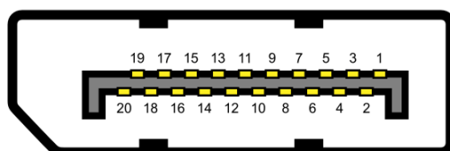
شکل ۸-۳۰- شماره پایه‌های سوکت DP
