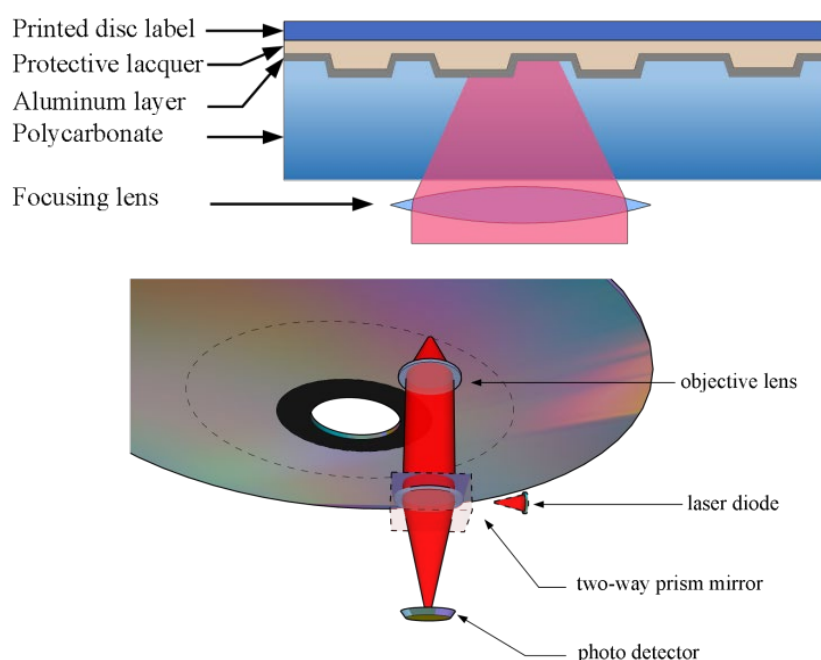
شکل ۷-۹۸- ساختار دیسک و خواندن اطلاعات یک دیسک
