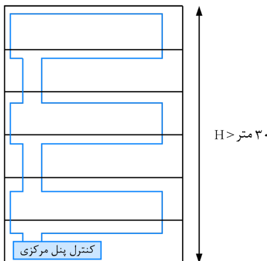
شکل ۴-۷۲- استفاده از کابل مقاوم در برابر حریق ارتفاع یافته در ساختمانی با ارتفاع بیش از ۳۰ متر (بدون شبکه بارنده خودکار)
