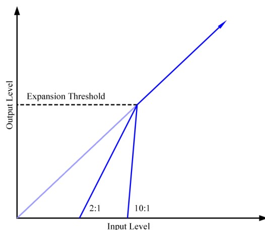
شکل ۷-۵۵- منحنی تابع دستگاه اکسپندر
