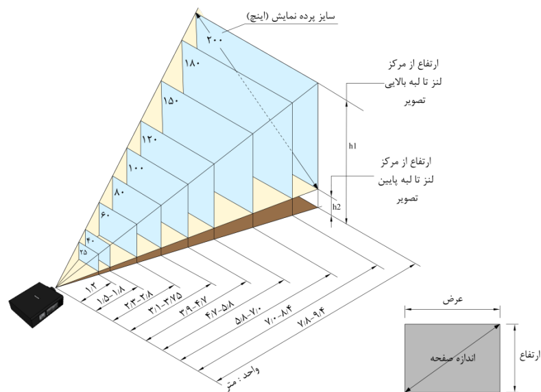
شکل ۸-۳۴- یک نمونه فاصله ویدیو پروژکتور متناسب با ابعاد پرده
