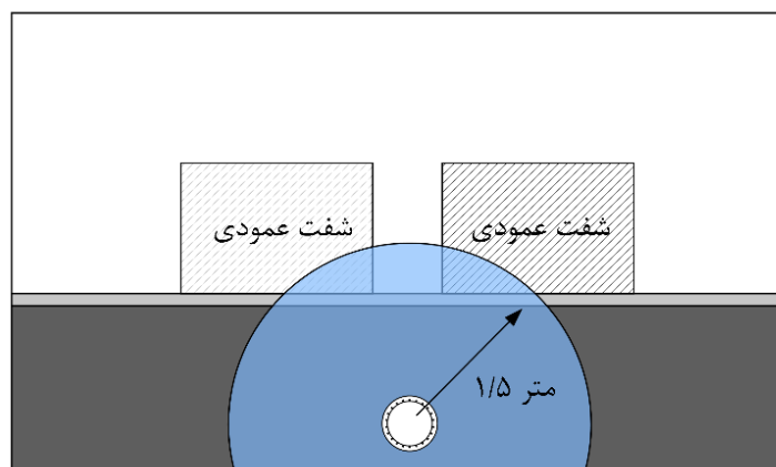
شکل ۴-۳۰- حداکثر فاصله جانمایی دتکتور دودی نقطه‌ای از بازشوها
