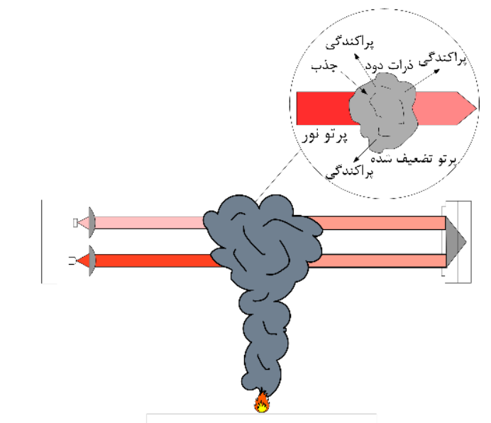
شکل ۴-۱۱- عملکرد دتکتور دودی خطی نوع منعکس کننده
