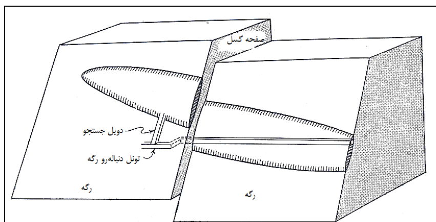
شکل ۵-۷- حفر دوبل برای یافتن بخش قطع شده ماده معدنی به وسیله یک گسل پرسیب
