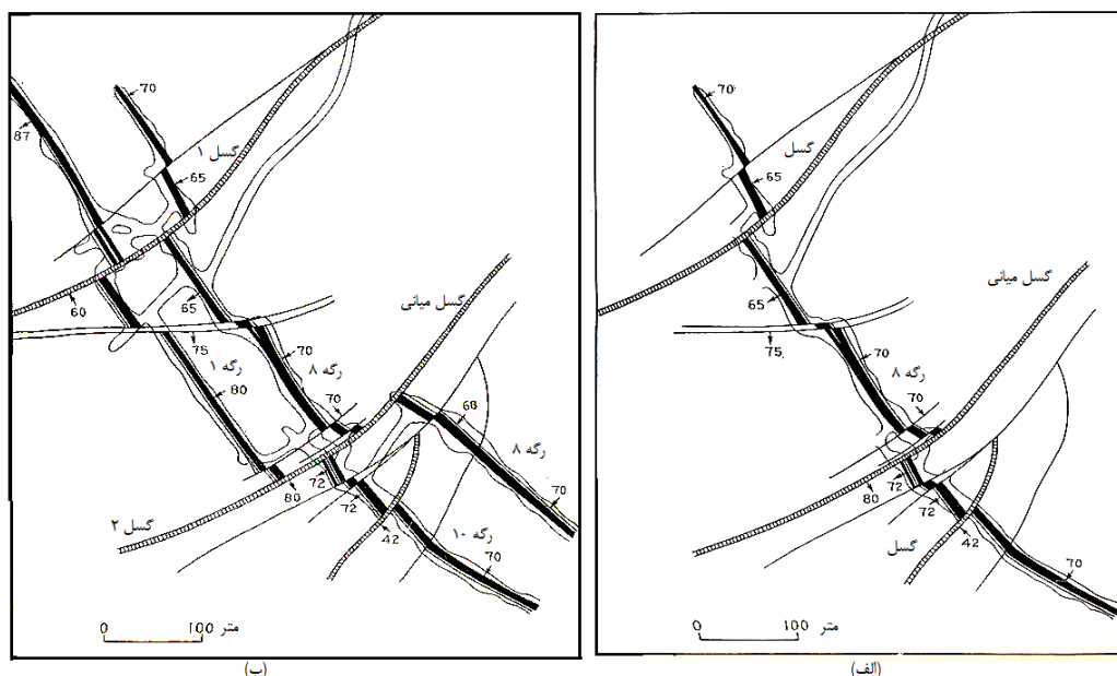
شکل ۵-۶- یافتن رگه جدیدی از ماده معدنی در اثر حفريات جستجوی گسل
