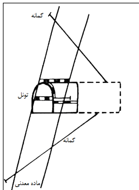
شکل ۸-۳- موقعیت نمونه برداری در مورد تونل‌های دنباله‌رو در مواد معدنی ضخیم
