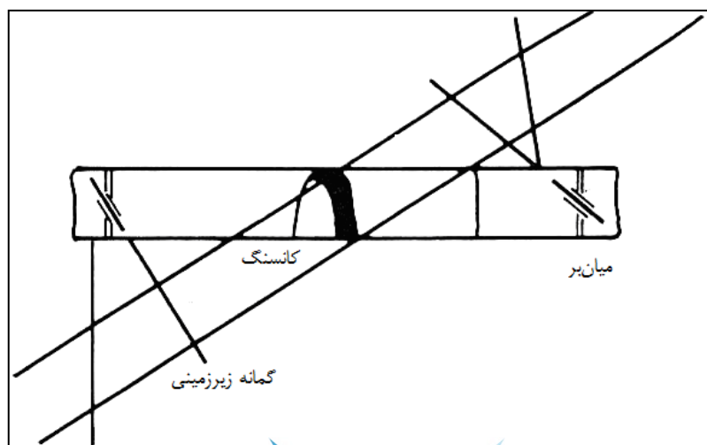
شکل ۹-۳- حفر میان‌بر دوگانه به فواصل منظم از درون تونل‌های دنباله‌رو
