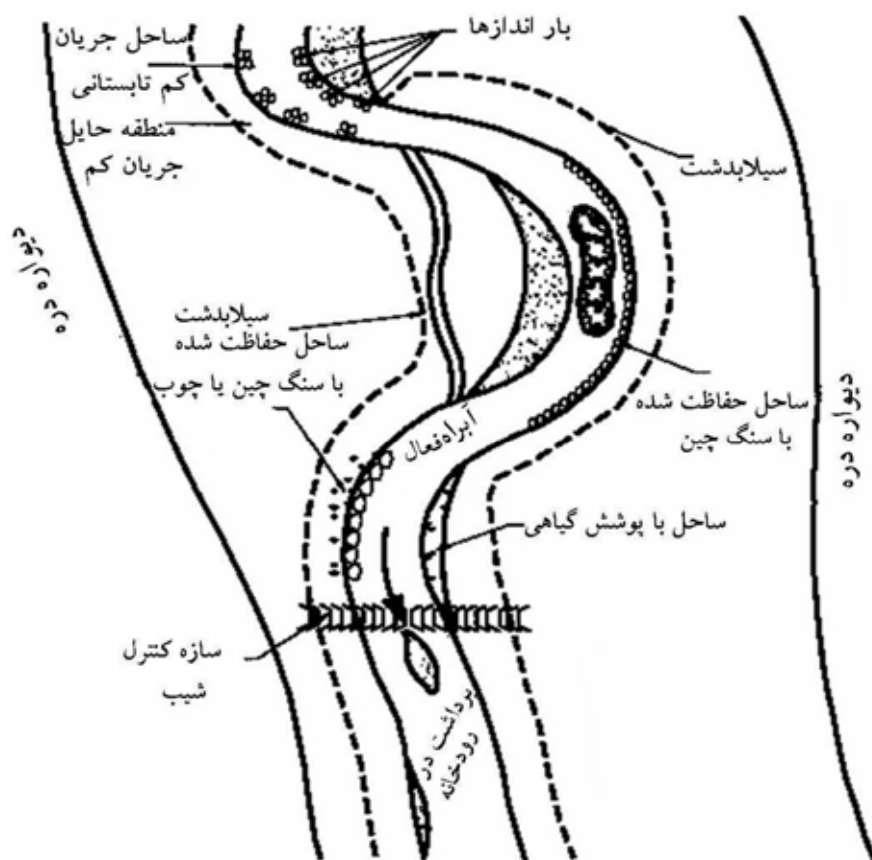
شکل ۴-۵- استفاده از سازه‌های محافظ
