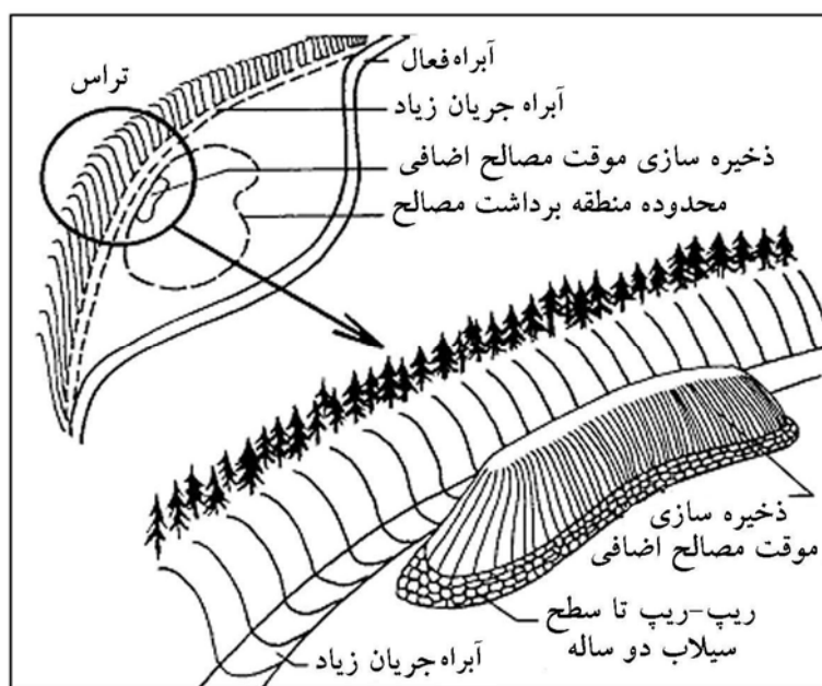
شکل ۷-۱۰-۵- تصویر نمونه از ذخیره‌سازی موقت مصالح اضافی (نشان‌دهنده شرایط مطلوب برای محل، شکل و محافظت)
