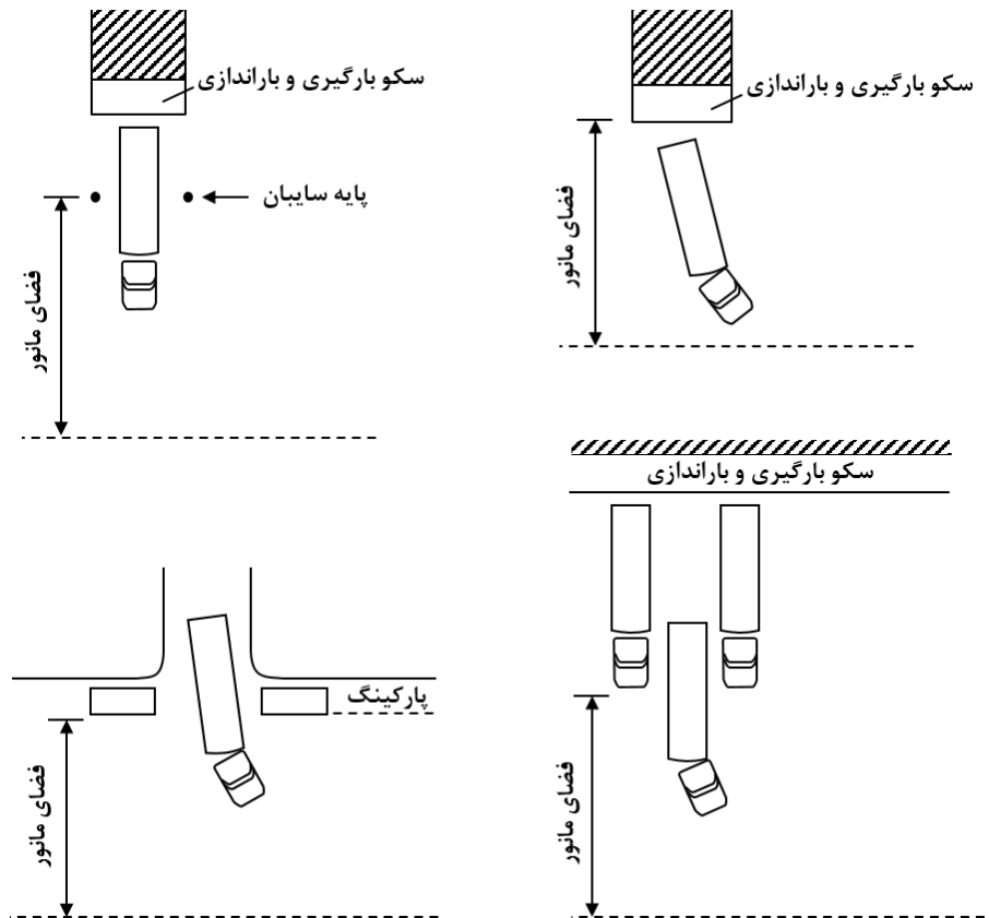
شکل ۵-۶- فضای مانور کامیون‌ها در حالت‌های مختلف تجهیزات بارگیری و باراندازی
