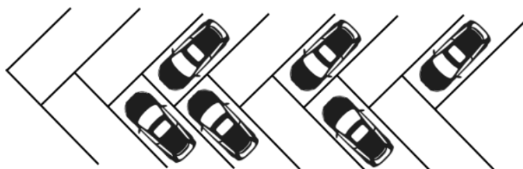
شکل ۵-۷- الگوی نامناسب برای طراحی فضاهای پارکینگ غیر حاشیه‌ای
