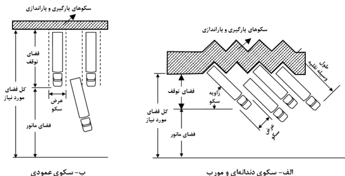
شکل ۶-۷- مشخصات هندسی و ابعاد انواع تجهیزات بارگیری و باراندازی
