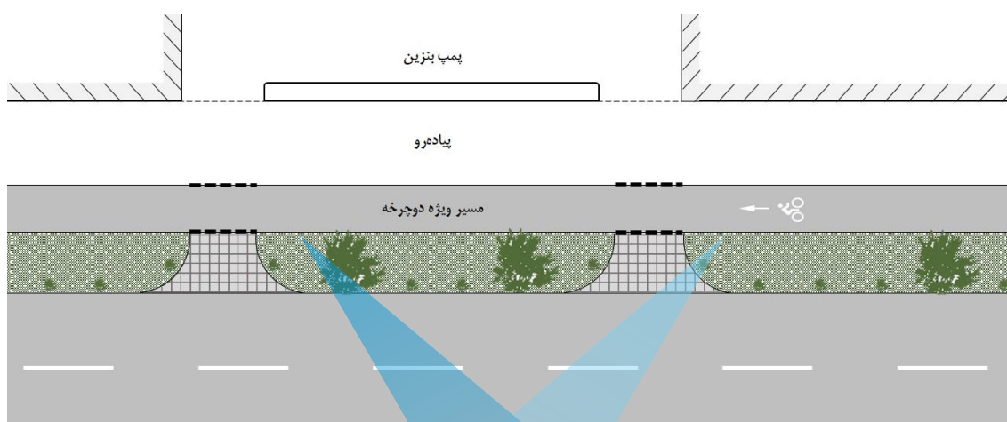
شکل ۴-۵- امتداد مسیر دوچرخه و پیاده‌رو در محل تلاقی راه دسترسی کاربری
