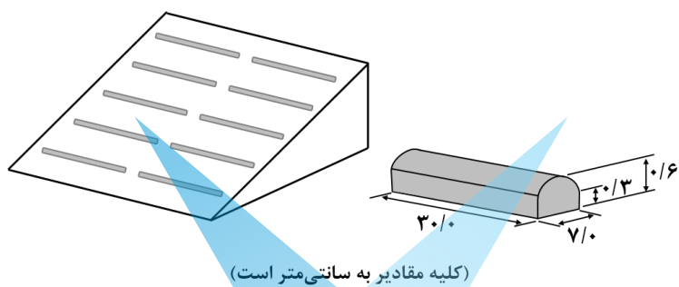
شکل ۵-۱۸- مشخصات هندسی ترمز شیراوه ویژه افراد دارای معلولیت
