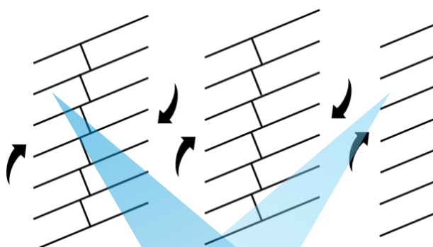
شکل ۵-۹- الگوی مناسب برای طراحی فضاهای پارکینگ غیر حاشیه‌ای زاویه‌دار با راهروهای دوطرفه
