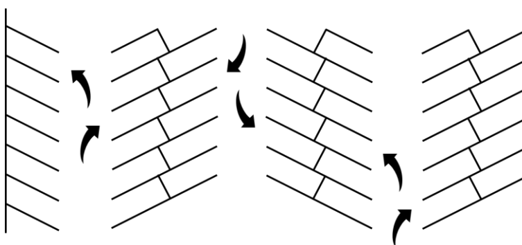
شکل ۵-۸- الگوی مناسب برای طراحی فضاهای پارکینگ غیر حاشیه‌ای زاویه‌دار با راهروهای یک‌طرفه
