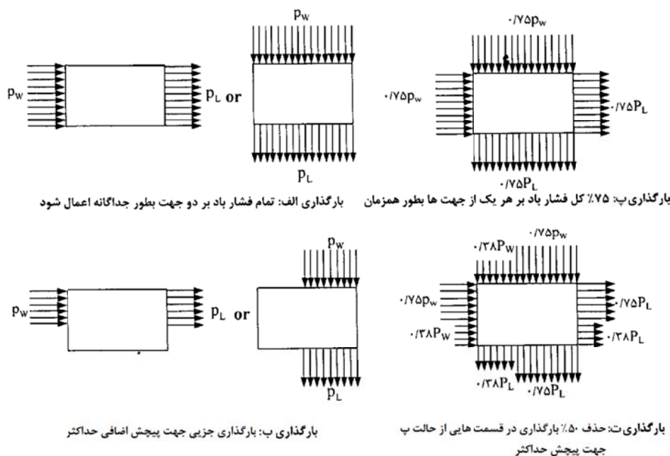
شکل ۶-۱۰-۸ بارگذاری باد کامل و جزئی
