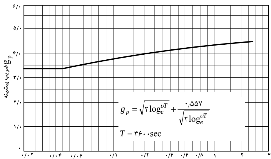
پ-۶-۲-۵ ضریب پیشینه بعنوان میانگین نرخ نوسانی
