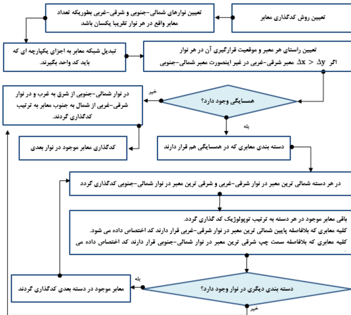
شکل (۳): روندنمای کدگذاری معابر بزرگراهی، شریانی (اصلی و فرعی) و جمع و پخش کننده
