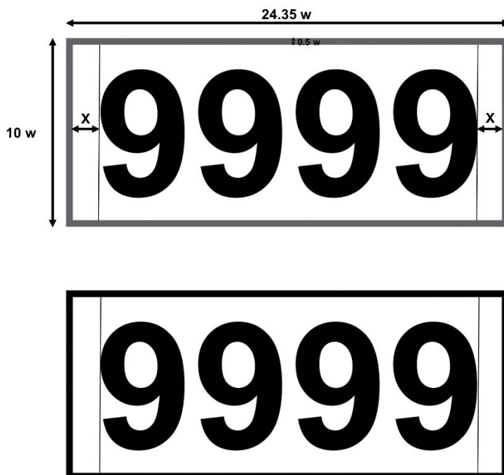
شکل (۱۱): جزئیات طراحی نماد (لوگو) کدگذاری معابر شریانی فرعی و جمع و پخش کننده (چهار کاراکتر)
