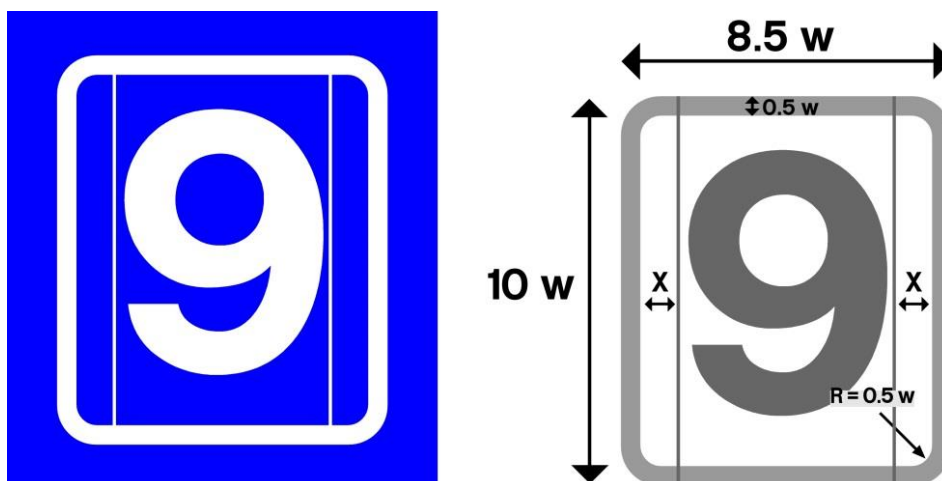
شکل (۱۲): جزئیات نماد (لوگو) کدگذاری معابر آزادراهی و برون‌شهری
