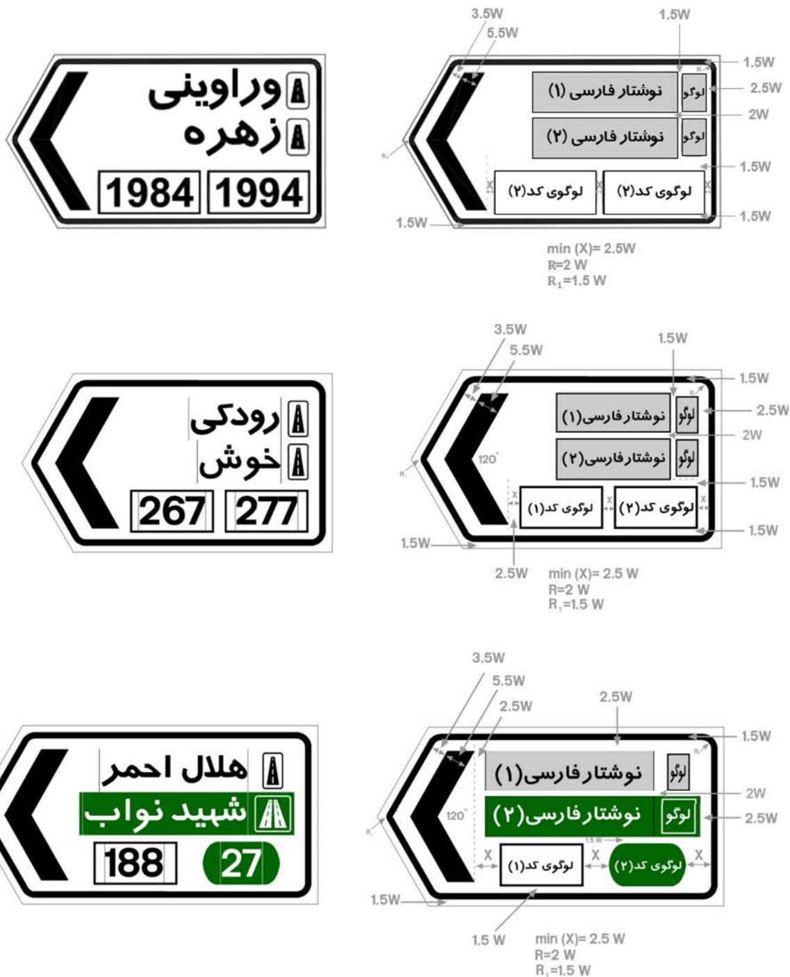
شکل (۱۴): نحوه چیدمان نوشتار و نماد (لوگو) کدگذاری در تابلوهای هدایت مسیر پرچمی جدید
