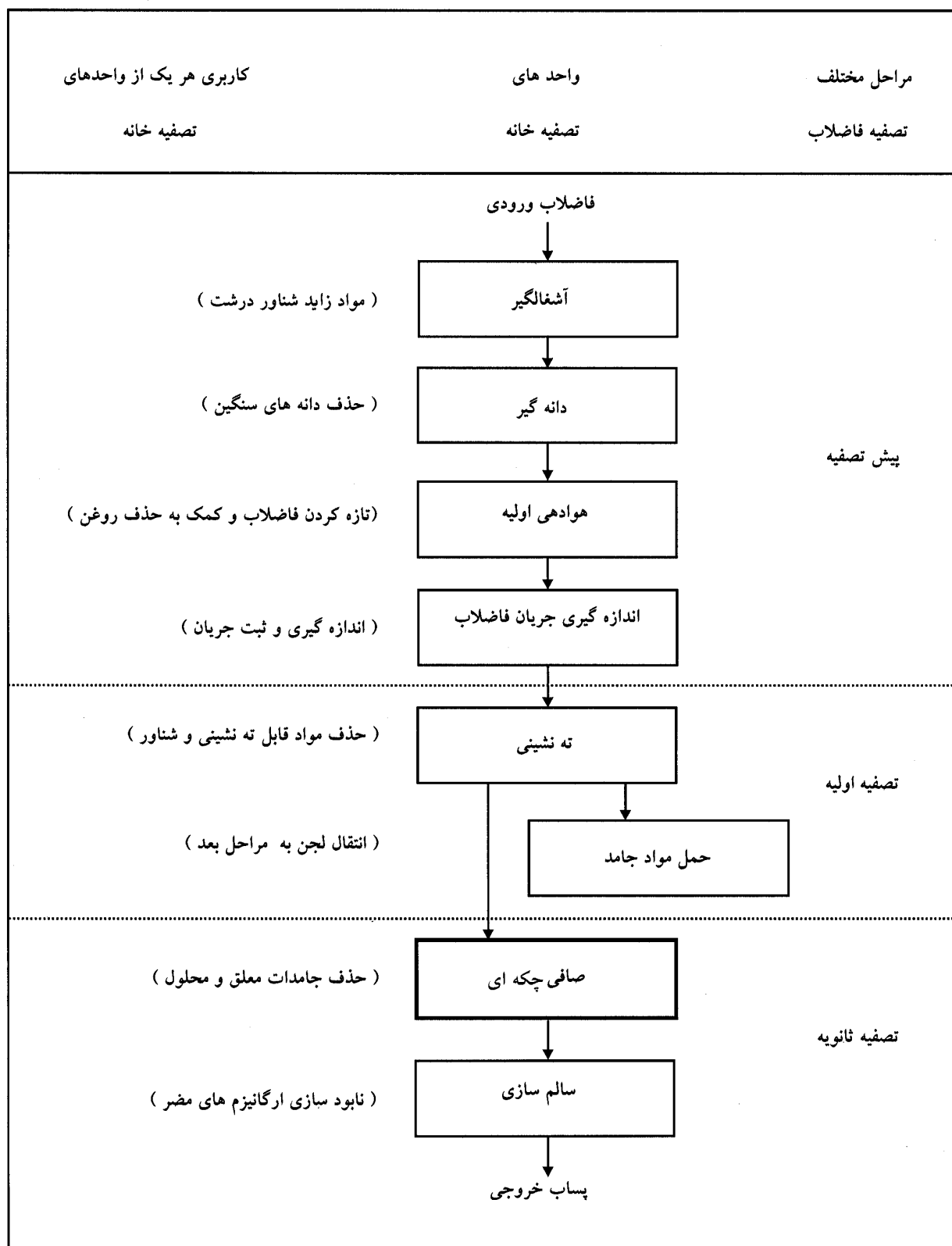
نمودار ۳-۱- موقعیت صافی چکه‌ای در تصفیه‌خانه فاضلاب
