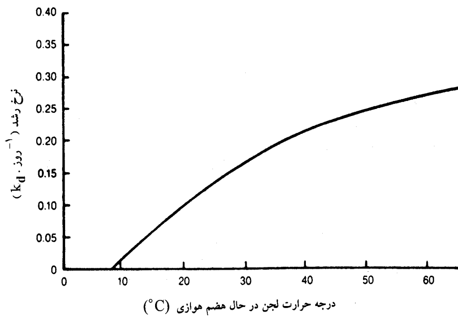
شکل ۴-۱۲ - تغییرات نرخ رشد لجن نسبت به درجه حرارت
