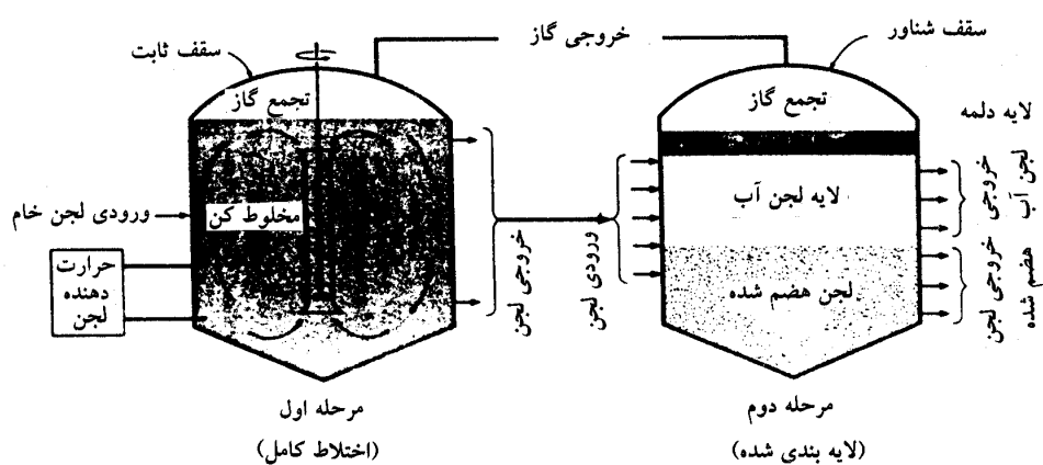
ب ( نمونه ای از یک هاضم سریع
