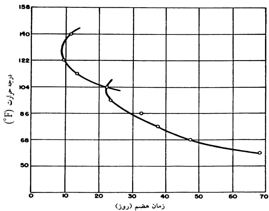
شکل ۴-۴ - رابطه مدت زمان هضم و درجه حرارت
