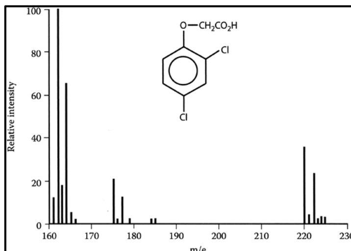
شکل ۹-۳- طیف‌سنجی جرمی قسمتی از علف کش ۲، ۴- دی کلرو فنوکسی استیک اسید (D-۲،۴)
