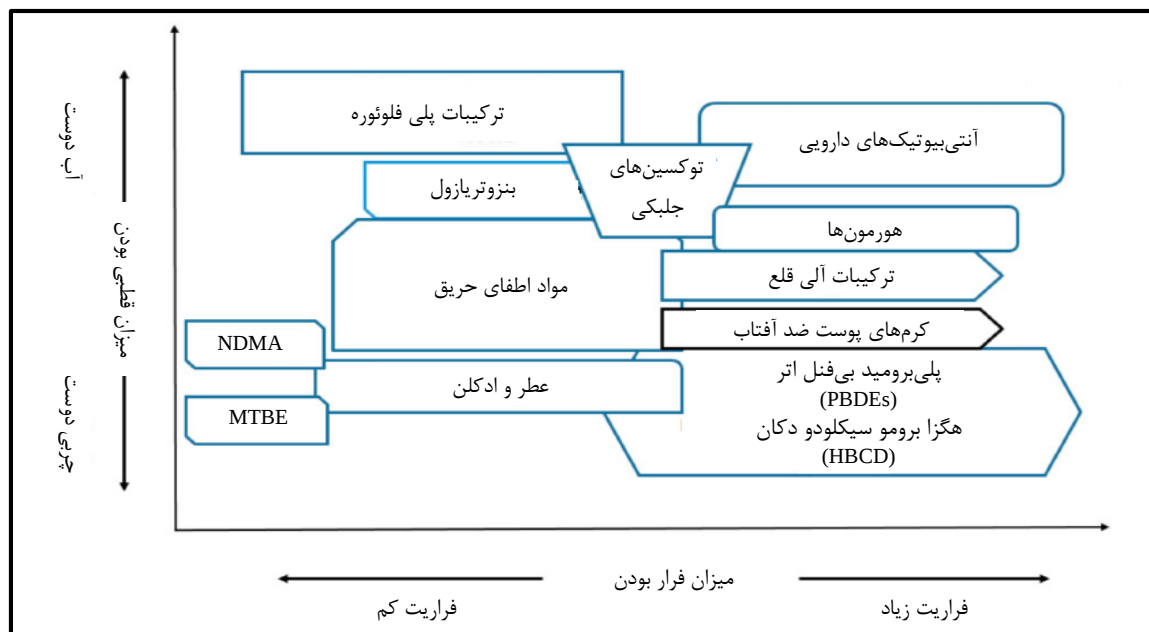
شکل ۴-۴- قطبیت و فراریت برخی آلاینده‌های نوظهور
