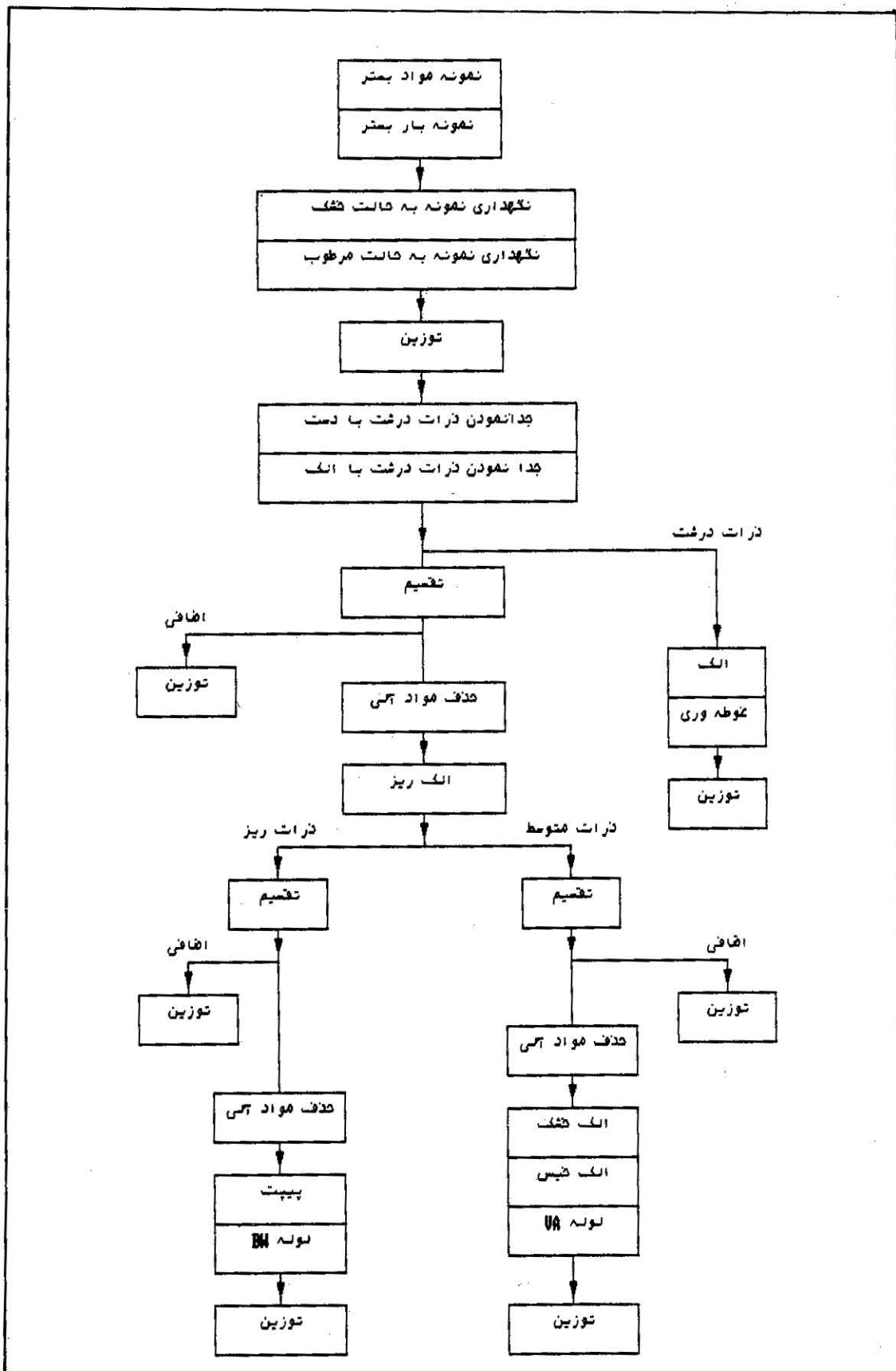
شکل ۱- روند نمای آزمایش کامل مواد کف و بار بستر
