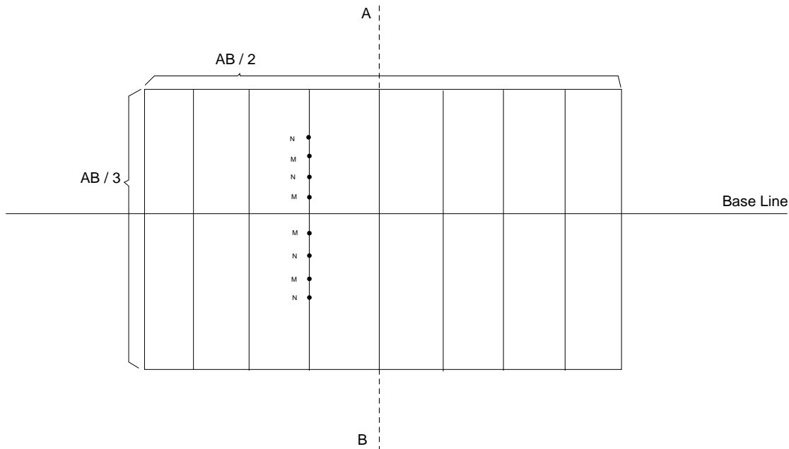
شکل ۲-۱. آرایش مستطیلی
