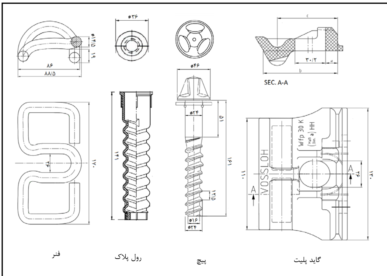
شکل ۵-۵- قطعات پایند نوع وسلو W30HH
