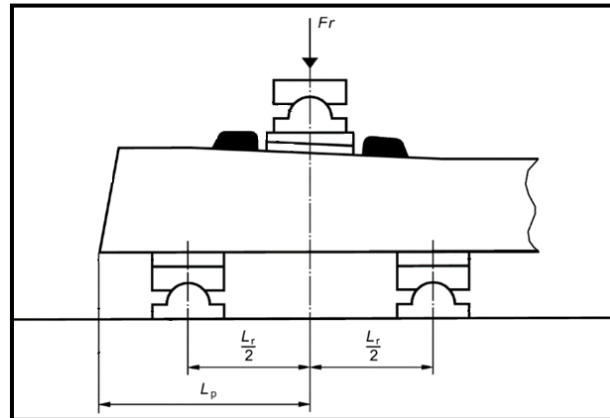
شکل ۴-۷- آزمایش لنگر خمشی مثبت محل نشیمن گاه ریل تراورس یک تکه
