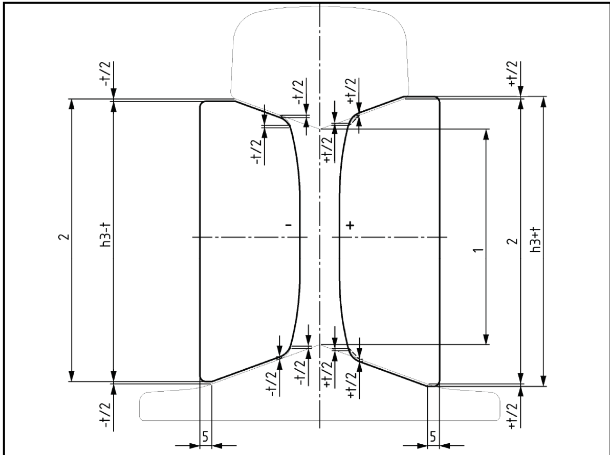
مقادیر ۱ و ۲ بایستی در فاصله ۱۴ میلی متری از لبه شابلون حک شده باشد. مقدار h3 اندازه تئوری است.
