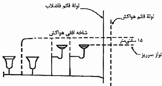
شکل ۱۶-۵-۲-۵ پ"ب" (۲) - اتصال هواکش به شاخه افقی لوله فاضلاب
